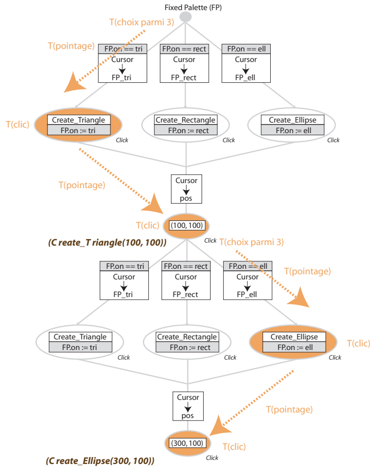
FIG. 3.7 : SimCIS : calcul des complexités
