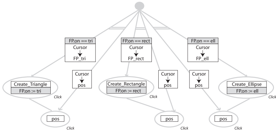
FIG. 3.34 : Un graphe d'interaction combinant parallélisme et persistance
