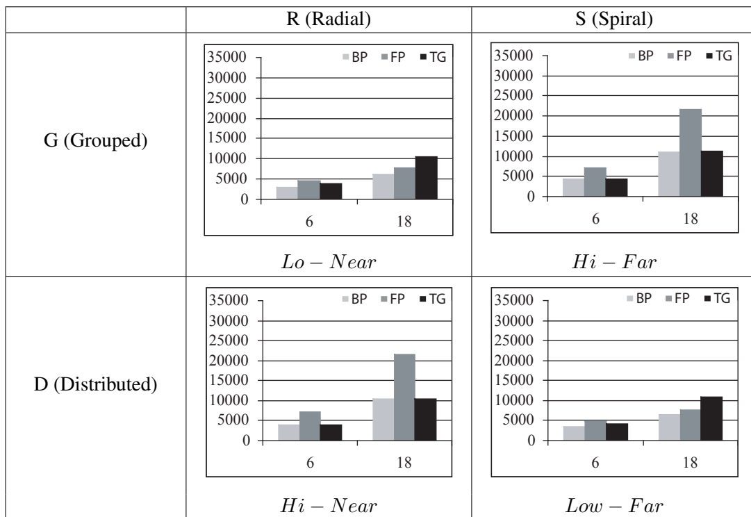
FIG. 4.3 : Les prédictions de SimCIS sur les tâches pour lesquelles l'ordre d'exécution est imposé
