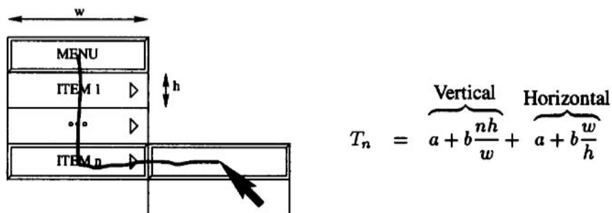
FIG. 3.2 : Suivi de chemin et sélection du n^{\text{e}} item dans un menu (Illustration extraite de [2])
