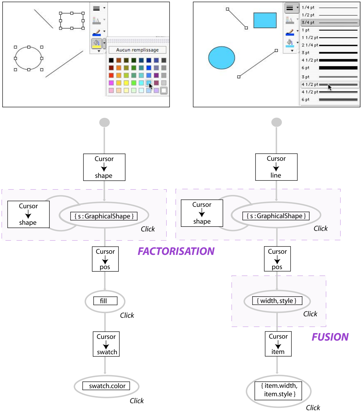
FIG. 2.17 : Propriétés de factorisation et de fusion. À gauche : appliquer la commande ( fill, s : GraphicalShape, c : Color ) à plusieurs objets de travail à la fois ; à droite : appliquer deux commandes ( width, s : GraphicalShape, w : Integer ) et ( style, s : GraphicalShape, s : Style ) à plusieurs objets de travail.
