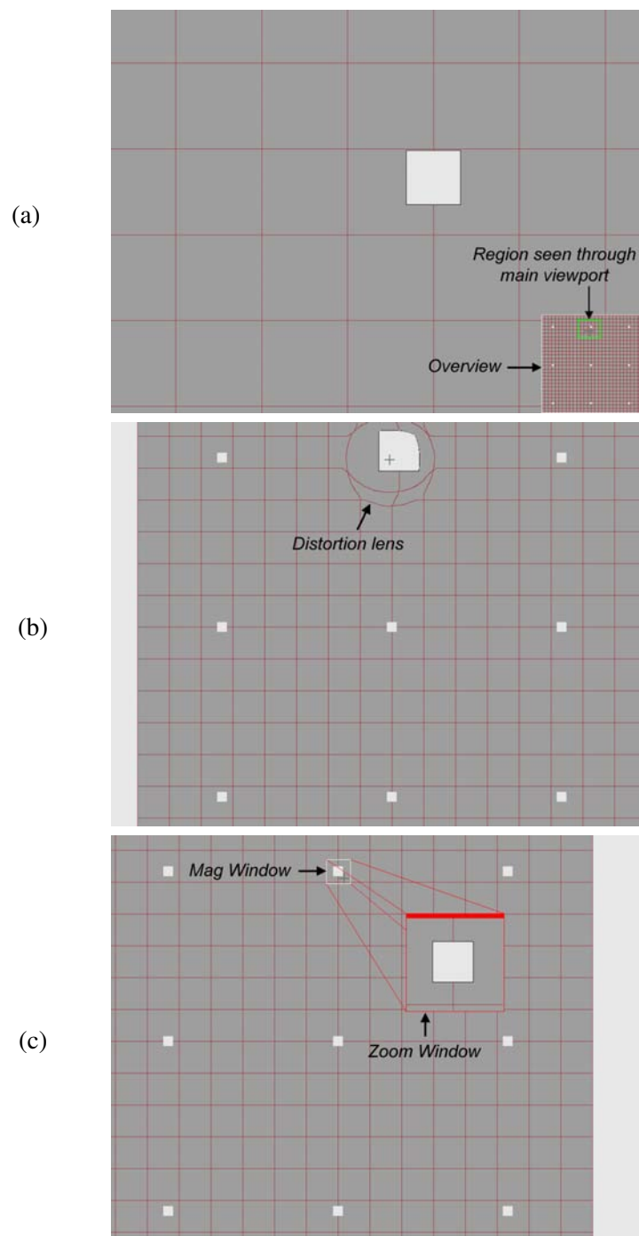
FIG. 4.16 : Dévoiler un objet avec (a) Pan & Zoom + Overview [OD] , (b) lentille de distortion [FL] , (c) DragMag [DM]
