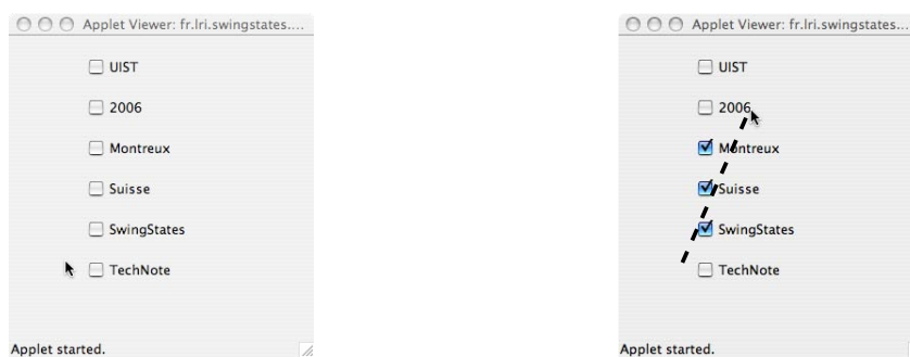
FIG. 5.13 : Des cases à cocher franchissables
