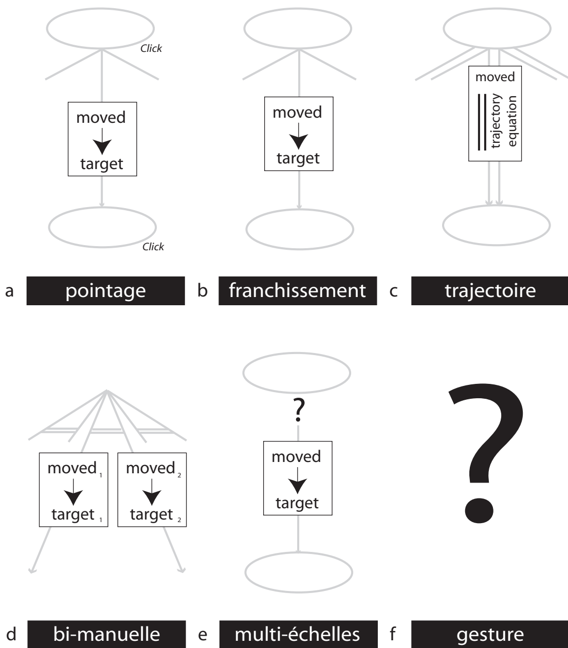
FIG. 4.12 : Les familles d'interaction et leurs profils CIS
