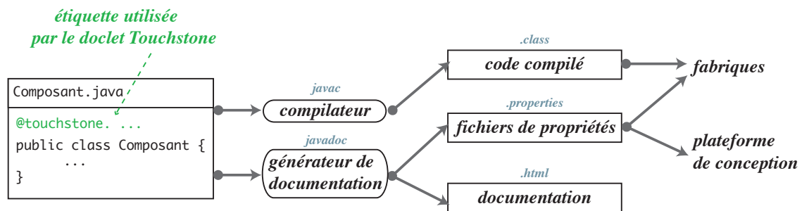
FIG. 6.14 : Mécanisme de fabriques et doclet de TouchStone
