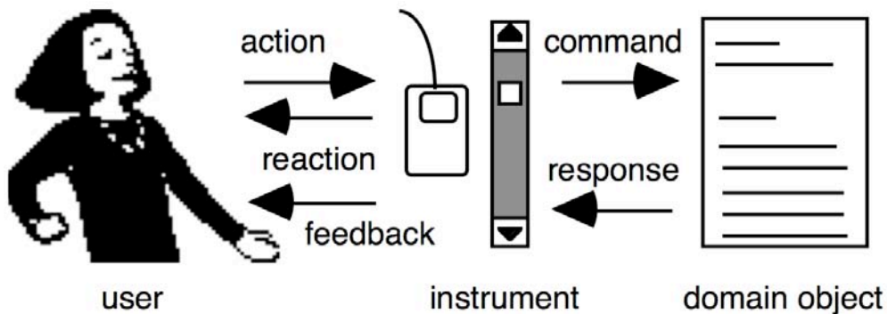
FIG. 2.6 : Le modèle de l'interaction instrumentale (Illustration extraite de [24])
