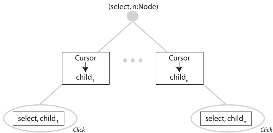
FIG. 3.22 : Structure CIS pour la sélection d'un nœud au niveau suivant avec une technique type "point-and-click"
