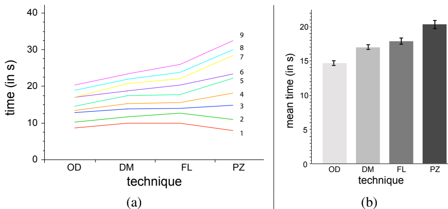
FIG. 4.19 : (a) Effet d'interaction rank * technique sur le temps de complétion (en s); (b) Temps de complétion moyen par technique (en s)
