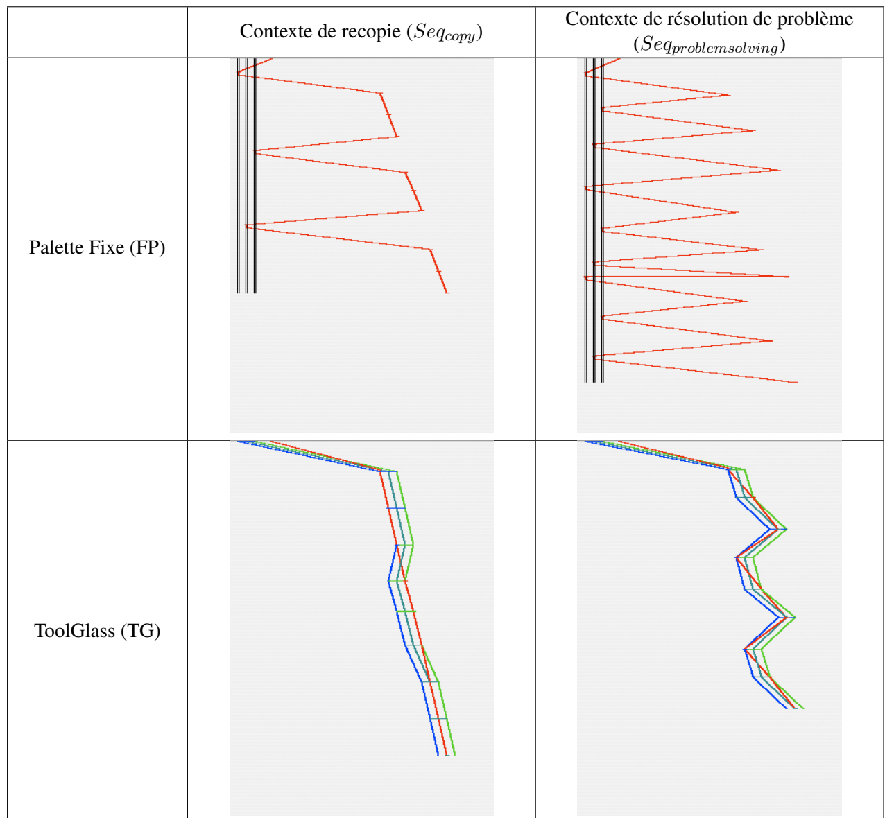
FIG. 3.9 : Exemples d'Object Movement Diagrams (OMDs)
