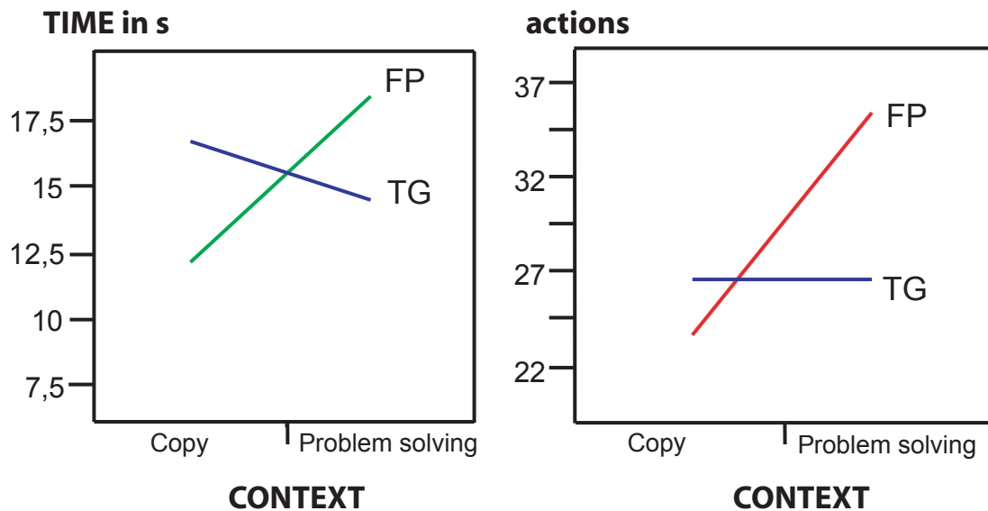
FIG. 3.8 : Complexités en temps (à gauche) et en actions (à droite) de la palette fixe et de la toolglass dans des contextes de copie et de résolution de problème
