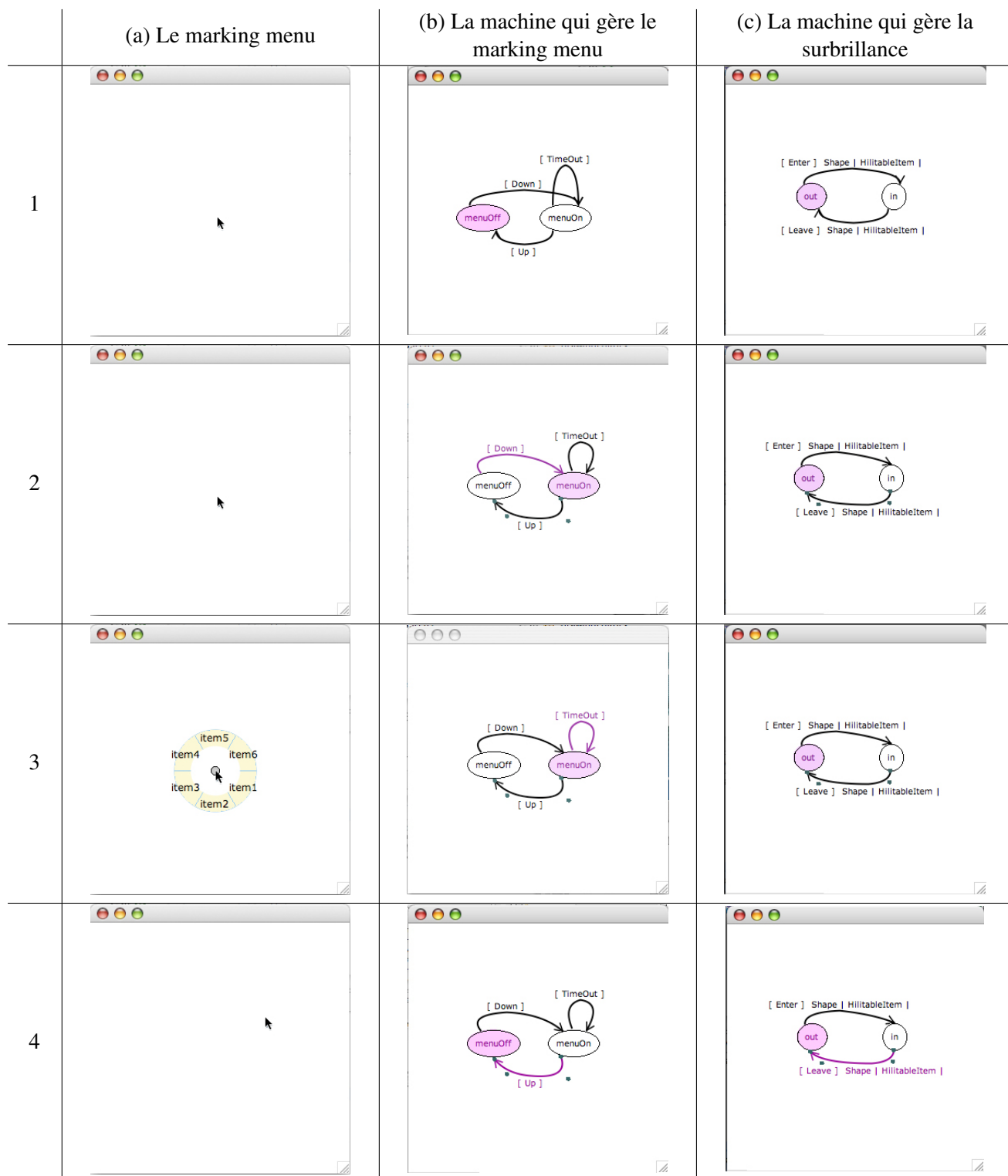
FIG. 5.11 : Visualiser les machines à états du marking menu
