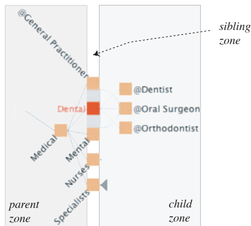
FIG. 3.22 : Structure CIS pour la sélection d'un nœud au niveau suivant avec une technique type "point-and-click"
