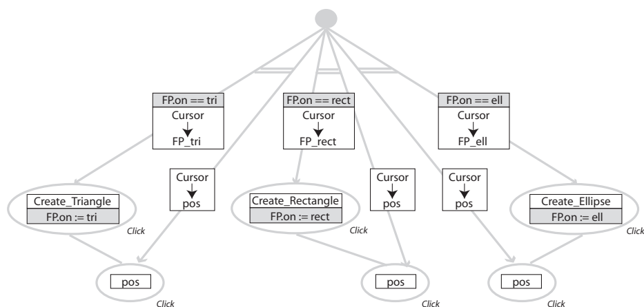
FIG. 3.34 : Un graphe d'interaction combinant parallélisme et persistance
