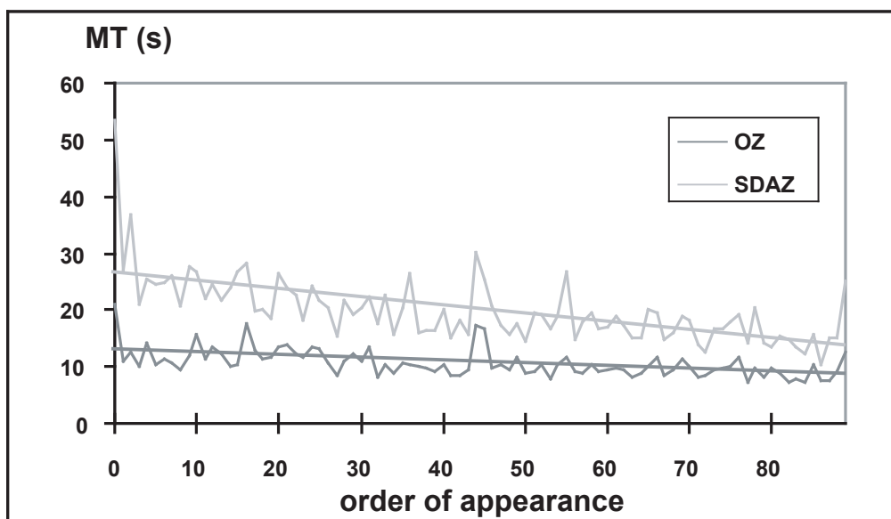
FIG. 3.19 : Apprentissage des deux techniques : temps moyen en fonction de l'ordre de présentation d'un essai
