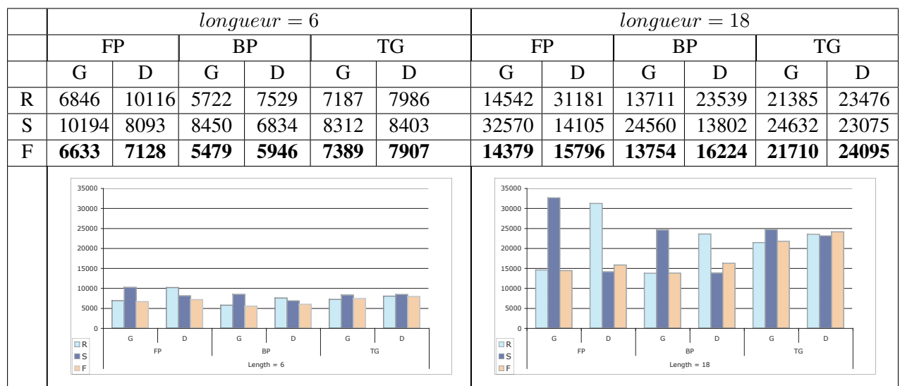
FIG. 4.8 : Séquences libres vs. séquences imposées : temps d'exécution moyen pour chacune des 36 conditions
