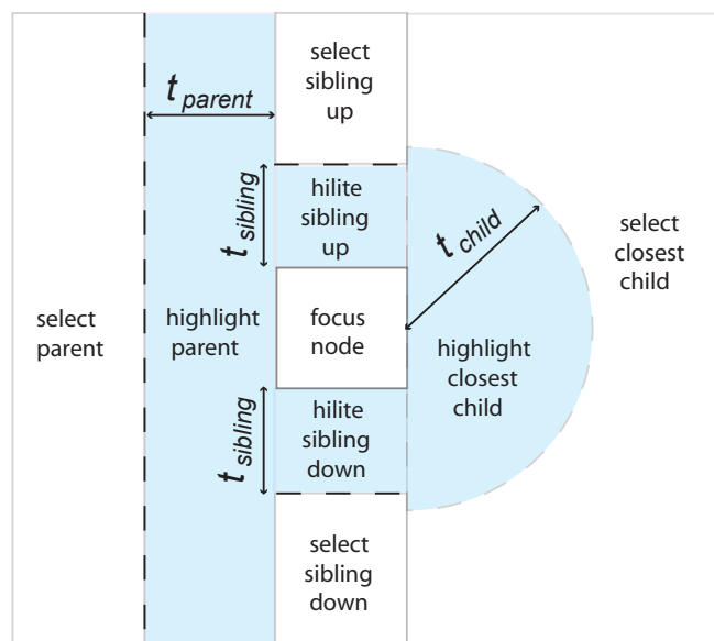
FIG. 3.25 : Zones d'interaction autour du nœud courant
