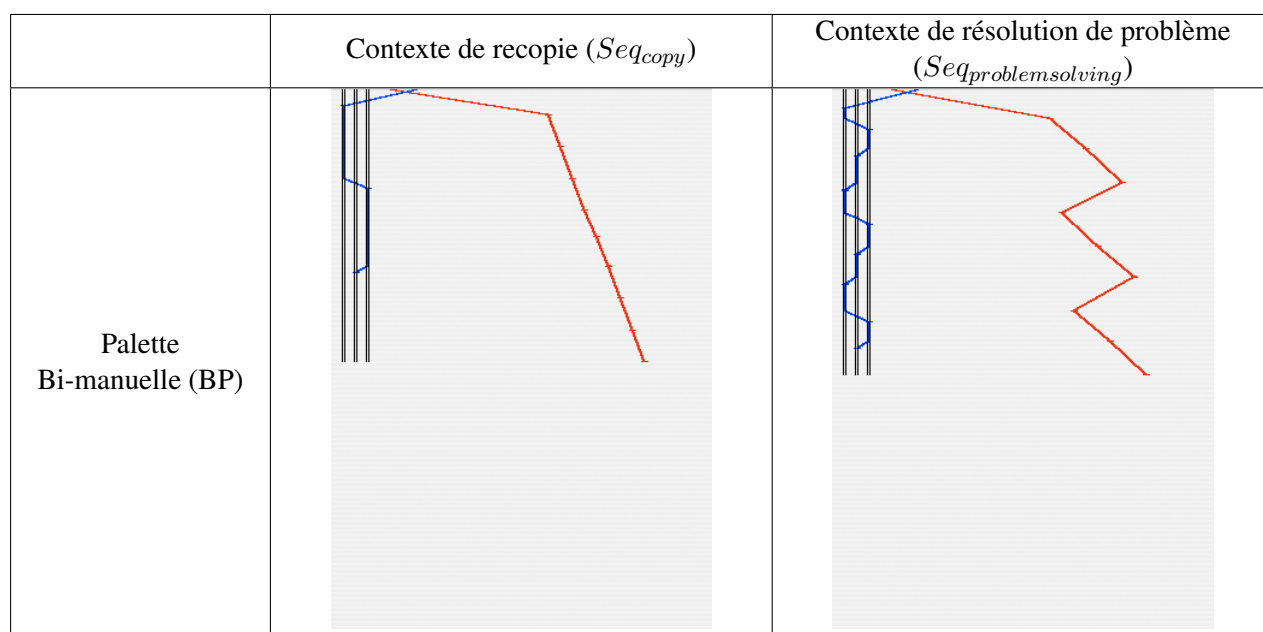
FIG. 3.37 : Object Movement Diagrams pour la palette bi-manuelle : à gauche, contexte de recopie ; à droite, contexte de résolution de problème
