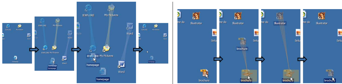
FIG. 3.11 : Diminuer D : à gauche, le drag-and-pop ; à droite, le drag-and-throw (Illustrations extraites de http://www.lirmm.fr/edel/dragging/ )
