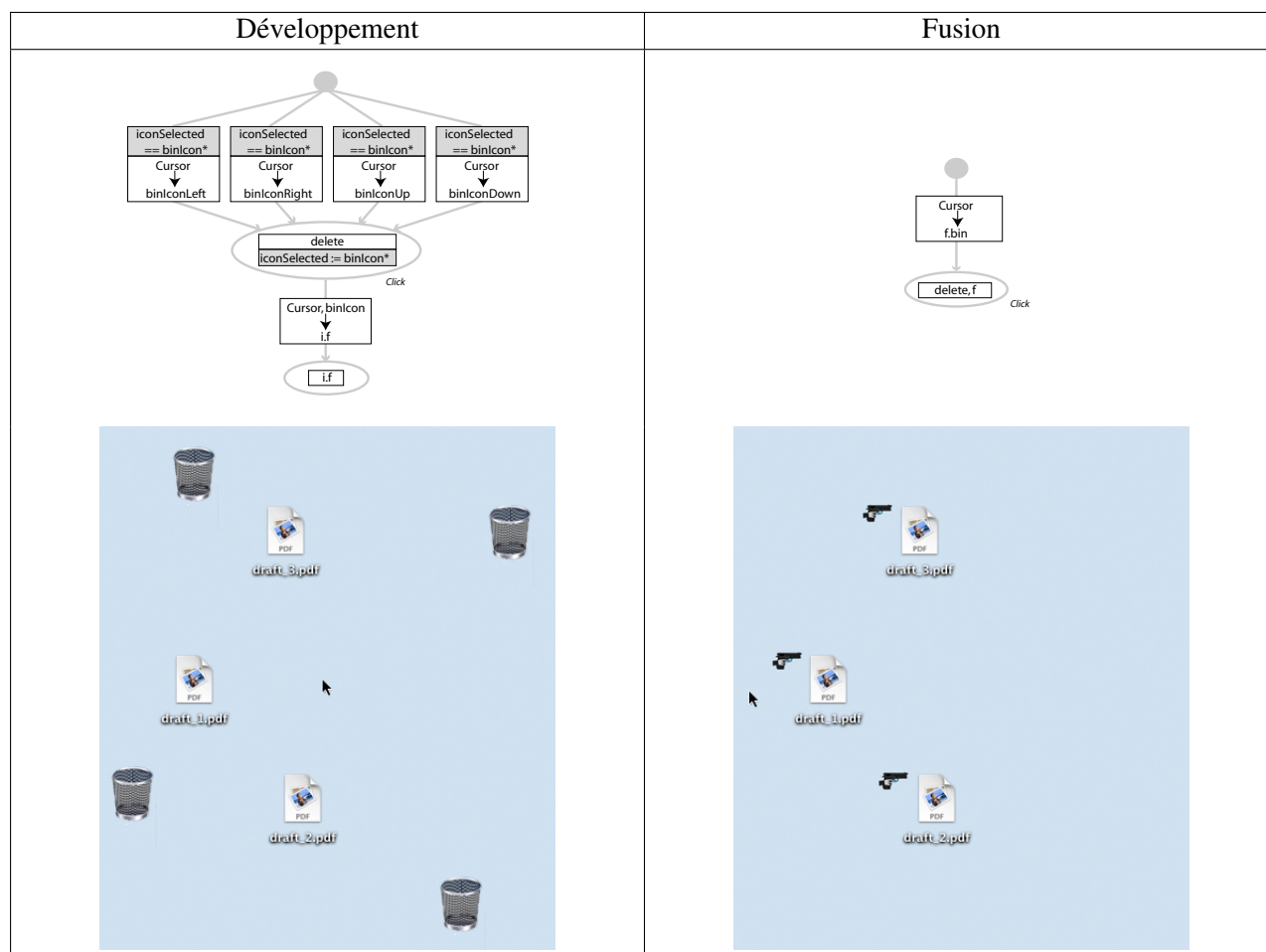
FIG. 3.33 : Développer ou fusionner
