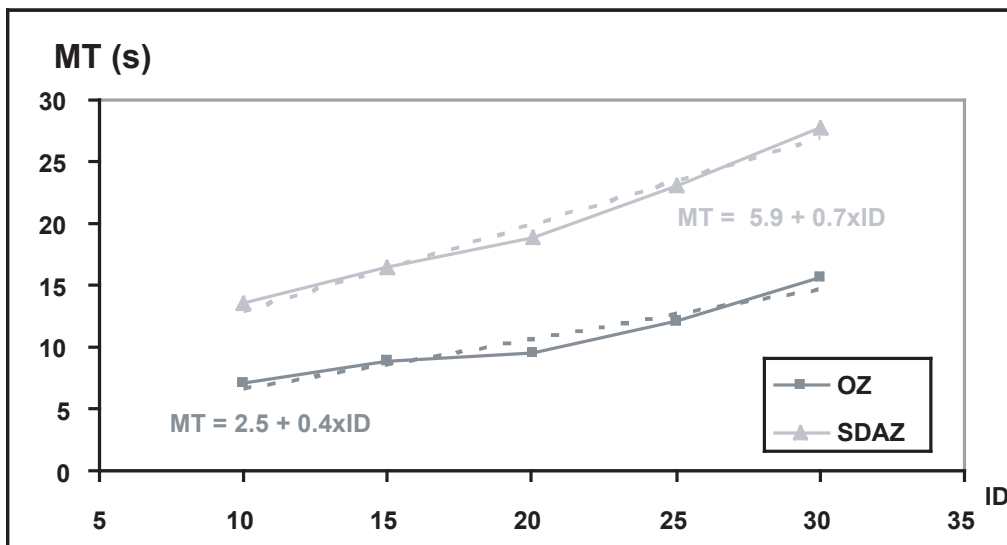
FIG. 3.18 : Analyse du temps de mouvement en fonction de l'indice de difficulté
