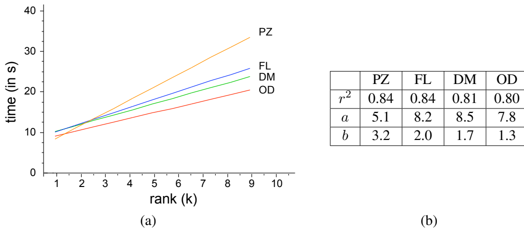
FIG. 4.18 : (a) Régression linéaire pour les quatre techniques; (b) Coefficients de corrélation ( r^2 ) et coefficients a et b ( time = a + b * rank ) pour les quatre techniques.
