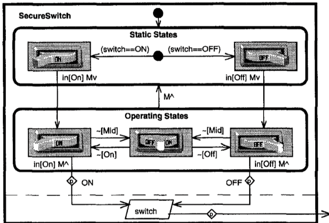
FIG. 2.4 : [IOG pour spécifier l'apparence et le comportement d'un interrupteur sécurisé] (Illustration extraite de [51])
