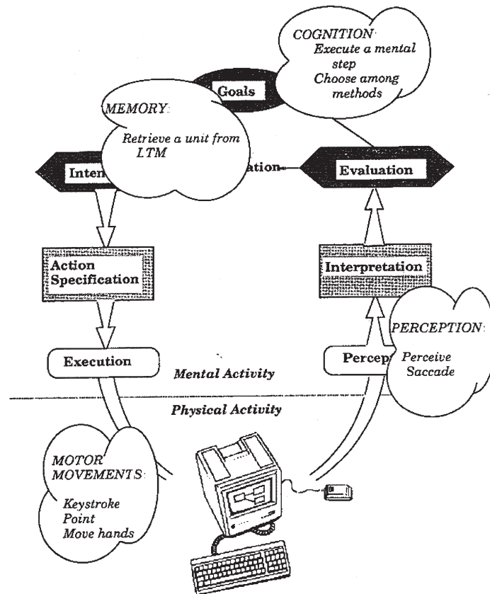
FIG. 2.8 : Les éléments modélisés par une architecture cognitive (Illustration extraite de [135])
