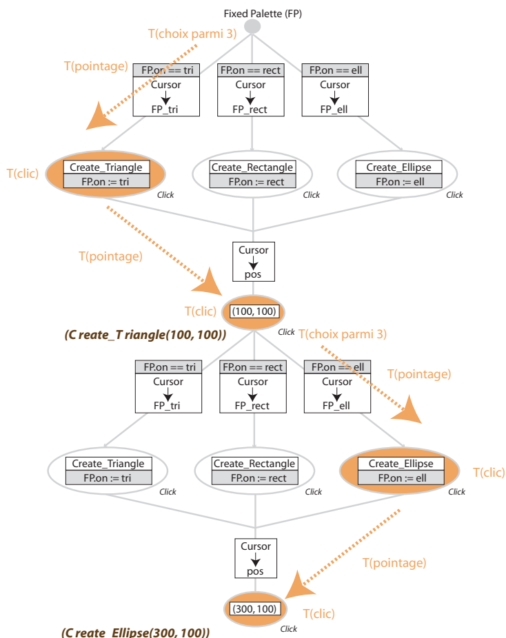
FIG. 3.7 : SimCIS : calcul des complexités
