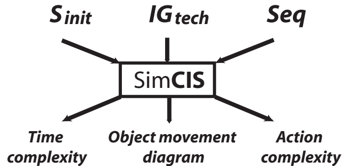
FIG. 3.6 : SimCIS : entrées et sorties
