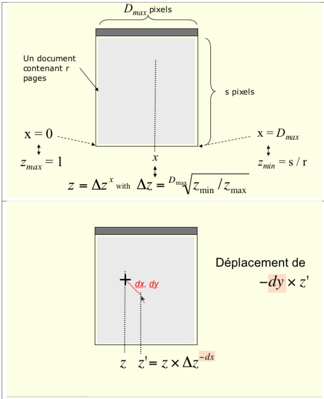
FIG. 3.13 : Utiliser la dimension orthogonale pour contrôler le facteur de zoom
