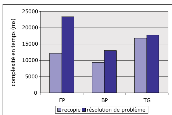
FIG. 3.36 : Complexité en temps de trois techniques dans deux contextes
