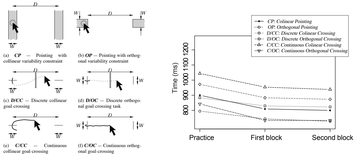
FIG. 3.3 : Pointage (P) VS. Franchissement (C) en fonction du type d'interaction (D : Discrète / C : Continue) et de la direction (O : Orthogonale / C : Colinéaire) (Illustration extraite de [4])
