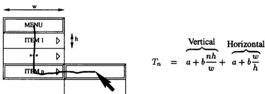
FIG. 3.2 : Suivi de chemin et sélection du n^e item dans un menu (Illustration extraite de [2])
