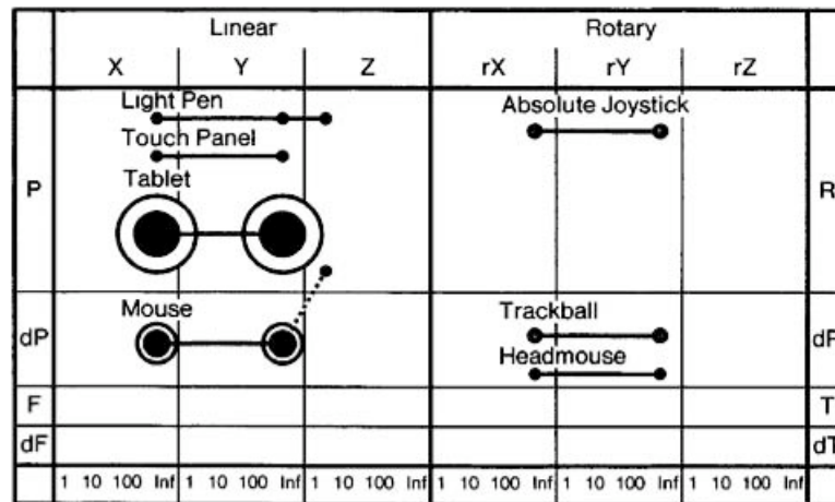
FIG. 2.1 : Représentation de l'espace de conception des périphériques de Card et al. (Illustration extraite de [47])
