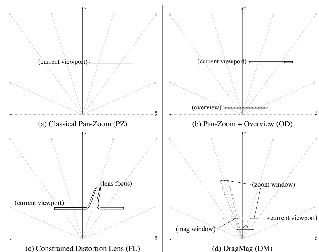
FIG. 4.13 : Représentation des techniques d'interaction multi-échelle dans des diagrammes espace-échelle. L'aire grisée représente la position de la seconde fenêtre de vue dans la vue courante.
