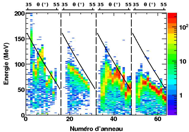
FIG. 3.9: Énergie dans les anneaux du détecteur E_{rés.} en fonction du numéro de l'anneau pour l'étalonnage avec la source 3\alpha . Les lignes continues représentent la valeur attendue pour les noyaux de ^{12}\text{C} diffusés élastiquement, tandis que les lignes verticales en pointillés marquent la limite des différents quartiers.
