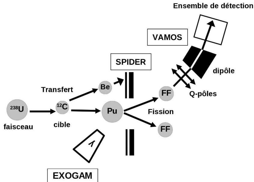
FIG. 2.10: Dispositif expérimental
