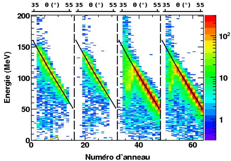
FIG. 3.12: Énergie dans les anneaux du détecteur E_{rés.} en fonction du numéro de l'anneau pour l'étalonnage avec la source 3\alpha et la diffusion élastique. Les lignes continues représentent la valeur attendue pour les noyaux de ^{12}\text{C} diffusés élastiquement, tandis que les lignes verticales en pointillés marquent la limite des différents quartiers.
