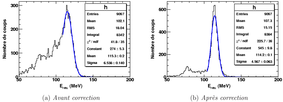
FIG. 3.19: Résolution en énergie résiduelle pour la cellule (anneau 38, secteur 9) du détecteur E_{rés.} pour la diffusion élastique du ^{12}\text{C} sur l'ensemble de l'expérience. La résolution avant correction est 13,33%, tandis qu'elle n'est plus que de 9,40% après. Les résultats des ajustements sont indiqués en encart.
