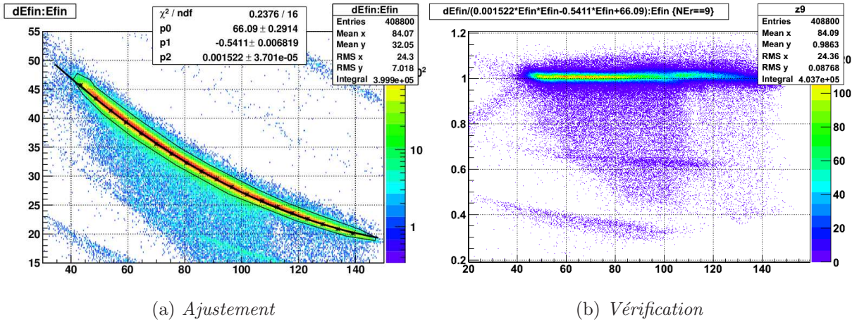
FIG. B.7: Ajustement avec un polynôme d'ordre 2 de la banane élastique de ^{12}\text{C} en \Delta E - E_{rés.} (a) et vérification de cet ajustement (b) pour les anneaux du secteur 9. Les paramètres de l'ajustement sont indiqués en encart.
