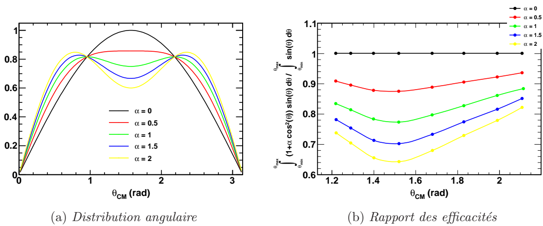
FIG. 4.24: Évolution de la distribution angulaire (a) et du rapport des efficacités (b) avec l'anisotropie
