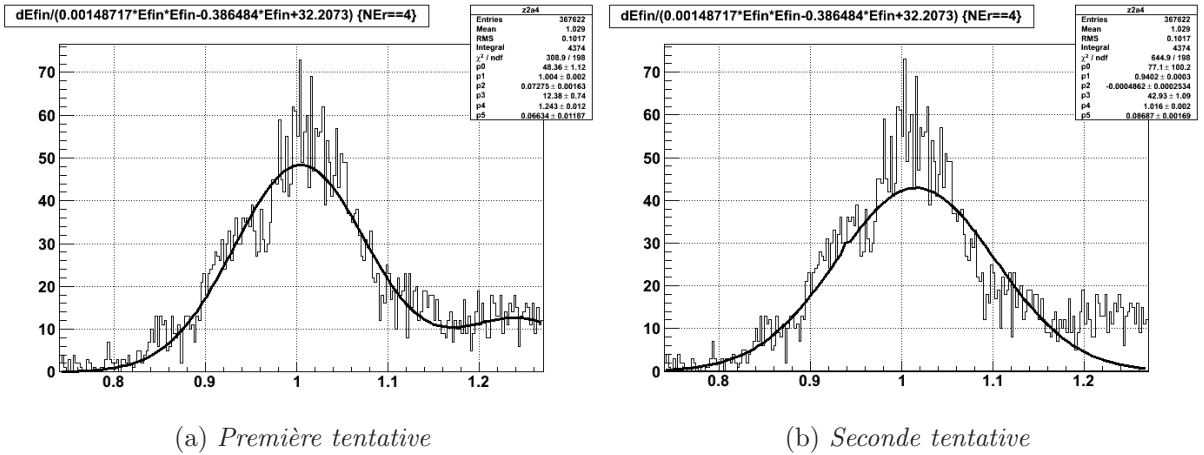
FIG. B.10: Tentatives d'ajustement à deux gaussiennes pour séparer les isotopes de Béryllium avec des paramètres initiaux différents. Les paramètres de l'ajustement sont indiqués en encart.
