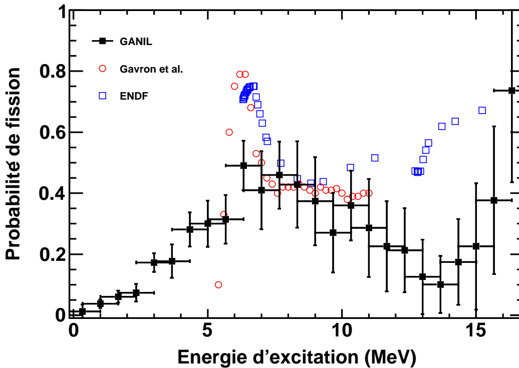
FIG. 4.33: Probabilité de fission du ^{239}\text{Np} obtenu lors de notre expérience (GANIL) comparée à celle obtenue par (^3\text{He},t,f) [Gavron 76] et aux données évaluées (ENDF/B-VII.0). B_f \simeq 5,8 \text{ MeV} et S_n \simeq 6,2 \text{ MeV} .
