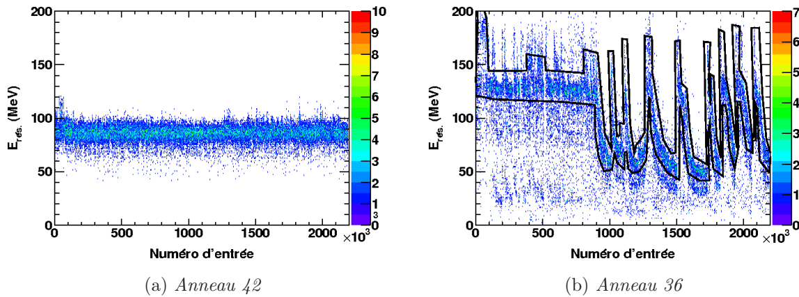
FIG. 4.14: Événements Carbone pour un anneau intermédiaire avec sélection en élément sur la matrice \Delta E - E_{rés.} (a) et pour un anneau interne avec une sélection dépendante du temps (b)
