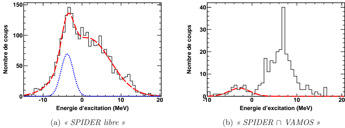
FIG. 4.32: Soustraction de la contamination par la voie Carbone des spectres en énergie d'excitation pour les déclencheurs « SPIDER libre » (a) et « SPIDER ∩ VAMOS » (b) pour B\rho_0 = 1,251 \text{ T.m}
