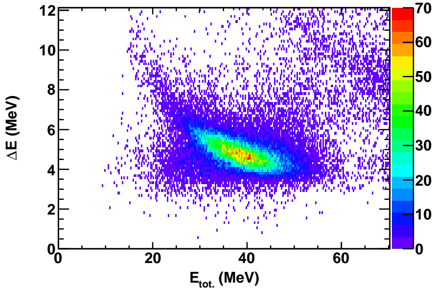
FIG. 4.5: Matrice d'identification pour la voie Hélium après étalonnage et corrections pour le déclencheur « SPIDER \cap VAMOS »
