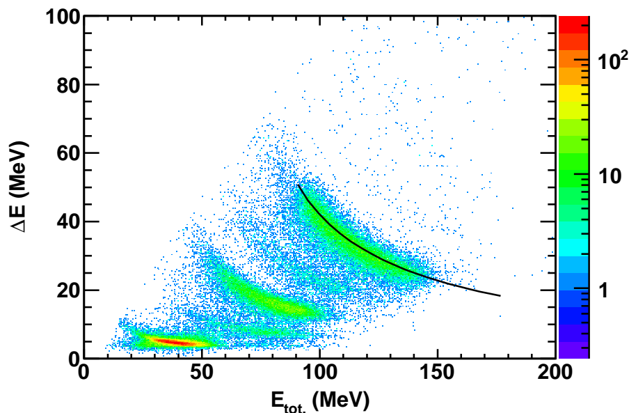
FIG. 4.4: Matrice d'identification après étalonnage, correction de l'évolution en temps et correction des effets liés à l'angle qui diffère pour les anneaux des deux détecteurs, pour le déclencheur « SPIDER \cap VAMOS ». La ligne continue représente la courbe attendue pour les noyaux de ^{12}\text{C} diffusés élastiquement.
