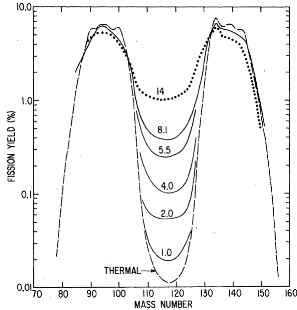
FIG. 2.6: Évolution de la distribution en masse des fragments de fission de l^{235}\text{U} en fonction de l'énergie incidente des neutrons qui l'induisent (cf. [Glendenin 81])
