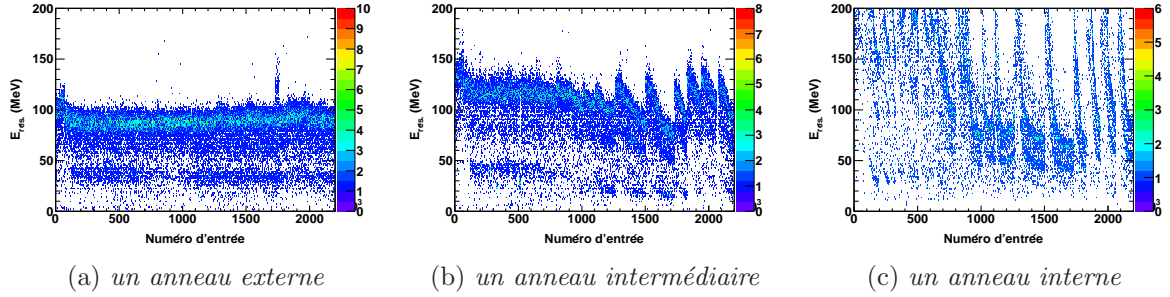
FIG. 3.14: Réponse en énergie pour différents anneaux du détecteur E_{rés} , en fonction du numéro d'événement (relié au temps)
