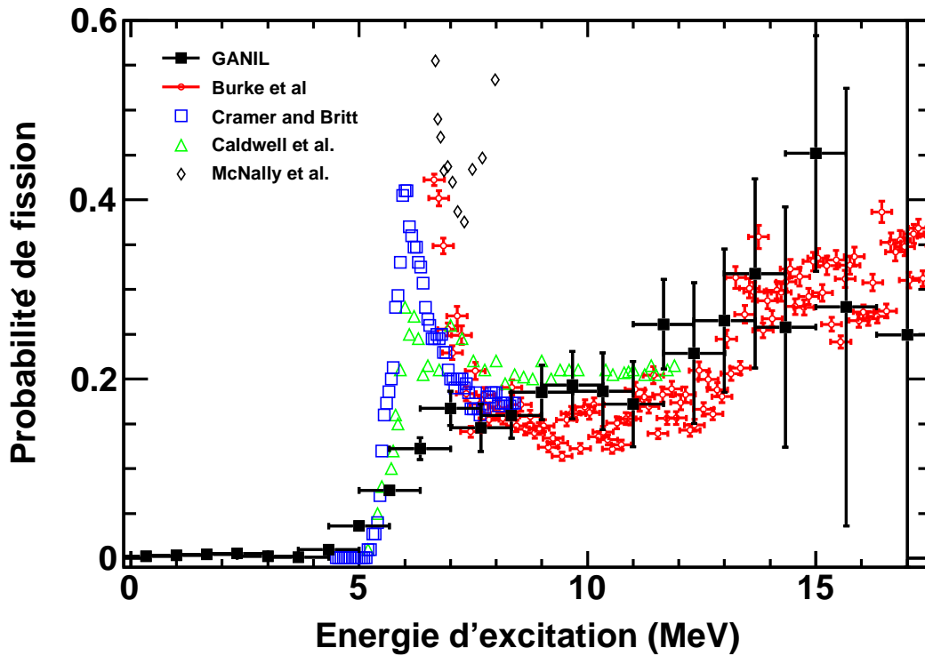
FIG. 4.29: Probabilité de fission de l^{238}\text{U} obtenu lors de notre expérience (GANIL) comparée aux résultats antérieurs : ^{238}\text{U}(\alpha, \alpha'f) [Burke 06], ^{238}\text{U}(\gamma, f) [Caldwell 80], ^{237}\text{U}(n, f) [McNally 74] et ^{236}\text{U}(t, pf) [Cramer 70]. B_f \simeq 5,9 \text{ MeV} et S_n \simeq 6,1 \text{ MeV} .
