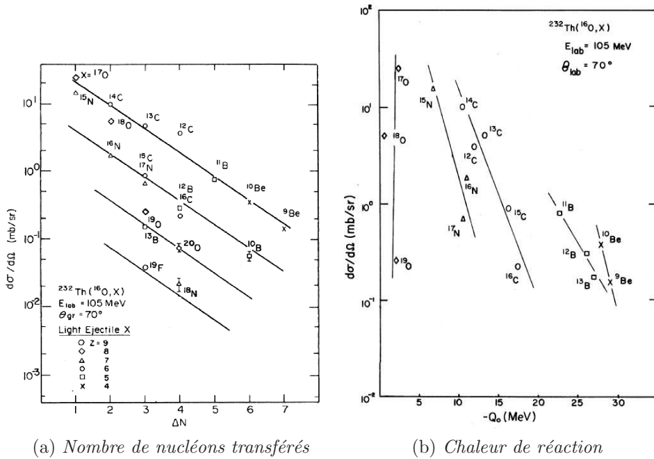
FIG. 2.4: Évolution de la section efficace de transfert en fonction du nombre de nucléons transférés (a) et de la chaleur de réaction (b) pour les voies de transfert ^{232}\text{Th}(^{16}\text{O}, X)
