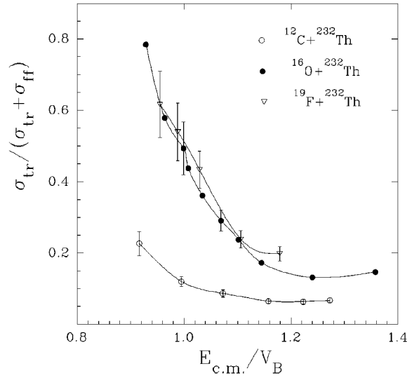
FIG. 2.3: Rapport des sections efficaces de transfert-fission et de fusion-fission en fonction du rapport de l'énergie dans le centre de masse sur la barrière coulombienne (cf. [Biswas 97])
