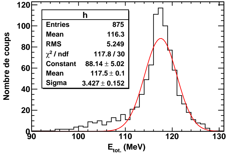
FIG. 4.7: Projection en énergie totale de la matrice d'identification \Delta E-E_{\text{tot}} pour la voie Carbone, un angle moyen de 47,8^\circ et une perte d'énergie comprise entre 32 et 33 MeV. Les paramètres de l'ajustement gaussien sont indiqués en encart.
