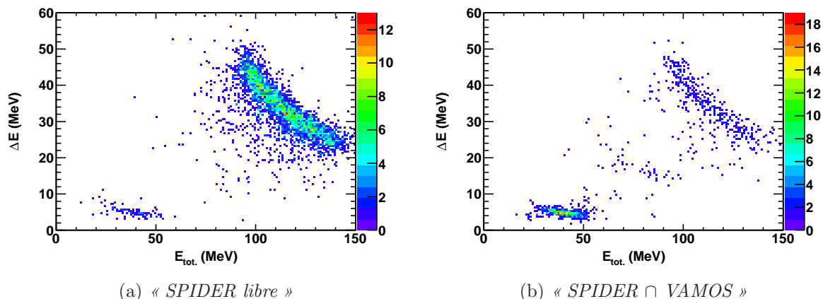
FIG. 4.6: Matrices d'identification \Delta E - E_{tot.} pour les événements ayant une multiplicité finale égale à deux pour les déclencheurs « SPIDER libre » (a) et « SPIDER \cap VAMOS » (b)
