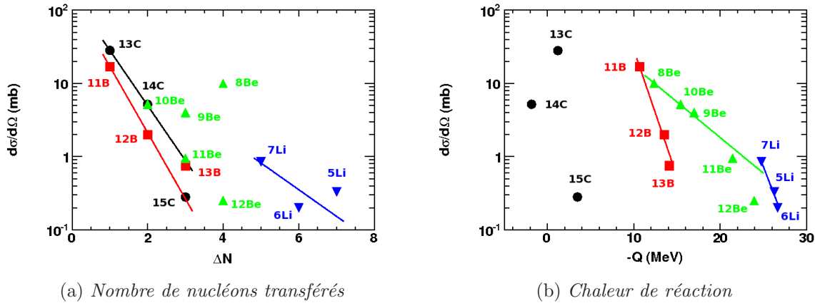
FIG. 2.5: Estimation de la section efficace de transfert en fonction du nombre de nucléons transférés (a) et de la chaleur de réaction (b) pour les voies de transfert ^{12}\text{C}(^{238}\text{U}, X) . Les lignes sont des ajustements exponentiels par chaîne isotopique.
