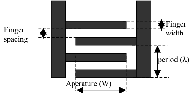
Figure 2.1 IDT parameters
