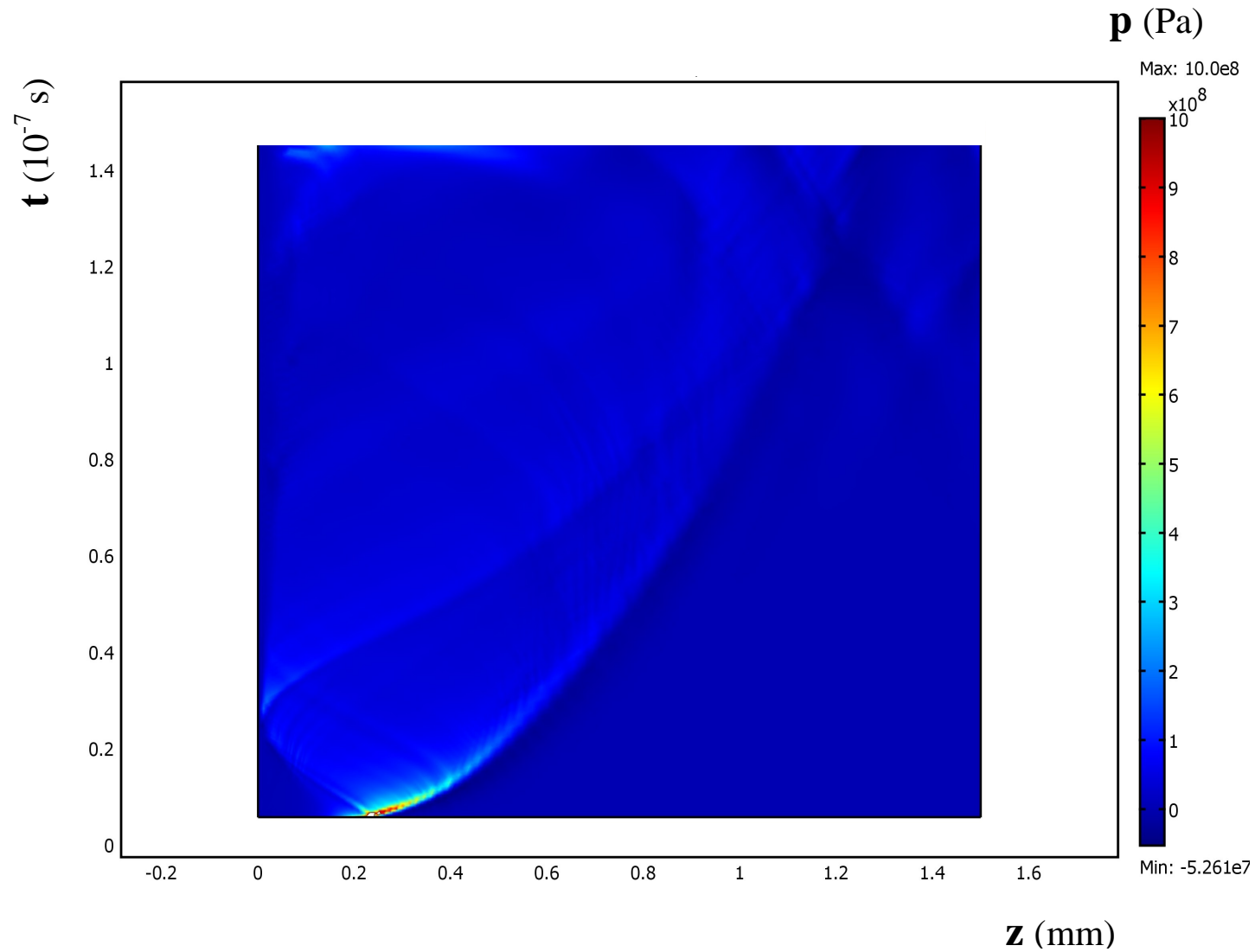
Fig. 7.23. Evolution temporelle de la distribution spatiale (le long de l'axe z ) de la pression du fluide « plasma + air » p .
