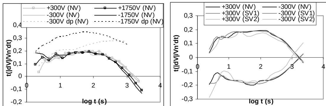
Figure 69 : Retour de potentiel normalisé au créneau de potentiel après déclin de 1800s
