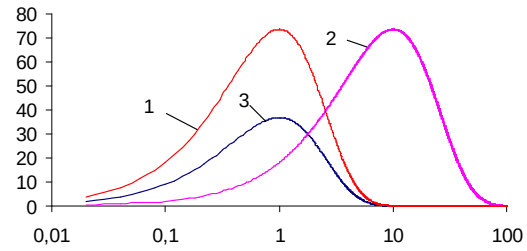
Figure 25 : Représentation d'exponentielles V_0 e^{-t/\tau} sous la forme t dV/dt = f(\log t)
