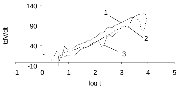
Figure 52 : Réponse de base du polypropylène
