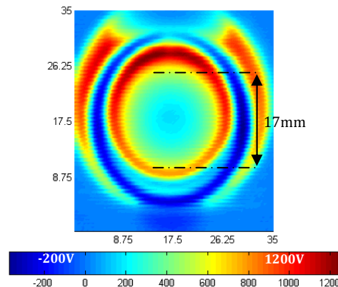
Figure 58 : Cartographie de potentiel sur PET Dépôts de charge positifs et négatifs successifs
