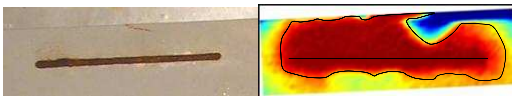
Figure 64 : Photographie et cartographie de potentiel au voisinage d'une blessure
