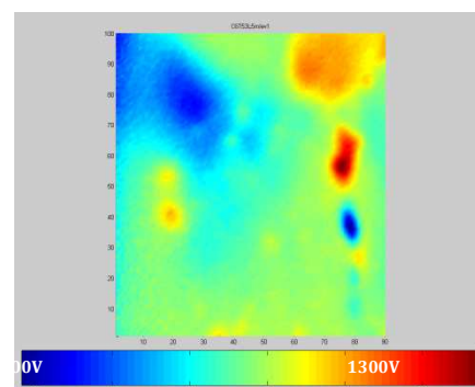
Figure 62 : Cartographie (100x100mm) de potentiel après décollement, rotation et repositionnement d'une plaque initialement neutre
