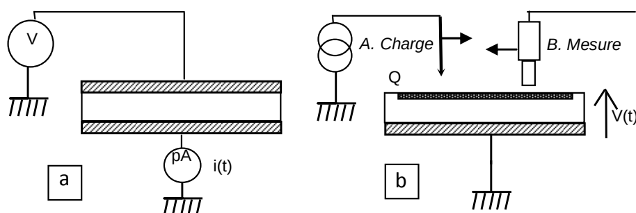
Figure 2 : Mesures électrostatiques
