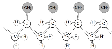
Figure 51 : Polypropylène isotactique
