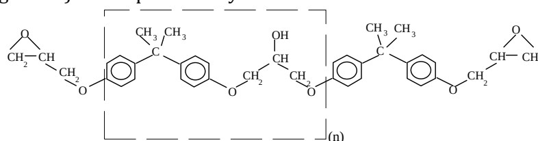
Figure 40 : Formule de la résine époxy DGEBA
