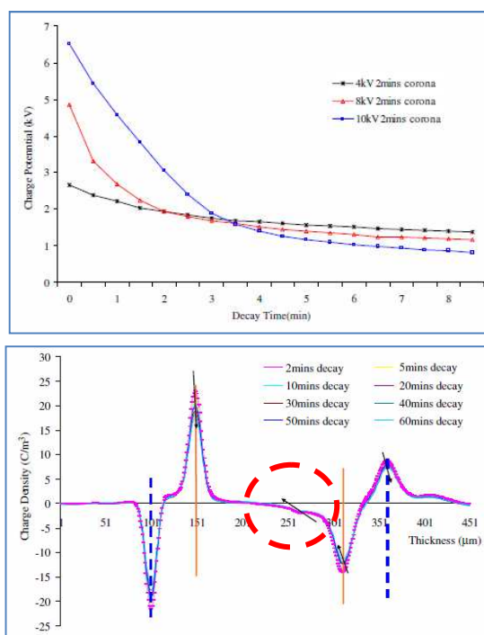
Figure 74 : Déclin de potentiel et mesures PEA [77]
