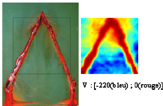
Figure 63 : Photographie et cartographie de V Revêtement anticorrosion blessé et vieilli au brouillard salin Cartographie 40x40mm
