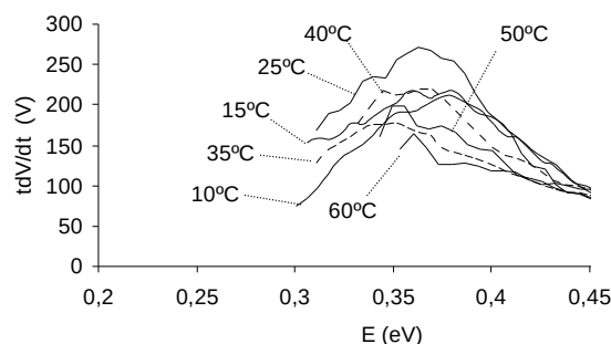
Figure 54 : Application du modèle de l'énergie de démarcation au « pic A »
