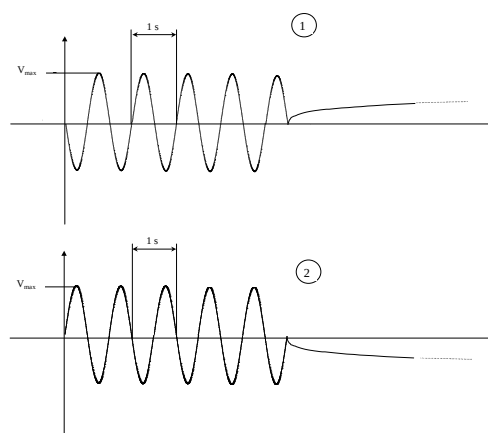
Figure 36 : Retour de potentiel après application d'une polarisation sinusoïdale
