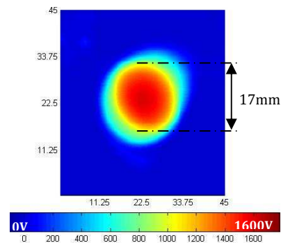
Figure 57 : Cartographie de potentiel sur PET Charge corona 20 \mu\text{A} +2000V, 21h après charge
