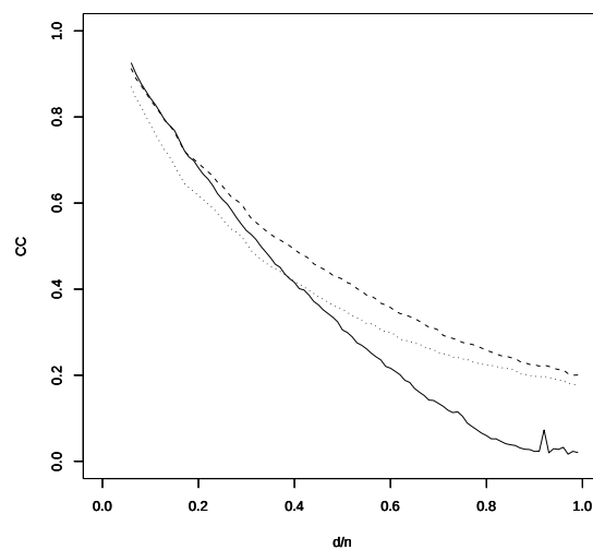
FIG. 3.5 – Critère CC en fonction de la dimension d de la variable X pour les méthodes SIR (trait continu), Ridge (tirets) et Tikhonov (pointillés). En abscisse, le rapport d/n et en ordonnée le critère CC.
