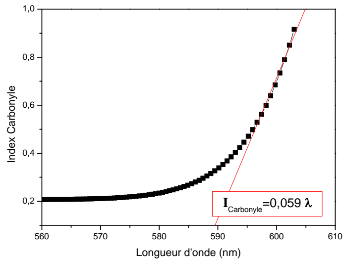
Figure IV- 12 : Corrélation entre la quantité de produit de dégradation carbonyle présente dans le matériau et la longueur d'onde d'émission de la sonde fluorescente.
