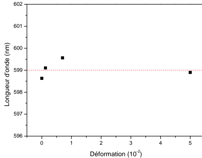
Figure V-12 : Evolution de la position du pic de fluorescence en fonction de la déformation totale appliquée.
