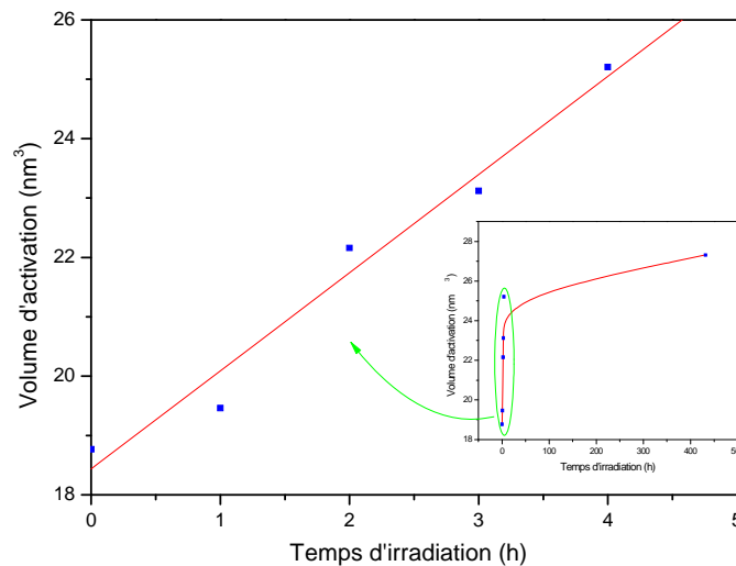
Figure IV- 32 : Evolution du volume d'activation viscoplastique sur des échantillons contraints à 2,75 MPa en fonction de la durée d'irradiation UV à 254 nm.
