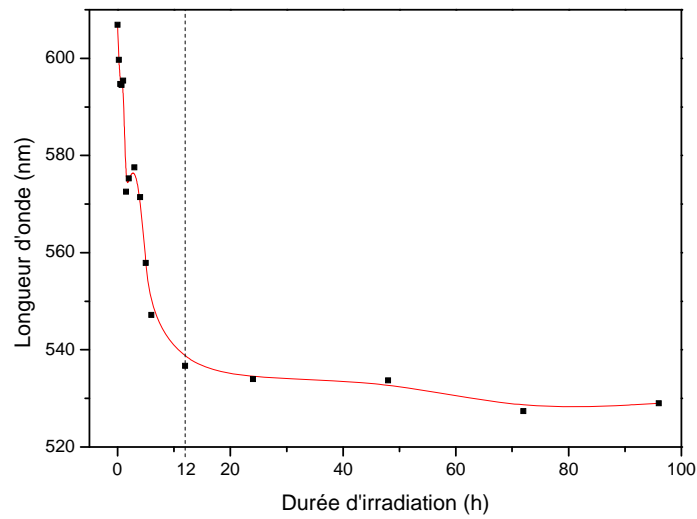
Figure IV- 5 : Evolution de la longueur d'onde du signal fluorescent émis au cours de l'irradiation UV.
