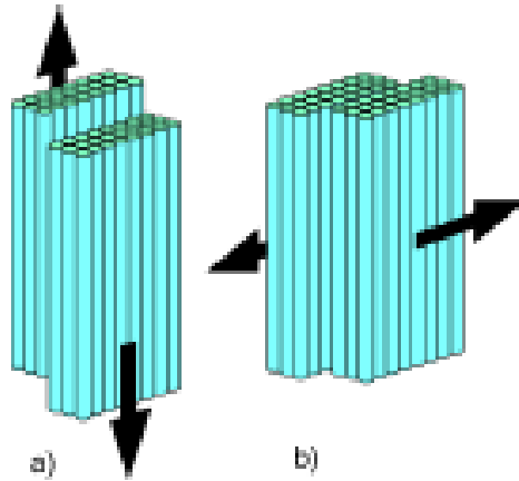
Figure I-19 : Glissement parallèle aux chaînes (a) ou perpendiculaire aux chaînes (b).
