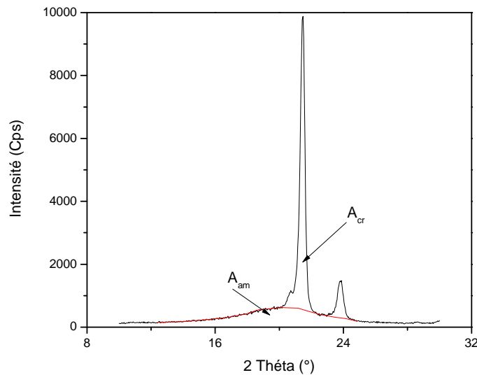
Figure III-9 : Diffractogramme élargi du PEHD pour calculer le taux de cristallinité.
