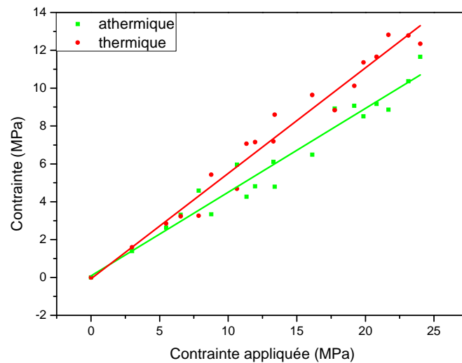
Figure V-21 : Evolution des contraintes thermique et athermique en fonction de la contrainte appliquée.
