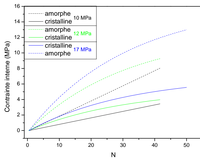
Figure V-35 : Evolution des contraintes internes dans les phases amorphe et cristalline en fonction du nombre de cycle N pour différentes valeurs de contraintes appliquées.
