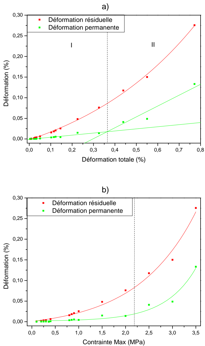
Figure V-8 : Evolution des déformations résiduelle et permanente en fonction de la déformation totale (a) et de la contrainte maximum (b).
