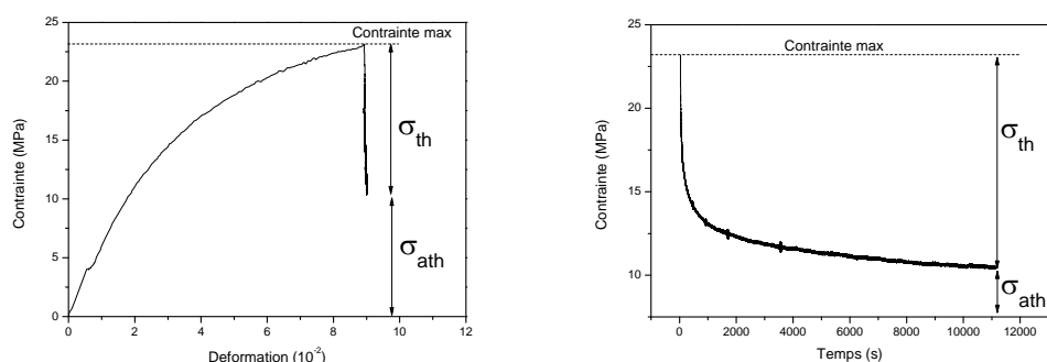
Figure V-19 : Courbes de contrainte déformation et de relaxation de contrainte avec les composantes thermique et athermique.
