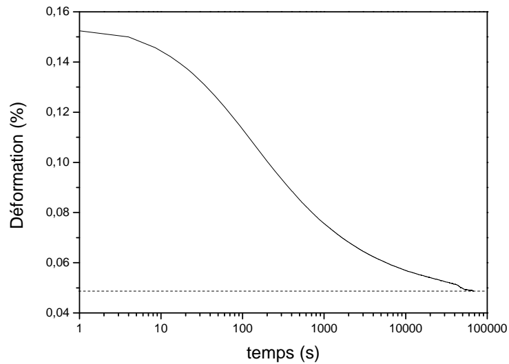
Figure V-7 : Recouvrance menée à la suite de l'essai de charge-décharge réalisé pour \varepsilon_t = 5,5 \cdot 10^{-3} .
