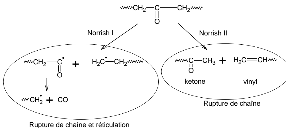
Figure IV- 37 : Schéma de dégradation du polyéthylène passant par les mécanismes Norrish I et II [9].
