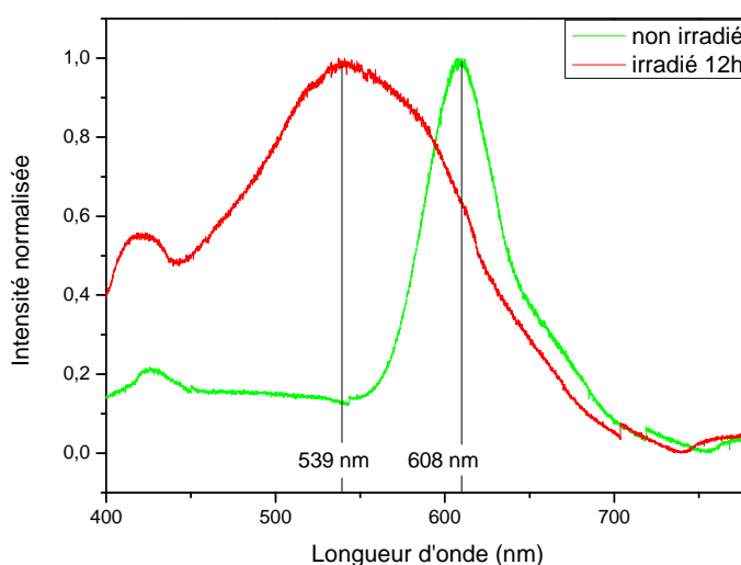
Figure IV- 4 : Spectres de fluorescence de deux échantillons de PEHD dopés en rhodamine 101 (500ppm), non irradié et irradié pendant 12h à 254 nm.
