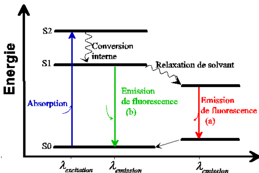
Figure II-2 : Diagramme de Jablonski [2].
