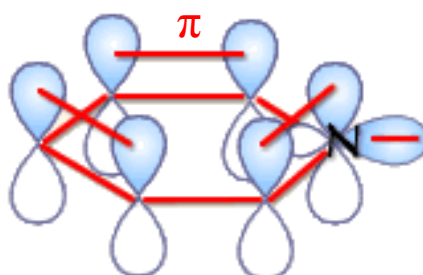
Figure II-1 : Schéma de la molécule de pyridine possédant un cycle aromatique et des liaisons \pi .
