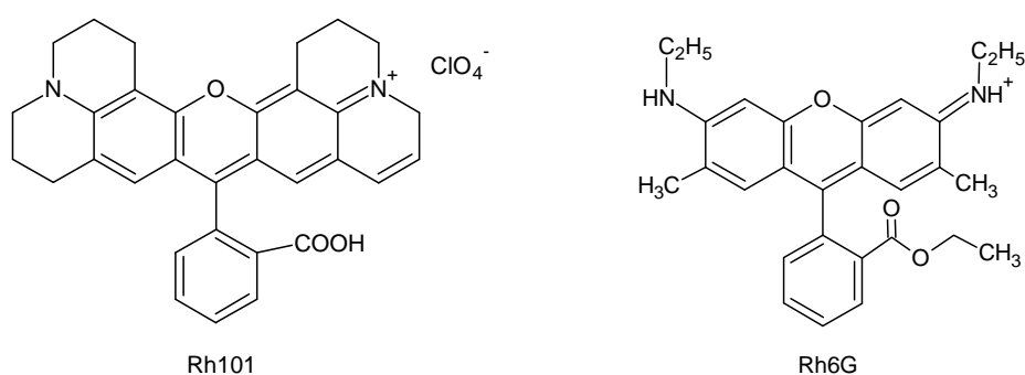
Figure III-2 : Schéma des molécules de colorants : rhodamine 101 (Rh101) et rhodamine 6G (Rh6G).
