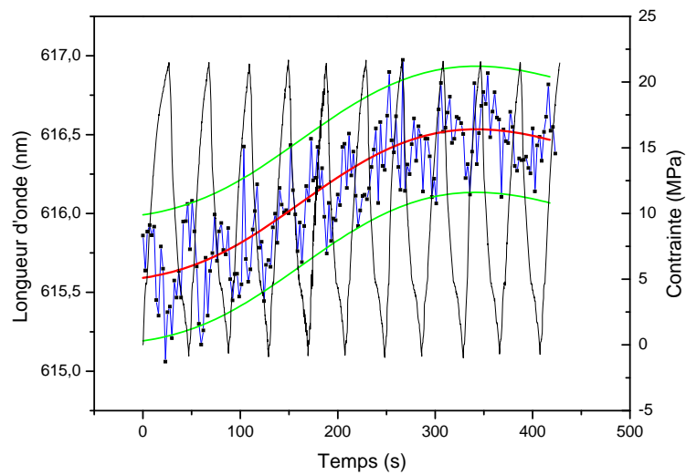
Figure V-27 : Corrélation en fonction du temps de l'évolution de la longueur d'onde de fluorescence et de la contrainte appliquée au cours de cycle de charge et décharge. Réalisée sur 10 cycles.
