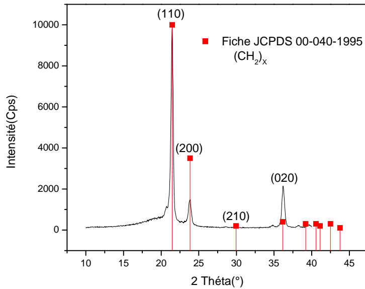
Figure III-8 : Diffractogramme du polyéthylène haute densité pur.
