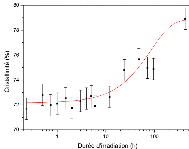
Figure IV- 13 : Evolution du taux de cristallinité au cours de l'irradiation UV.
