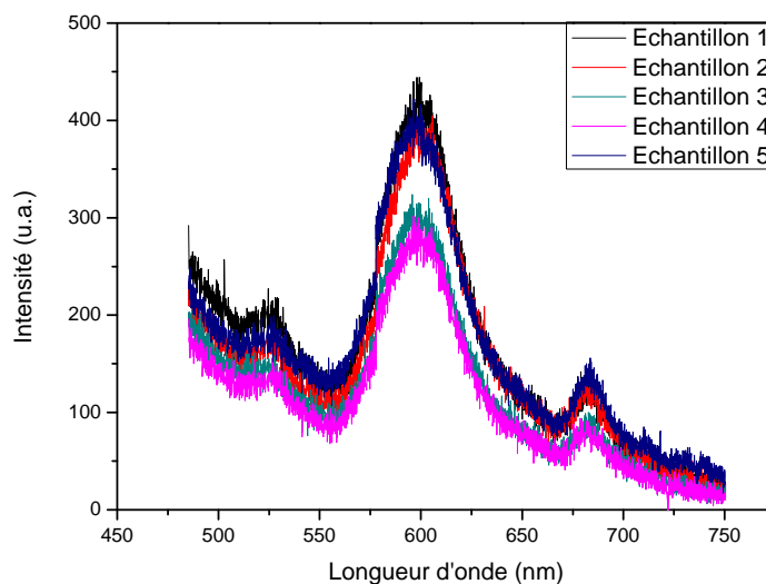
Figure V-10 : Spectres de fluorescence pour cinq échantillons de PEHD + Rh101 non déformés, chaque spectre est issu de la moyenne entre cinq acquisitions.
