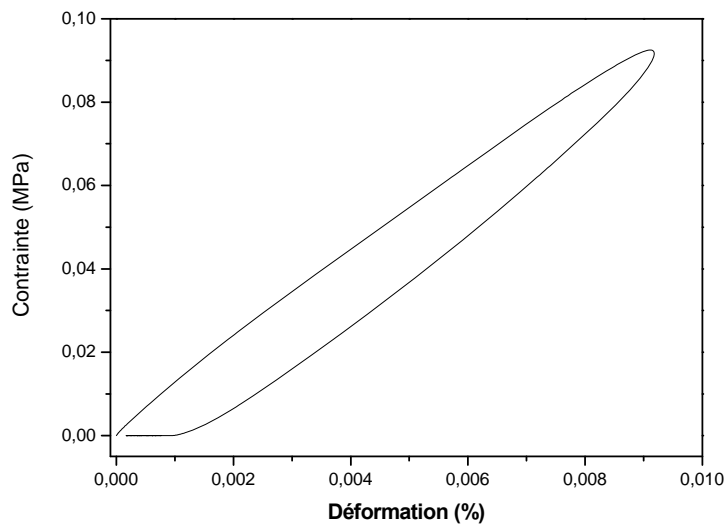
Figure V-4 : Essai de charge-décharge-recouvrance réalisé à 1 mm/min.
