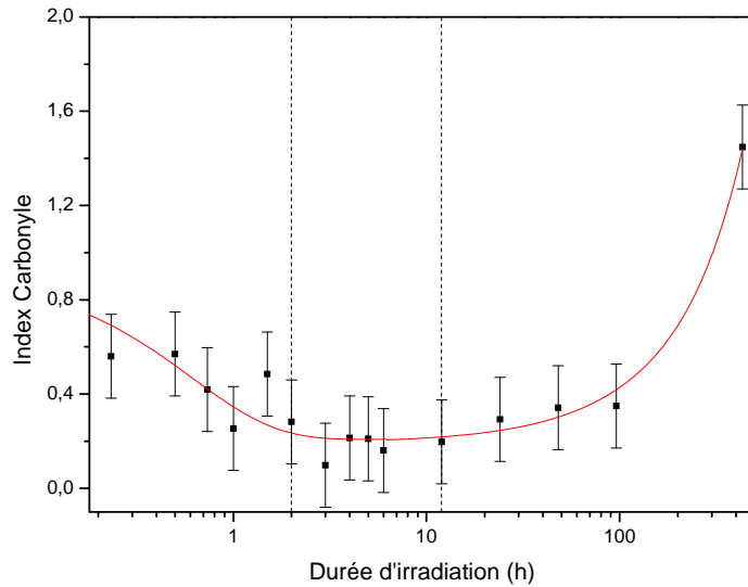
Figure IV- 11 : Evolution du produit de dégradation carbonyle en fonction de la durée d'exposition au rayonnement UV. Cas particulier d'une campagne d'essais avec des échantillons initiaux possédant une forte quantité de carbonyle.
