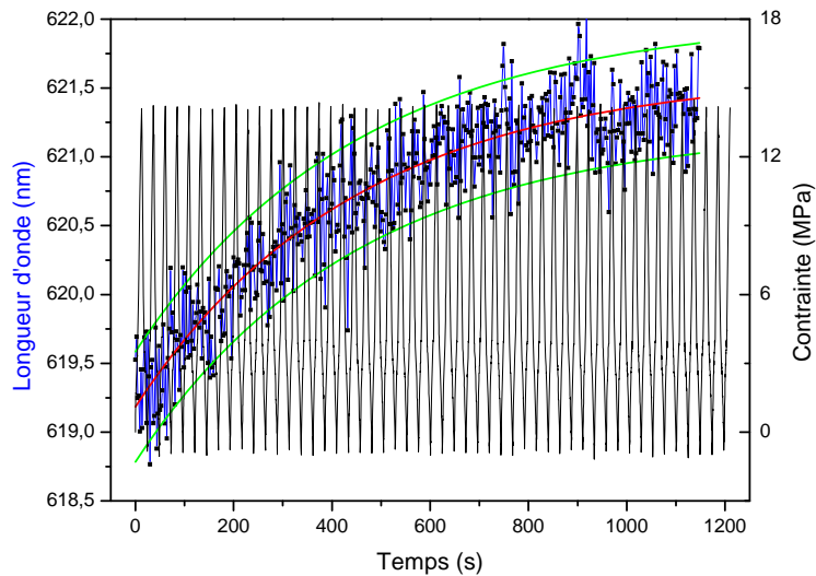
Figure V-33 : Corrélation en fonction du temps de l'évolution de la longueur d'onde de fluorescence et de la contrainte appliquée au cours de cycle de charge et décharge. Essai réalisé sur 50 cycles.
