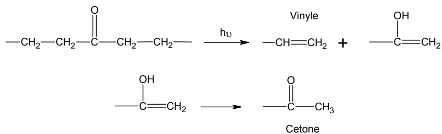
Figure I-16 : Mécanisme de dégradation de type Norrish II conduisant à de la rupture de chaîne et à la production de vinyle et de cétone [29-31].
