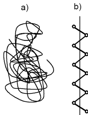
Figure I-5 : Conformations globales de la chaîne macromoléculaire du polyéthylène; a) Pelote statistique; b) Zigzag plan.
