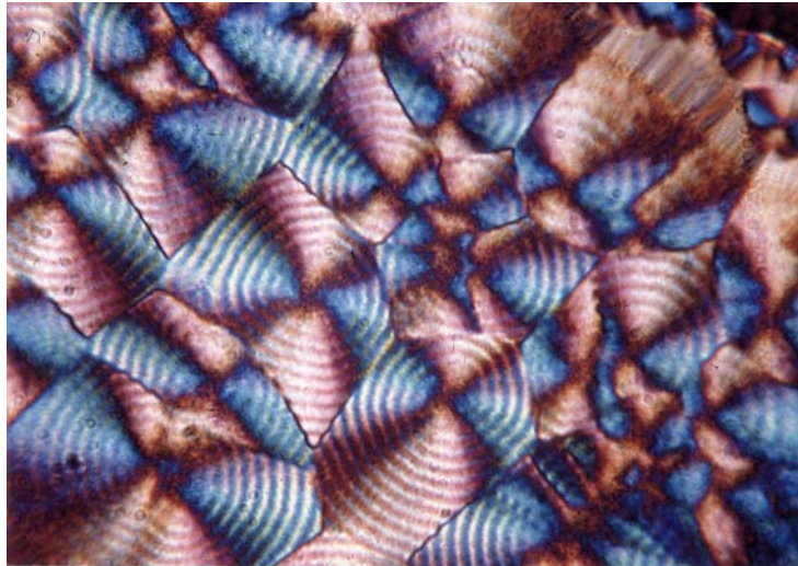
Figure I-9 : Sphérolites d'un polyéthylène observés en microscopie optique en lumière polarisée.
