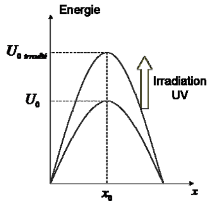
Figure IV- 34 : Modification de la barrière d'énergie visant à augmenter l'énergie U_0 .
