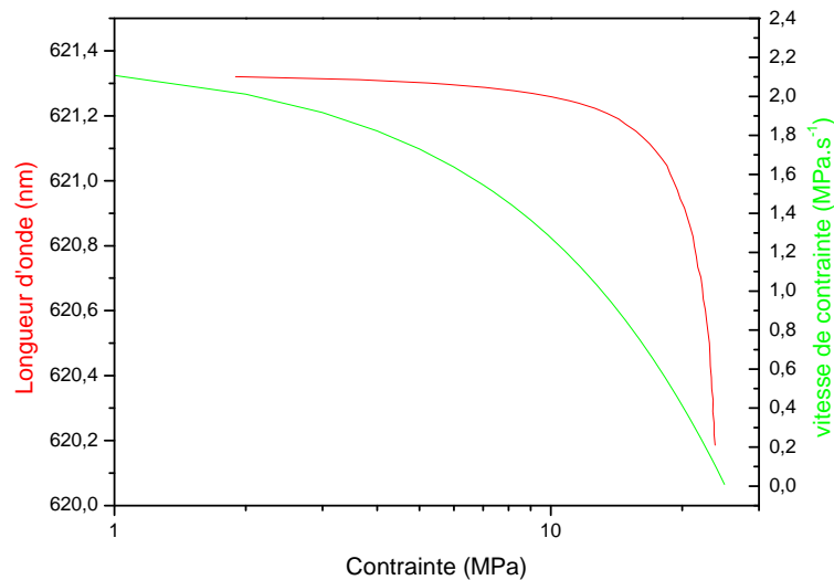
Figure V- 18 : Evolution de la longueur d'onde et de la vitesse de contrainte en fonction de la contrainte appliquée à l'échantillon au cours d'un essai en traction.
