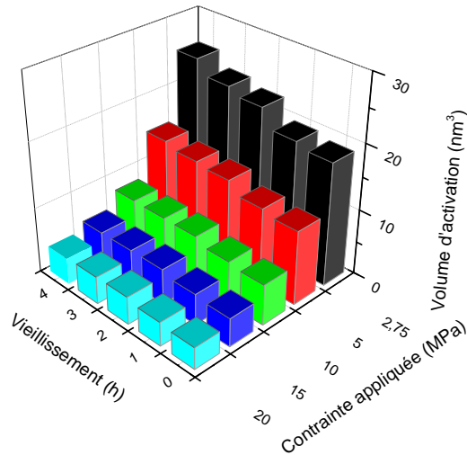
Figure IV- 31 : Evolution des volumes d'activation simulés en fonction du vieillissement et de la contrainte.
