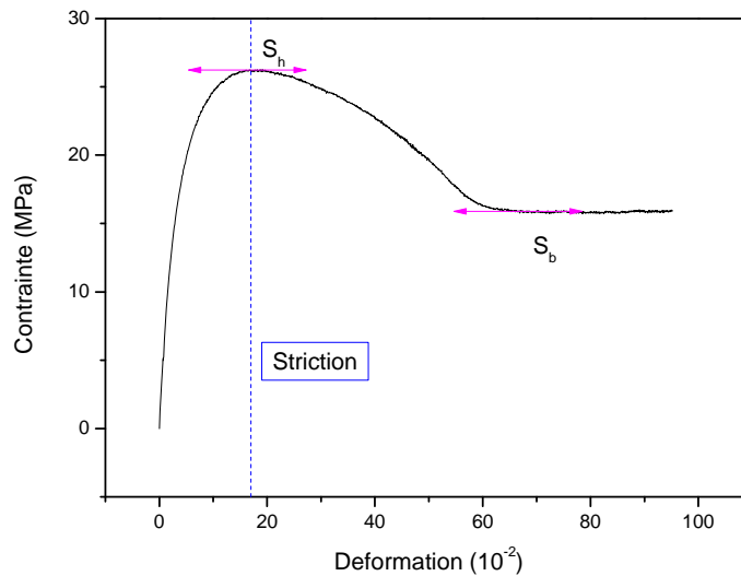
Figure V-1 : Courbe de déformation d'un échantillon de polyéthylène haute densité. S_b et S_h représentant respectivement les seuils d'écoulement bas et haut.
