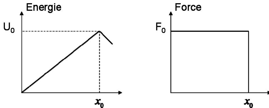
Figure IV- 24 : Profil de la barrière d'énergie et de la fonction force correspondante. La barrière a la forme d'un triangle, et la force, la forme d'un échelon.
