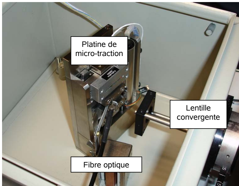
Figure II-8 : Photo du positionnement de la platine de traction dans l'enceinte d'analyse de fluorescence.
