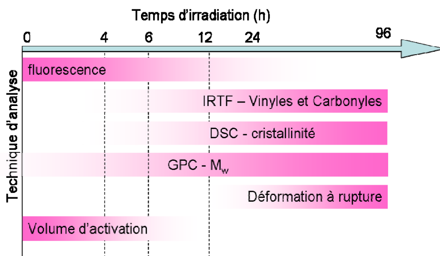
Figure IV- 38 : Evolution de la sensibilité de chaque technique d'analyse en fonction de l'échelle de temps.
