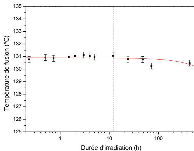
Figure IV- 14 : Evolution de la température de fusion des échantillons en fonction de l'irradiation UV.
