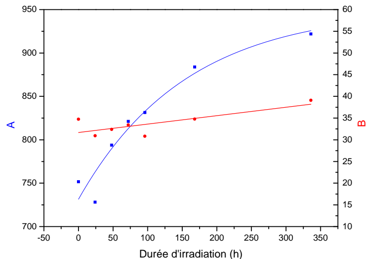
Figure IV- 20 : Evolution des constantes A et B calculées à partir des courbes d'érouissage en fonction du vieillissement UV.
