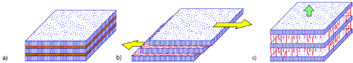
Figure I-20 : Mécanisme de déformation dans la phase amorphe interlamellaire : (a) état non déformé, (b) glissement interlamellaire et (c) séparation interlamellaire.
