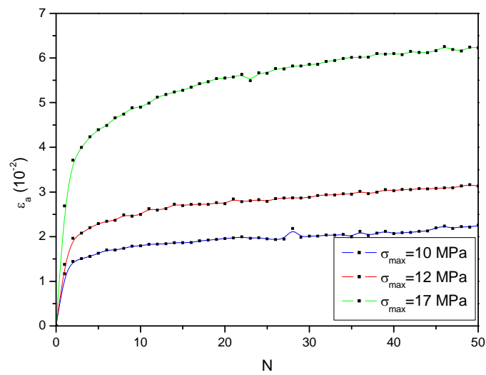
Figure V-37 : Evolution de la déformation absolue \epsilon_a au cours des cycles de charge décharge N pour différentes valeurs de contrainte maximum.
