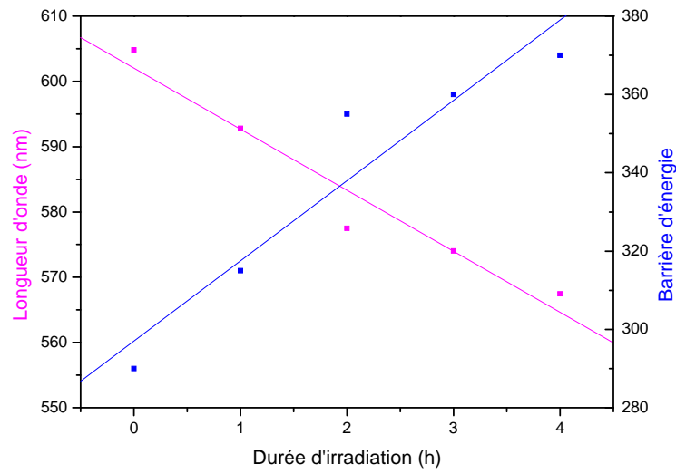
Figure IV- 35 : Evolutions comparées de la longueur d'onde d'émission et de la valeur de la barrière d'énergie en fonction de la durée d'irradiation UV.
