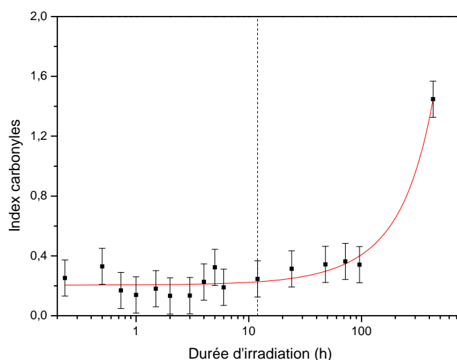
Figure IV- 9 : Evolution des produits de dégradation carbonyle en fonction de la durée d'irradiation UV.
