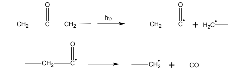
Figure I-15 : Mécanisme de dégradation de type Norrish I conduisant à de la rupture de chaîne et de la réticulation [29, 30].
