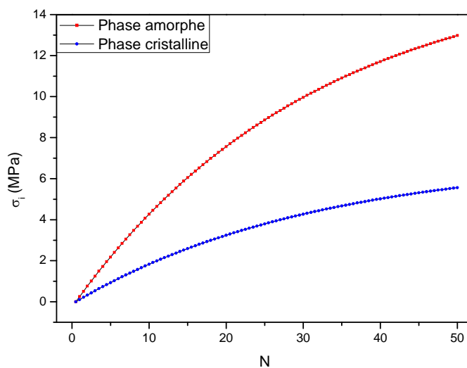
Figure V-34 : Evolution des contraintes internes dans la phase amorphe et dans la phase cristalline en fonction du nombre de cycle N.
