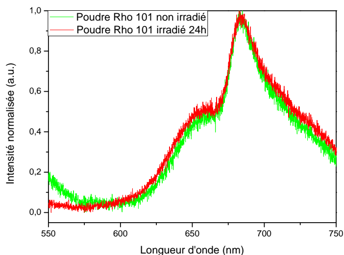
Figure IV- 2 : Spectres de fluorescence de rhodamine 101 sous forme de poudre, non irradié et irradié 24 h avec une longueur d'onde de 254 nm.
