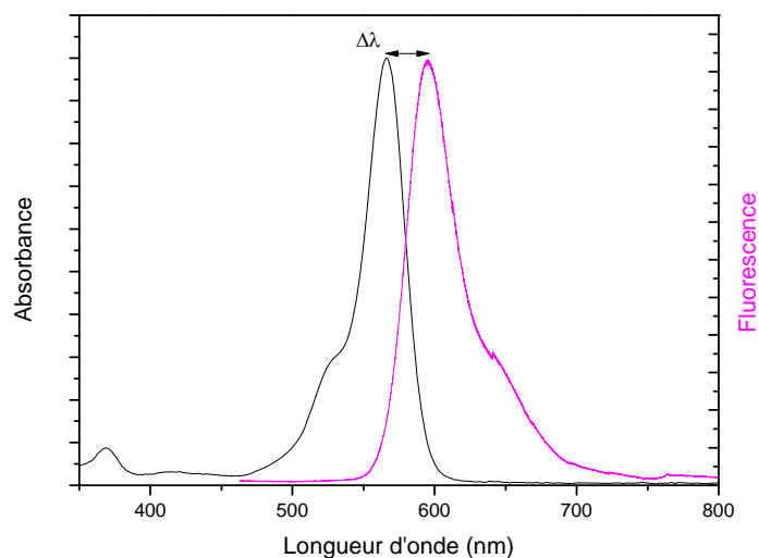
Figure II-3 : Spectre d'absorption et de fluorescence d'une molécule de rhodamine 101 dans l'éthanol à 25°C. \Delta\lambda représente le déplacement de Stokes.
