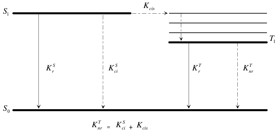
Figure II-4 : Schéma de Jablonski modifié.
