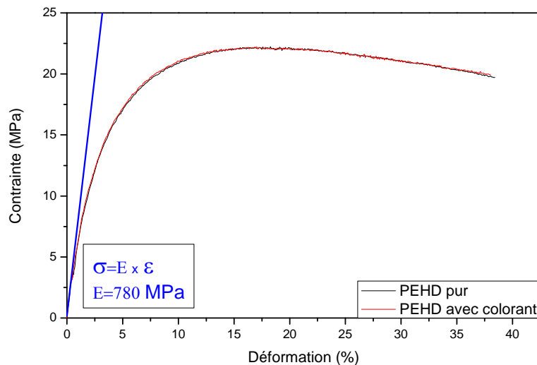
Figure III-18 : Courbes de traction des échantillons de PEHD pur et coloré obtenues avec une vitesse de déformation de 1mm/min.
