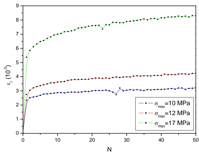
Figure V-38 : Evolution de la déformation de rochet \epsilon_r au cours des cycles de charge décharge N pour différentes valeurs de contrainte maximum.
