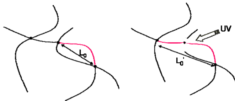
Figure IV- 29 : Représentation schématique de l'influence de la rupture de chaîne sur la longueur des segments
