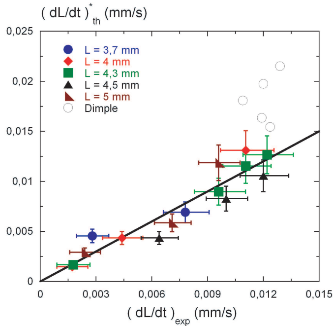
FIG. 3.11 – Corrélation entre la vitesse de mûrissement mesurée et la vitesse théorique à épaisseur de film variable.
