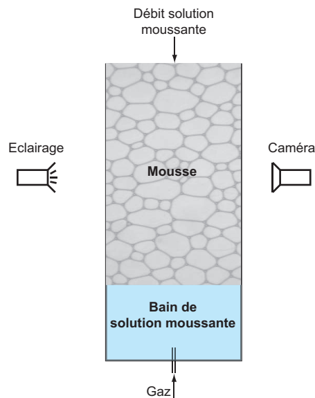
FIG. 2.12 – Schéma du dispositif expérimental.
