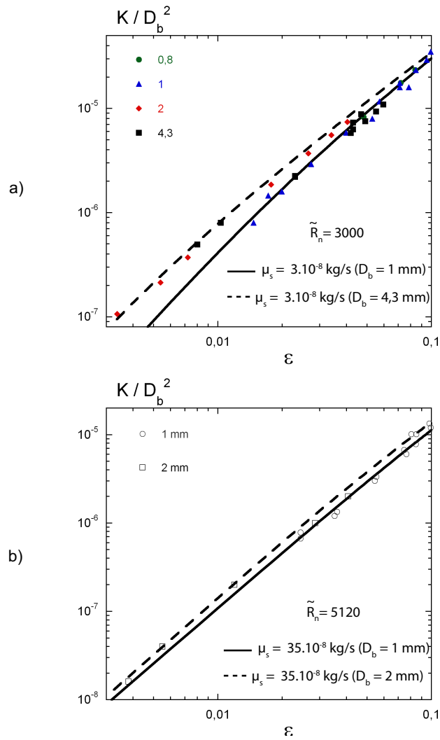
FIG. 2.19 – Modèles de Saint-Jalmes et al. . a) Solution de TTAB : \mu_s = 3.10^{-8} kg/s et \tilde{R}_n = 3000 . La ligne continue correspond à l'ajustement du modèle en prenant D_b = 1 mm. La ligne discontinue correspond à D_b = 4,3 mm avec les mêmes valeurs des paramètres libres. b) Solution de TTAB + DoH : \mu_s = 35.10^{-8} kg/s et \tilde{R}_n = 5120 . La ligne continue correspond à l'ajustement du modèle en prenant D_b = 1 mm. La ligne discontinue correspond à D_b = 2 mm avec les mêmes valeurs des paramètres libres.
