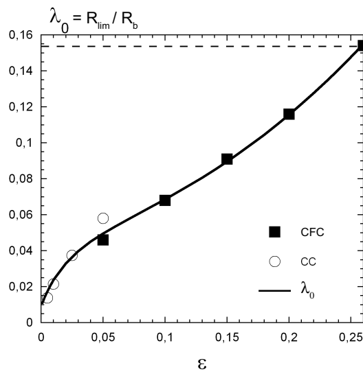
FIG. 6.2 – Evolution de la limite de capture géométrique en fonction de la fraction volumique de liquide. L'ajustement est donné par l'équation 6.2
