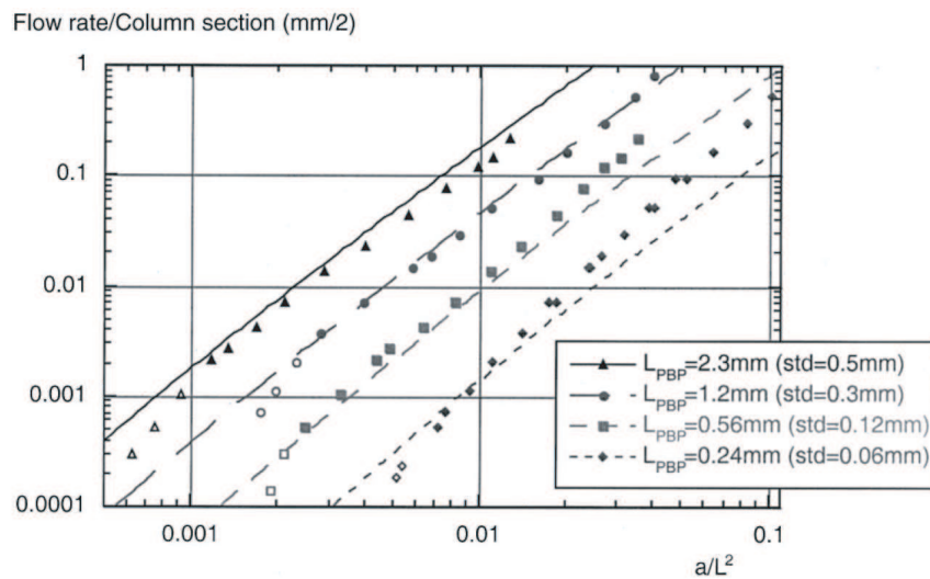
FIG. 1.16 – Vitesse débitante en fonction de A_{bdP}/L_{nn}^2 (relatif à la fraction volumique de liquide) pour une solution moussante de faible viscosité de cisaillement de surface. Tiré de [6].
