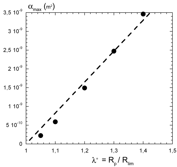
FIG. 6.10 – Evolution de \alpha_{\text{max}} en fonction du paramètre \lambda^* . La droite d'ajustement est donnée par l'équation 6.9
