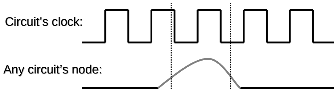
Figura 1: Uma falha transiente de longa duração (LDT)
