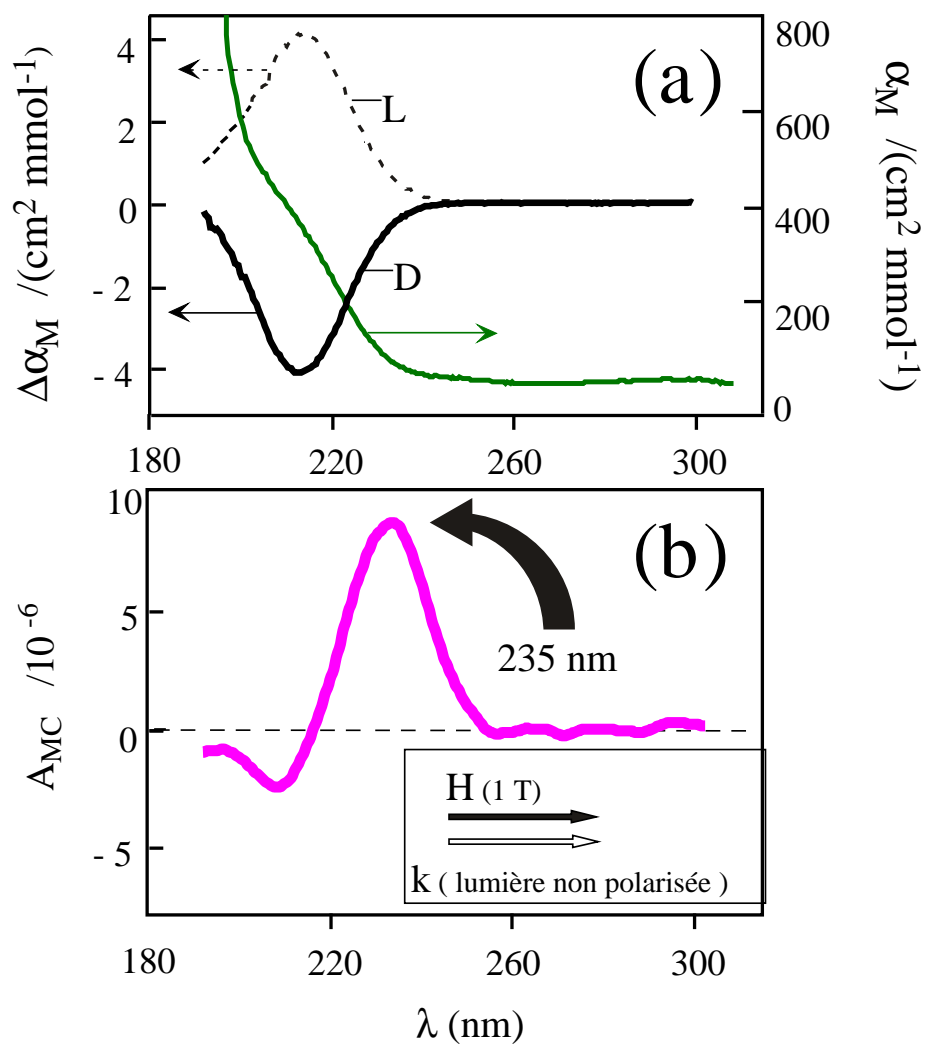
Figure 39 - (a) Coefficient d'extinction molaire \alpha_M et de dichroïsme circulaire \Delta\alpha_M pour des solutions de tartrates de calcium ( 1,3 \cdot 10^{-4} mol/L dans l'eau). Ligne continue : D-tartrate, ligne pointillée : L-tartrate. (b) Valeur déduite pour le coefficient d'anisotropie magnétochirale en absorption dans les tartrates pour un champ de 1 T et pour \vec{H} et \vec{k} parallèles.
