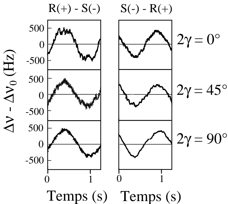
Figure 29 - Résultats des mesures d'indice magnétochiral pour trois polarisations incidentes. Les courbes de gauche sont obtenues avec C_1 remplie de R(+) -limonène et C_2 de S(-) -limonène, les courbes de droite avec les produits permutés. La polarisation sélectionnée est linéaire et inclinée d'un angle 2\gamma par rapport à l'axe (Ox).
