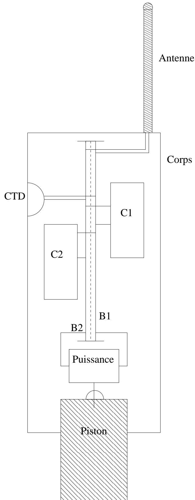
FIG. 3.2 – Schéma du flotteur
