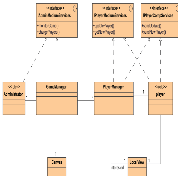
Figure III.1: Modèle du Médium de Synchronisation avec Gestionnaires de Rôle
