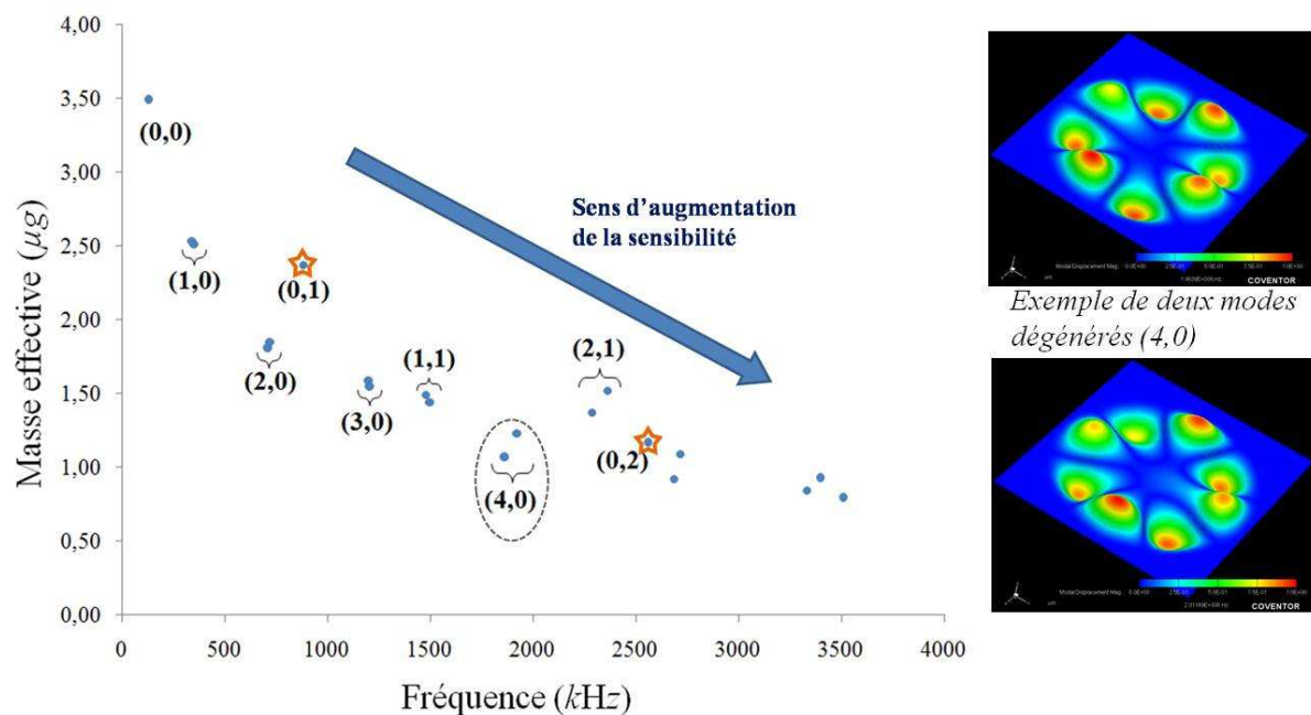
Figure 2.4 : Représentation graphique des résultats de l'analyse modale pour une micromembrane de rayon externe 400 \mu\text{m} et surmontée d'une pastille de PZT de rayon 200 \mu\text{m} .
