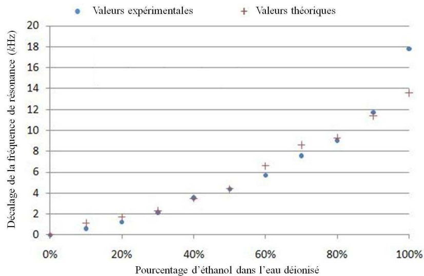
Figure 3.17 : Décalages de la fréquence de résonance, calculés (selon le modèle de Lamb étendu) et mesurés expérimentalement en fonction du pourcentage d’éthanol dans l’eau déionisée pour une membrane de rayon 440 \mu\text{m} vibrant selon le mode (0,1).
