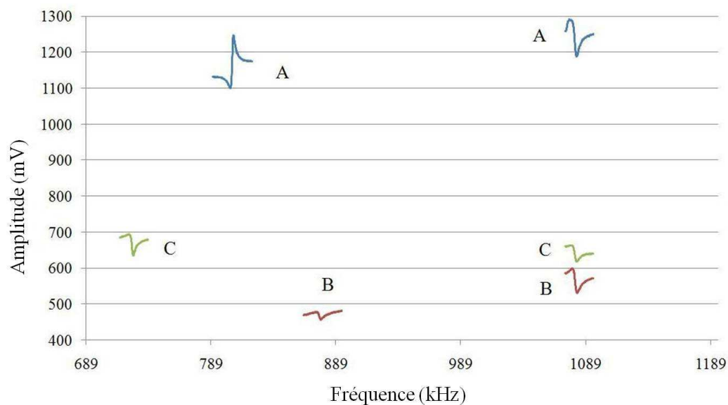
Figure 3.6 : Détail des spectres de résonances pour le mode de vibration (0,2) de trois membranes avec un rayon de 440\text{ }\mu\text{m} (courbe verte, C) avec un rayon de 430\text{ }\mu\text{m} (courbe bleue, A), avec un rayon de 420\text{ }\mu\text{m} (courbe rouge, B). Le pic de résonance apparaissant sur les trois spectres est caractéristique de la résonance de la membrane de référence vibrant également selon le mode de vibration (0,1) (rayon de 360\text{ }\mu\text{m} , pic localisé à 1077\text{ kHz} ).
