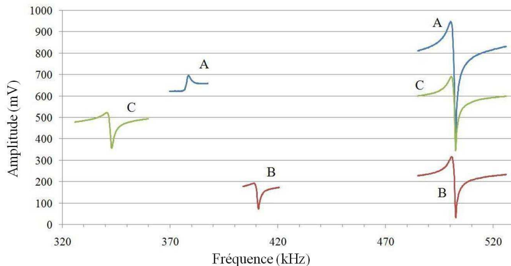
Figure 3.5 : Détail des spectres de résonances pour le mode de vibration (0,1) de trois membranes avec un rayon de 440\text{ }\mu\text{m} (courbe verte, C) avec un rayon de 430\text{ }\mu\text{m} (courbe bleue, A), avec un rayon de 420\text{ }\mu\text{m} (courbe rouge, B). Le pic de résonance apparaissant sur les trois spectres est caractéristique de la résonance de la membrane de référence vibrant également selon le mode de vibration (0,1) (rayon de 360\text{ }\mu\text{m} , pic localisé à 499\text{ kHz} ).
