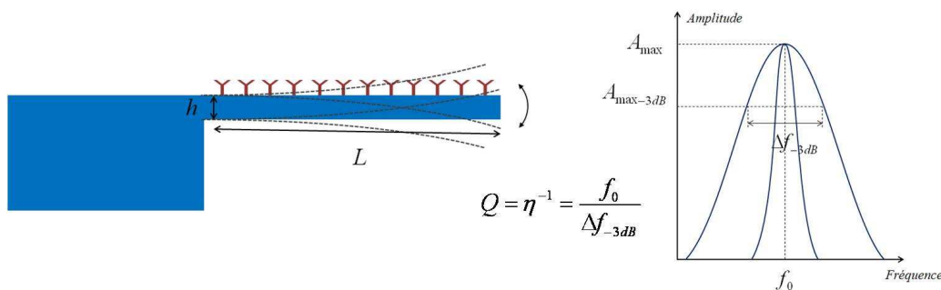
Figure 1.17: Principe de fonctionnement d'un BioMEMS dynamique, ici un levier dans un mouvement de vibration hors-du-plan. A droite, représentation schématique de deux courbes de résonance respectivement symboliques de facteur de qualité Q faible et élevé.
