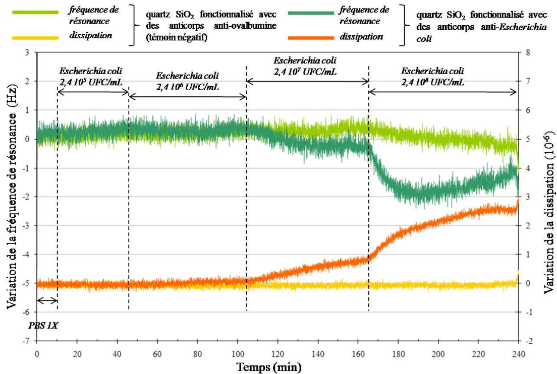
Figure 4.10 : Graphique des variations des fréquences de résonance et des dissipations pour la 7ème harmonique de 2 quartzes SiO 2 en parallèle, pendant l'injection d' Escherichia coli à différentes concentrations. Un des quartzes est fonctionnalisé avec un anticorps anti- Escherichia coli , l'autre avec un anticorps anti-ovalbumine (témoin négatif).
