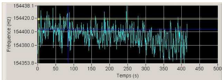
Figure 2.31 : En haut, deux captures d'écran représentatives de l'interface informatique associée à la carte électronique de commande. Les captures d'écran présentées montrent entre autres, la possibilité de réglage de la polarisation des piézorésistances mais également des paramètres d'amplification avec ou sans utilisation de la boucle de rétroaction positive. En bas, capture d'écran montrant un suivi en temps réel d'une micromembrane par détection piézorésistive, vibrant dans l'air et tel qu'affiché par l'interface informatique
