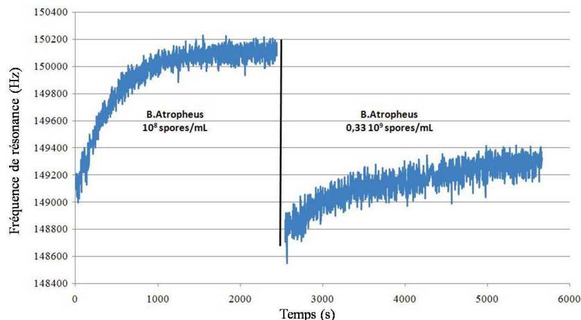
Figure 4.13 : Courbes de suivi en temps réel de la fréquence de résonance d'une micromembrane de 440 \mu\text{m} de rayon vibrant selon le mode (0,1) et fonctionnalisée avec des anticorps anti- Bacillus atrophaeus . Les deux signaux correspondent à l'injection, juste après la fonctionnalisation, de deux solutions de Bacillus atrophaeus concentrées à 10^8 spores/mL puis à 0,33 \cdot 10^9 spores/mL
