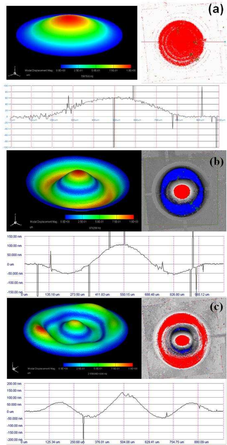
Figure 3.1 : (a) Forme du mode fondamental (0,0) d'une membrane de 465 \mu\text{m} de rayon, obtenu par simulation par éléments finis, comparé à l'image de surface et à la coupe de la déformée maximale au cours de la vibration obtenues par interférométrie optique. Les mêmes courbes sont présentées en (b) pour le mode (0,1) et en (c) pour le mode (0,2).
