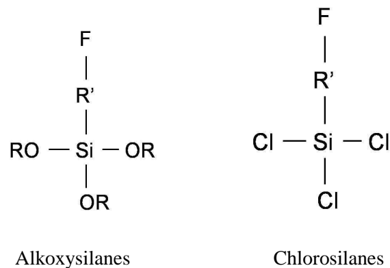
Figure 1.6 : Structure chimique de deux types de silanes communément utilisés pour l'immobilisation covalente de biorécepteurs sur des substrats de verre. R et R' sont des radicaux libres et F représente le groupement fonctionnel.
