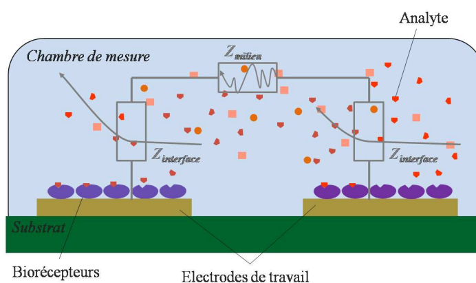
Figure 1.12: Schéma descriptif du principe d'une transduction conductimétrique. Ici, la mesure s'effectue en mesurant l'impédance entre les deux électrodes de travail. Le sens de variation des impédances d'interfaces en fonction de la quantité de couples biorécepteurs/analytes a été choisi arbitrairement.
