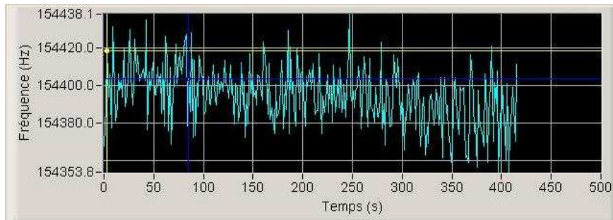
Figure 3.7 : Capture d'écran de l'interface informatique, présentant un graphe obtenu lors du suivi en temps réel de la fréquence de résonance d'une membrane vibrant dans l'air.
