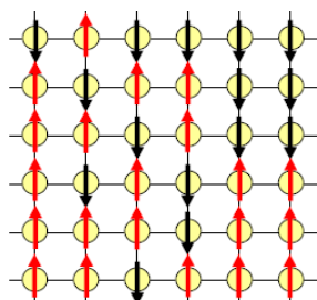
Illustration 22 : Modèle d'Ising
