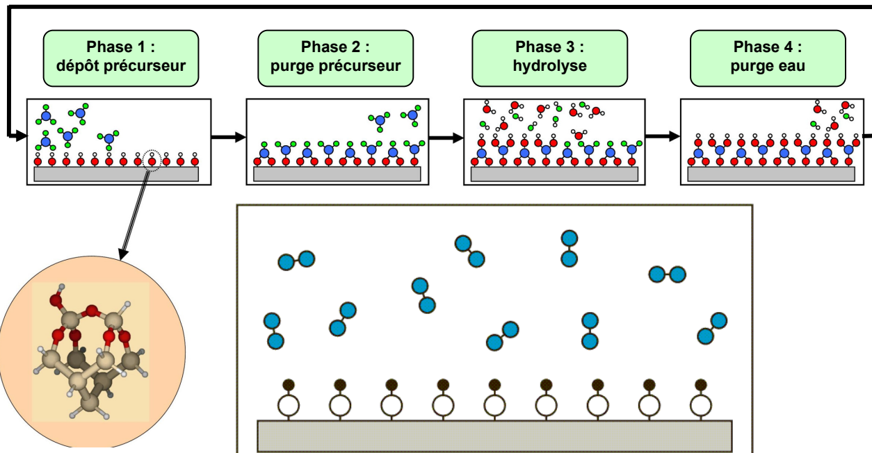
Illustration 15 : Principe du dépôt par ALD
