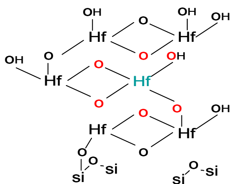
Illustration 60 : Schéma simplifié d'une suite de motifs densifiés illustrant l'augmentation du nombre de coordination des atomes d'hafnium durant le dépôt.
