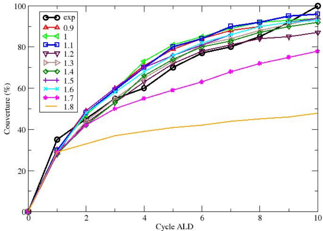
Illustration 54 : Étalonnage de l'énergie de densification basé sur le taux de couverture expérimental [Blin 2003]
