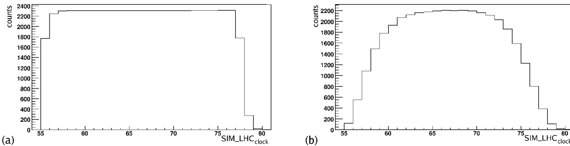
FIG. 4.15 – Simulation de collisions proton-proton minimum bias à \sqrt{(s)} = 14 \text{ TeV} : nombre de déclenchements en coïncidence 3/4 All p_t en fonction de la variable SIM\_LHC_{clock} pour le résultat de référence (a) et après introduction de toutes les sources de dispersions (b).
