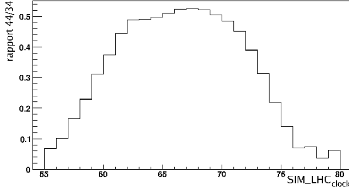
FIG. 4.14 – Simulation de collisions proton-proton minimum bias à \sqrt{(s)} = 14 \text{ TeV} : rapport entre les coïncidences 4/4 All p_t et 3/4 All p_t en fonction de la variable SIM\_LHC_{clock} pour un résultat de référence couplé à l'ajout de toutes les sources de dispersion.
