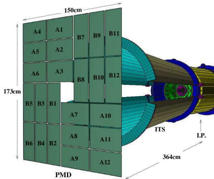
FIG. 2.16 – Schéma du détecteur PMD.
