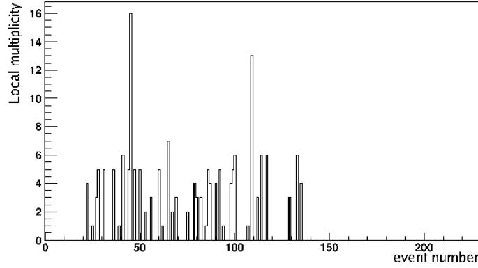
FIG. 6.8 – Déclenchement ZDC : multiplicité de déclenchements au niveau Local en fonction du numéro d'événement.
