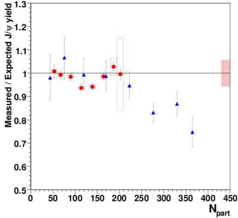
FIG. 1.15 – Rapport entre les nombres de J/\Psi mesurés et attendus en fonction du nombre de nucléons participants pour des collisions Pb-Pb à \sqrt{s_{NN}} = 17.3 GeV (NA50, triangles bleus) et In-In à \sqrt{s_{NN}} = 17.3 GeV (NA60, cercles rouges) au SPS [50]. Les données sont corrigées de l'absorption nucléaire normale et du shadowing.
