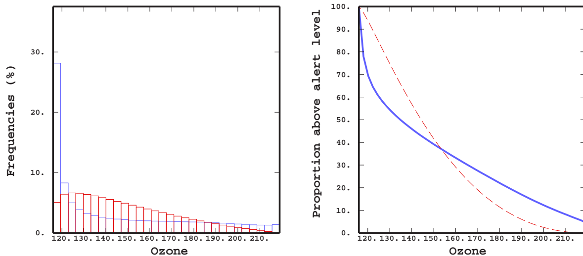
FIG. 4.5 – A gauche : histogrammes des blocs (en bleu) et des cellules (en rouge). A droite : courbes de proportions de blocs (bleu) et de cellules (en rouge) au-dessus de valeurs limites d’ozone.
