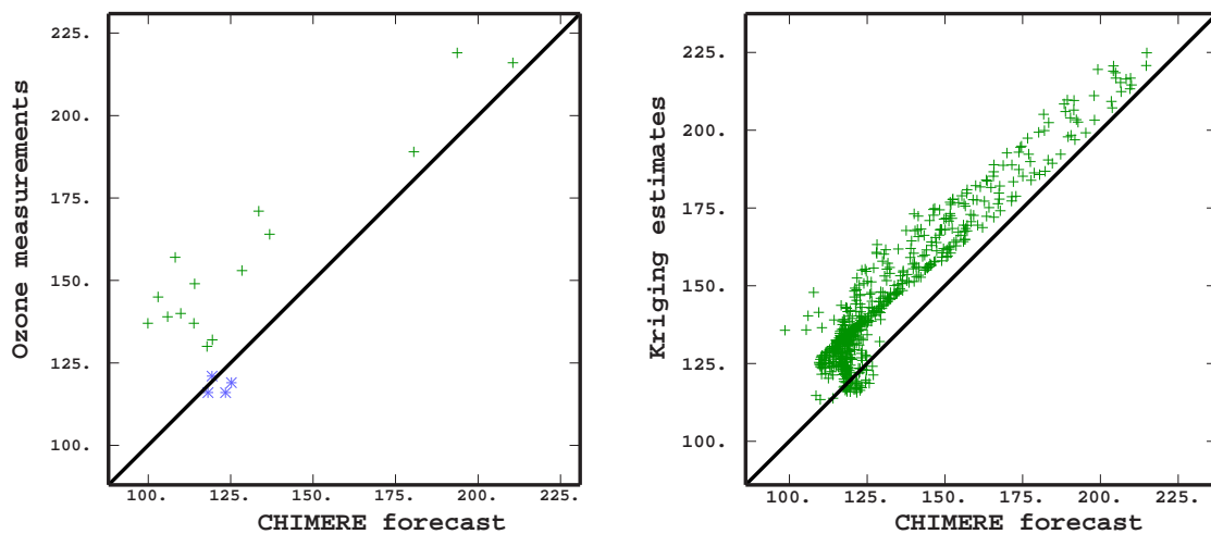
FIG. 4.2 – A gauche : les valeurs de Chimère (abscisse) et les mesures des 19 stations (ordonnée). A droite : les valeurs de Chimère (abscisse) et les valeurs obtenues par krigeage avec dérive externe (ordonnée).
