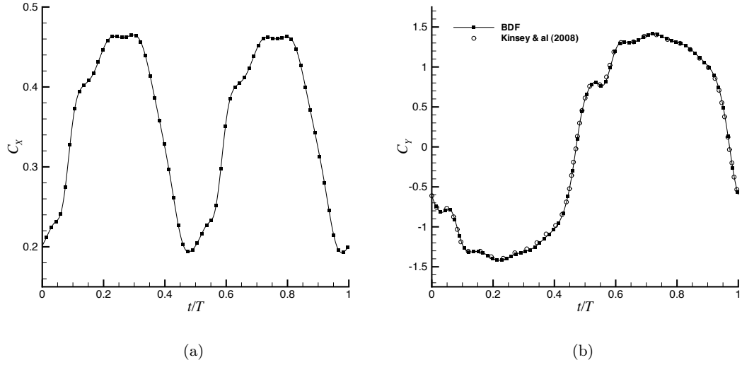
Fig. 3 Cas test PP. (a): Evolution du C_X evolution en utilisant notre approche BDF. (b): Evolution du C_Y calculé dans [14] et avec notre approche BDF
