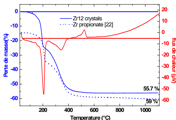
Figure III. 14. Analyse thermogravimétrique comparant Zr(prop)_4 et les cristaux de Zr12.
