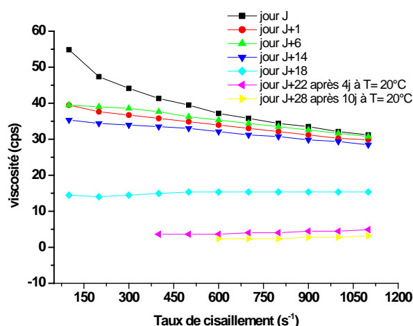
Figure III. 5. Evolution de la viscosité de la solution de précurseur Ce(EH)_3 (0.05M) au cours du vieillissement [2]. La solution est stockée à 4^\circ C et mesuré à T ambiante. Quelques points ont vieillis à 20^\circ C .
