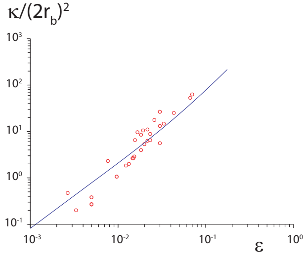
Fig. 2.18- La courbe représentant l'équation 2.23 est représentée en bleu, nos valeurs de perméabilité pour toutes les valeurs de r_b testées en fonction de \epsilon sont les points rouges, et sont en bon accord avec le modèle de perméabilité, pour R_n=480 et Bo=0,25 , comme sur la figure 2.9)
