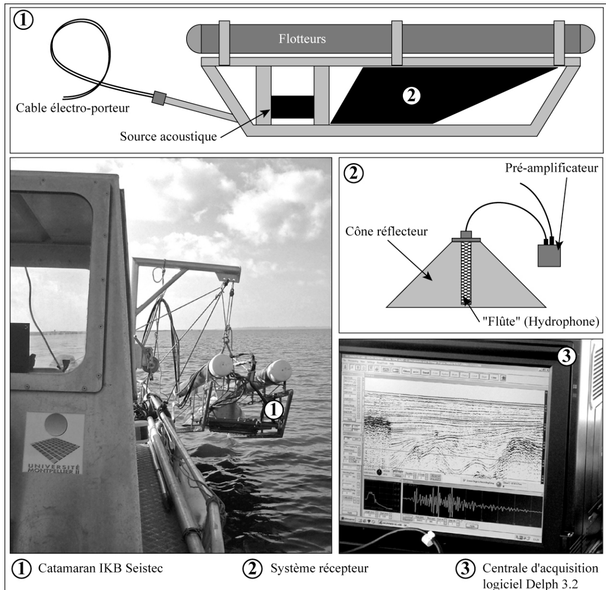
FIG. 3.1 – Le boomer IKB Seistec. Le regroupement de la source acoustique et des hydrophones récepteurs sur le même catamaran font de cet appareillage un outil particulièrement adapté à la prospection en faible bathymétrie.
