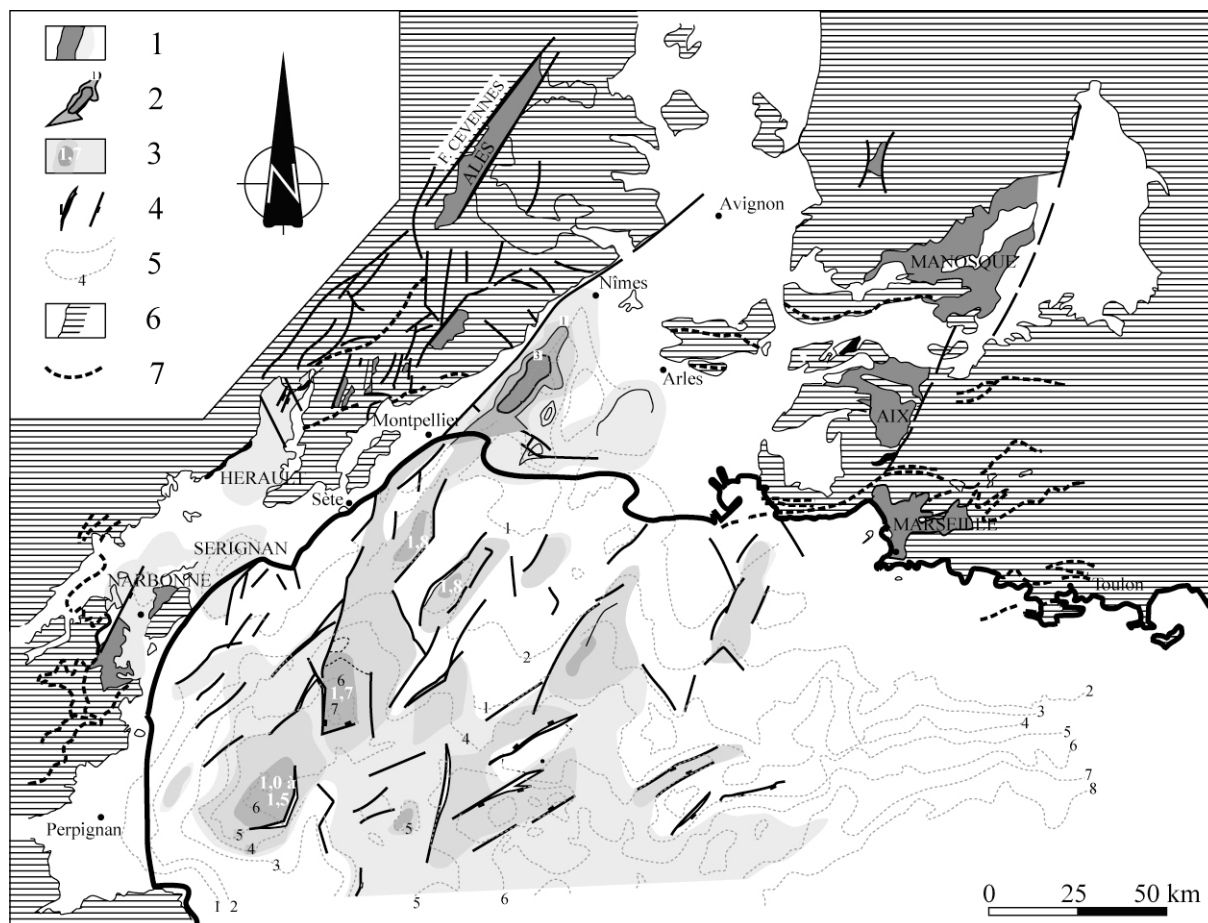
FIG. 1.4 – Carte simplifiée du rift du Golfe du Lion et des fossés du Sud-est (Guennoc et al., 2000). 1.fossé à terre ; 2.Isopaques en milliers de mètres dans le bassin de Camargue d'après Bénédicte (1996); 3. épaisseur maximale en secondes temps double des séries syn-rift en mer; 4. failles du rift; 5. isobathes du substratum pré-rift (en milliers de mètres); 6. limites d'affleurement du substratum pré-rift à terre; 7. principales structures pyrénéennes à terre.
