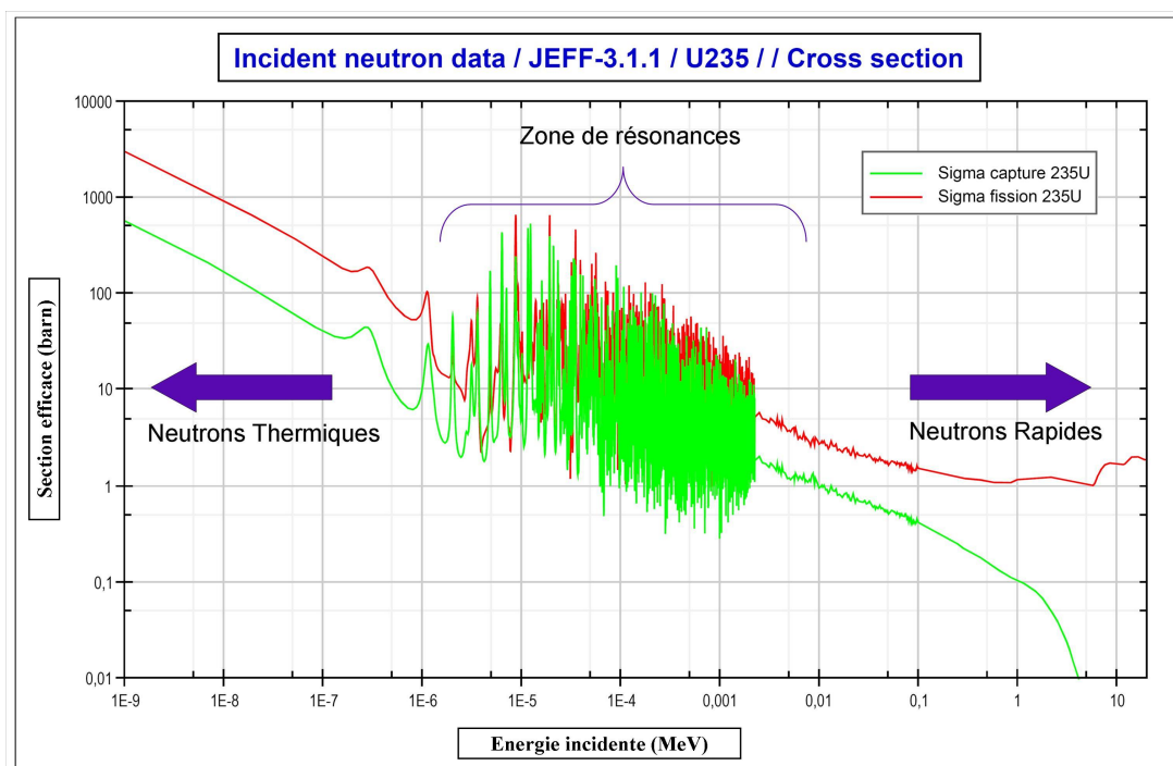
FIGURE I.2 – Section efficace de capture neutronique et de fission de l' ^{235}\text{U} en fonction de l'énergie du neutron incident [NEA10].
