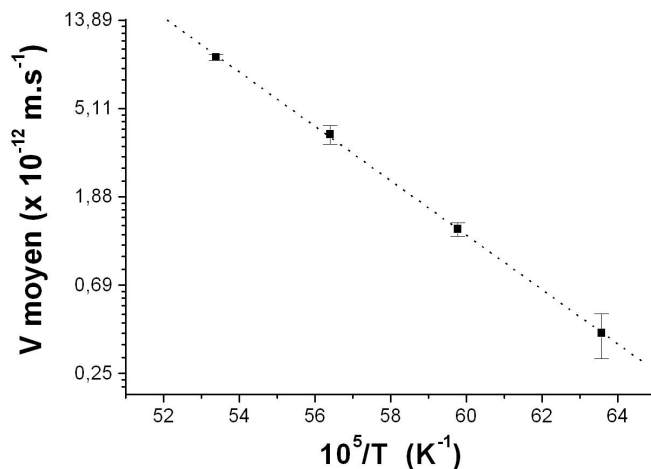
FIGURE II.17 – Diagramme de type Arrhénius de la vitesse de transport, mesurée sur le lot 2.
