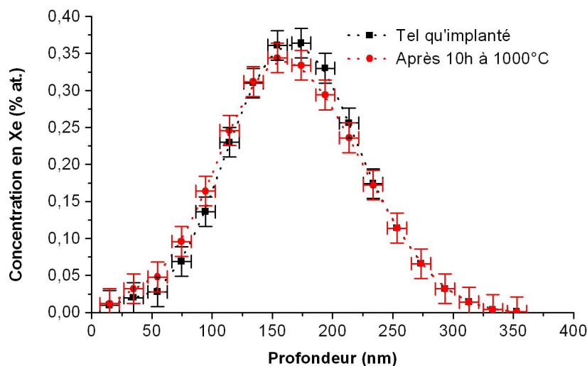
FIGURE II.5 – Evolution de la concentration en xénon en fonction de la profondeur après un traitement thermique de guérison des défauts de surface à 1000^{\circ}\text{C} pendant 10 heures.
