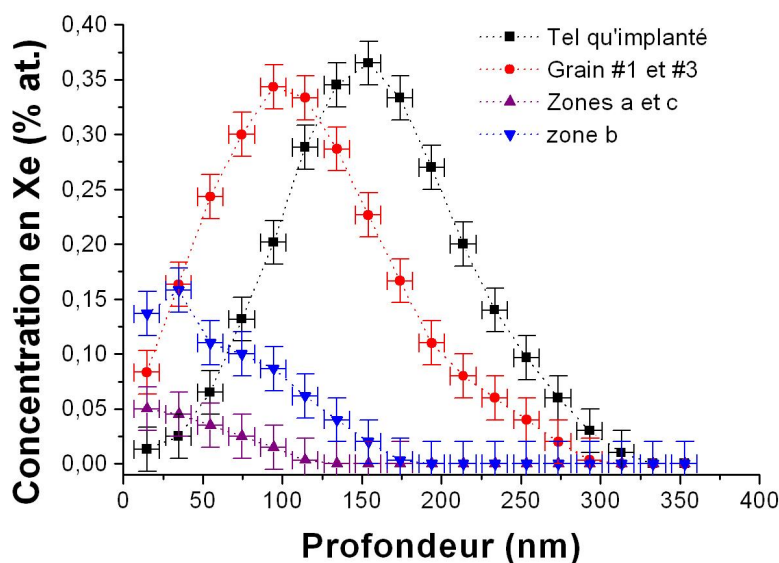
FIGURE III.2 – Profils de concentration en Xe du lot 2 obtenus sur les zones analysées en micro-sonde après 5 heures à 1500° C. Le profil tel qu'implanté est identique quelle que soit la zone sondée.
