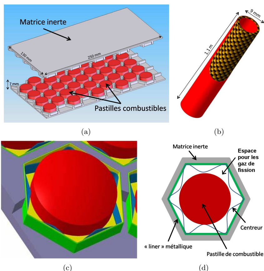
FIGURE I.6 – Plaque (a) et aiguille (b) des différents concepts de géométrie combustible telles qu'envisagées par le CEA pour le RNR-G. Zoom (c) et représentation schématique (d) d'une alvéole du concept à plaque.
