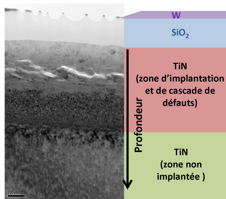
FIGURE IV.13 – Image MET et représentation schématique d'une lame de microscopie électronique en coupe transverse telle que fabriquée au cours de cette étude.
