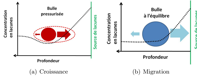
FIGURE I.10 – Schémas à une dimension de croissance (flèches rouges) et de migration (flèches bleues) des bulles proches d'une source sous pression (a) et à l'équilibre lorsque le gradient de lacunes est maintenu (b). La ligne pointillée noire représente la concentration en lacunes.
