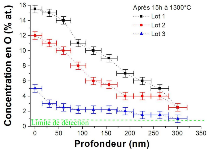
FIGURE III.9 – Profils de concentration en oxygène en fonction de la profondeur obtenus pour les 3 lots, après 15 heures à 1300°C.
