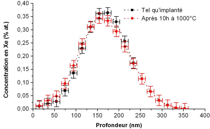
FIGURE II.5 – Evolution de la concentration en xénon en fonction de la profondeur après un traitement thermique de guérison des défauts de surface à 1000^{\circ}\text{C} pendant 10 heures.
