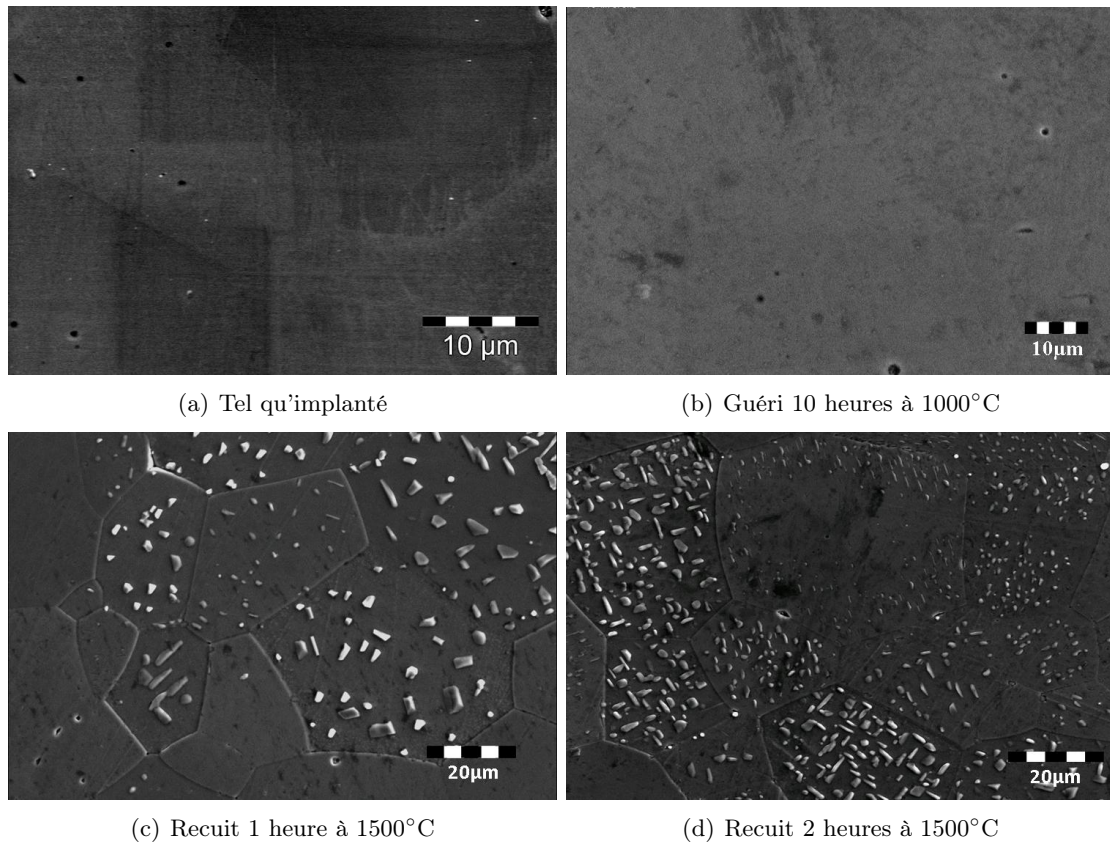
FIGURE III.10 – Comparaison des clichés MEB de la surface non implantée d'un échantillon du lot 2 demi-implanté tel qu'implanté (a), après guérison à 1000°C pendant 10 heures (b) et après recuit à 1500°C pendant 1 heure (c) et 2 heures (d).
