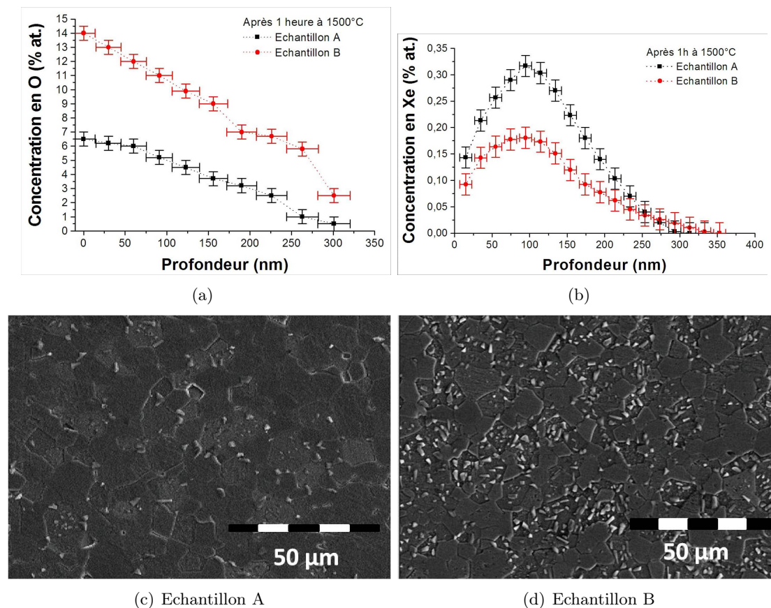
FIGURE III.12 – Profils de concentration (a) en oxygène et (b) en xénon, comme fonction de la profondeur après 1 heure à 1500°C pour deux échantillons du lot 1. Clichés MEB de la surface de ces échantillons A (c) et B (d).
