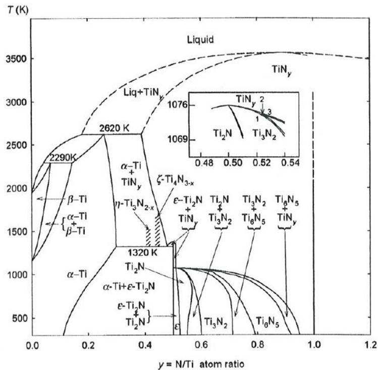
FIGURE I.7 – Diagramme de phase du nitrure de titane. D'après [Gus01].
