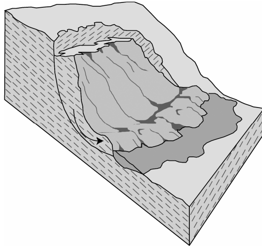
Figure 1-4 : Schéma d'un glissement rotationnel en milieux rocheux
