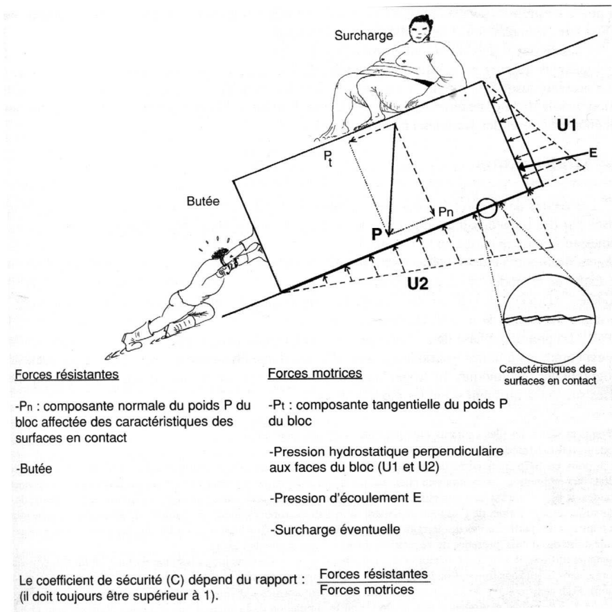
Figure 1-13 : schéma récapitulant les principales forces macroscopiques mises en œuvre lors de la destabilisation d'un versant d'après Besson, 1996
