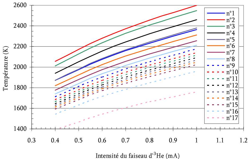
Fig. 41 _ Evolution de la température maximale des disques de l'empilement en fonction de l'intensité du faisceau d 3 He pour le graphite flexible d'épaisseur 75 µm.
