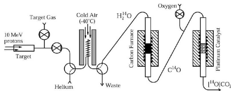
Fig. 15 _ Schéma du système de production utilisé à LBNL pour produire l' ^{14}\text{O} [104].
