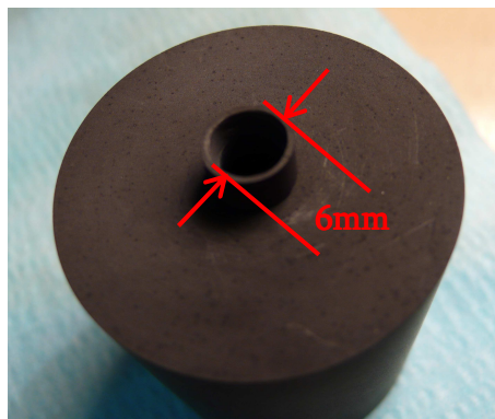
Fig. 54 _ Photo du couvercle de la cavité, comprenant l'orifice d'injection des ions.
