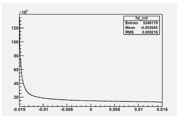
Fig. 126_ Histogramme représentant le lieu des collisions au cours de la vie de l'alcalin.
