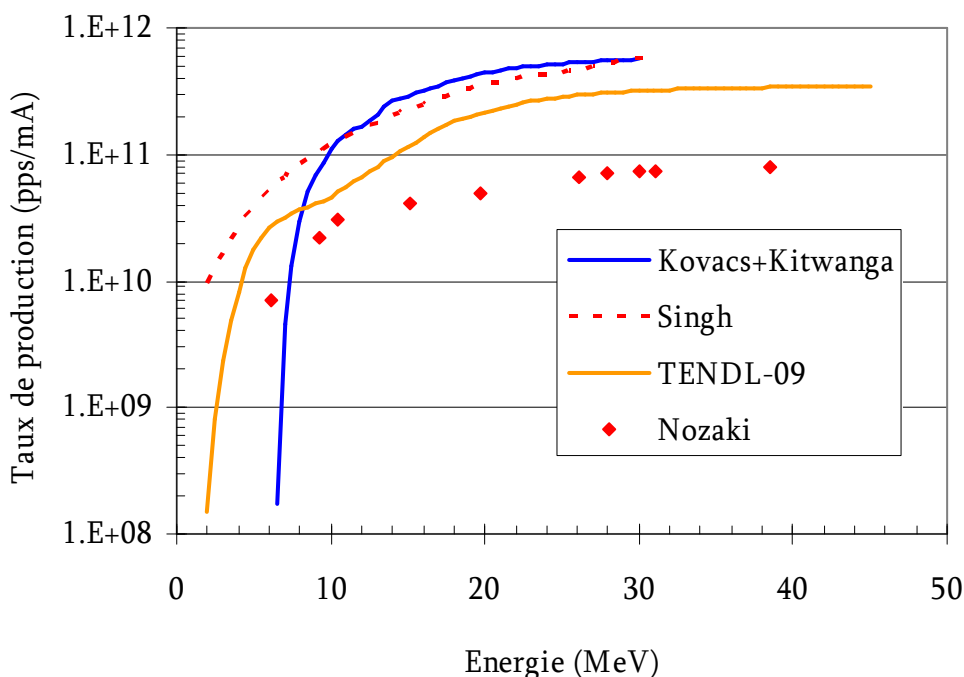
Fig. 18_ Calculs du taux de production d 14 O à saturation dans une cible épaisse pour un faisceau incident de 1 mA en fonction de l'énergie incidente. L'activité à saturation mesurée par Nozaki et Iwamoto est aussi présentée. La courbe bleu correspond à la réaction ^{14}\text{N}(p,n)^{14}\text{O} et les autres à ^{12}\text{C}(\beta\text{He},n)^{14}\text{O} .
