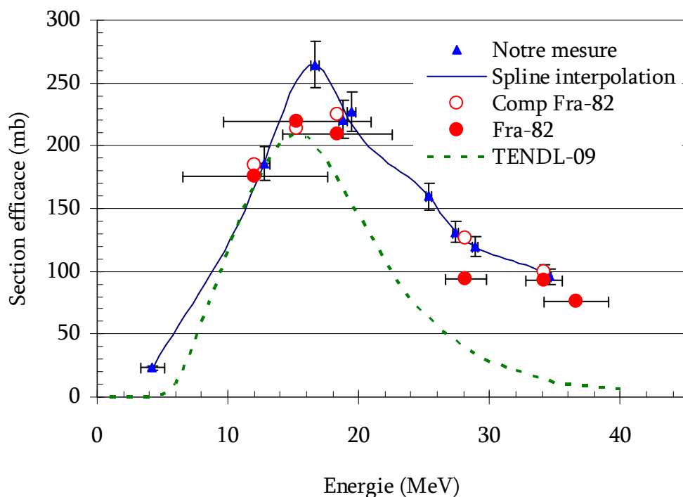
Fig. 27_ Comparaison de notre mesure de section efficace aux valeurs de Frantsvog et al. et à celle de la base de données TENDL-09 pour la réaction ^{27}\text{Al}(\beta\text{He},2p)^{28}\text{Al} .
