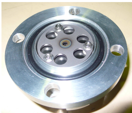
Fig. 53 _ Photo de la partie interchangeable du canon à ions. Elle est constituée de l'émetteur d'ions alcalins et d'une électrode d'extraction.
