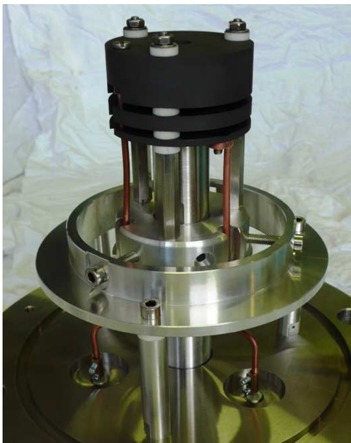
Fig. 80 _ Photo du canon à ions adapté pour effectuer les tests sur la SIS de SPIRAL 2.
