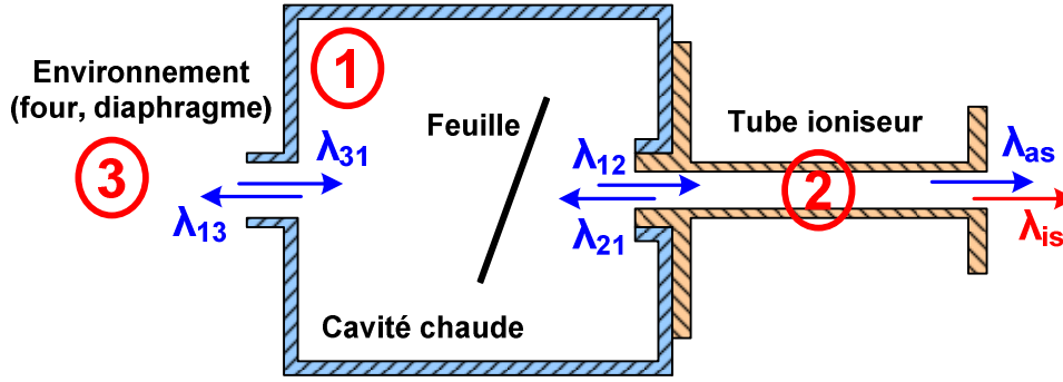
Fig. 64 _ Schéma de principe du dispositif pris pour le modèle. On y distingue les trois zones principales qui seront utilisées dans la description analytique : 1-cavité, 2-tube ioniseur et 3-l'environnement rencontré en cas de sortie des atomes vers le canon à ions.
