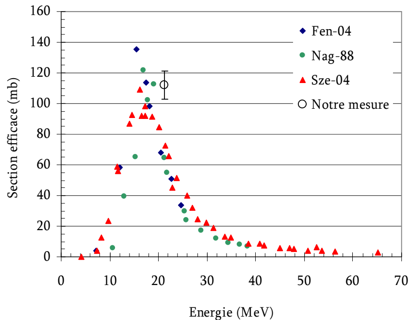
Fig. 28 _ Comparaison de notre mesure de section efficace aux valeurs obtenues dans la littérature pour la réaction ^{59}\text{Co}(\beta\text{He},2n)^{60}\text{Cu} . Les barres d'erreurs ne prennent pas en compte les 10% d'incertitude sur l'épaisseur de la feuille de Co.
