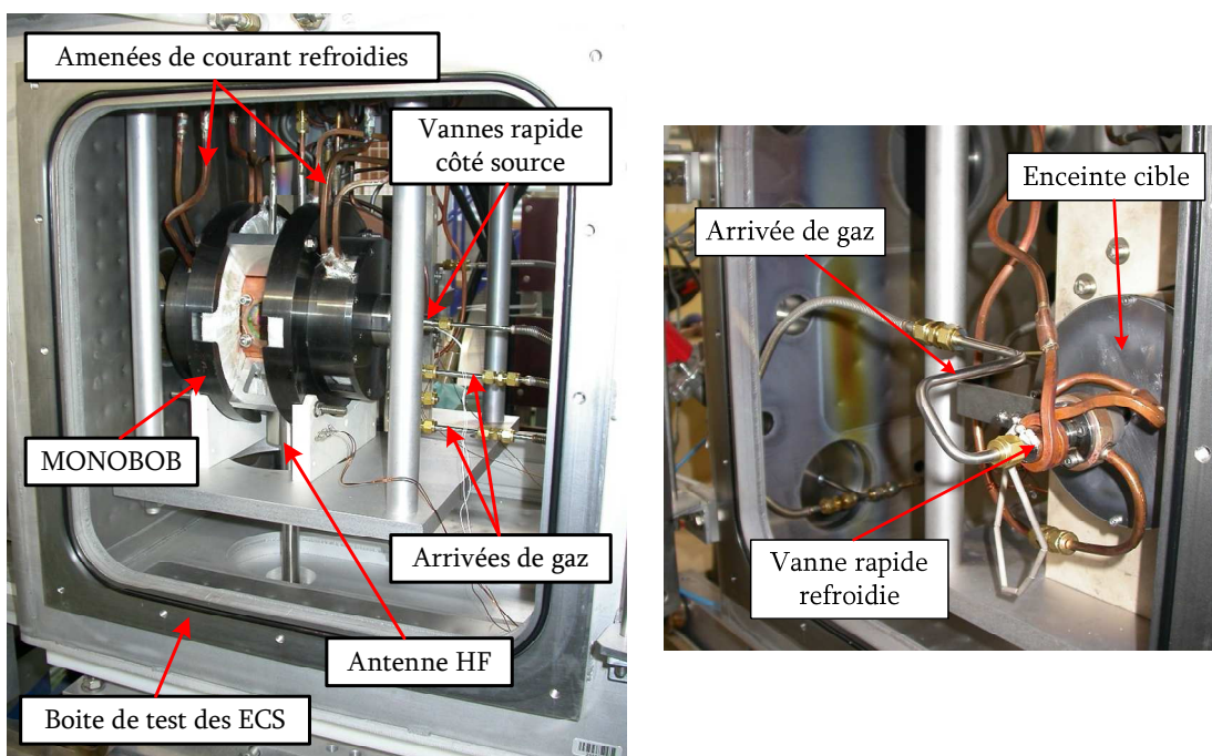
Fig. 91 _ Vue de l'intérieur de la boîte des tests des ECS côté source (photo de gauche) et côté cible (photo de droite).
