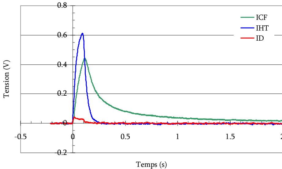
Fig. 71 _ Exemple de mesure réalisée pour le potassium avec le tube en rhénium à une température de 1670 K. En bleu, l'impulsion I_{HT} , en rouge I_D et en vert I_{CF} . Ces données sont brutes ; en ordonnée est donc représentée une tension (intensité au cours de l'impulsion multipliée par la résistance de lecture).
