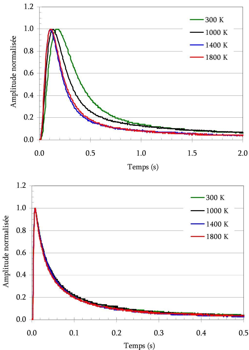
Fig. 97_ Réponses à une impulsion de krypton pour différentes températures de la cible. Sur le graphique du haut, le gaz est injecté côte cible et sur le graphique du bas côté source.
