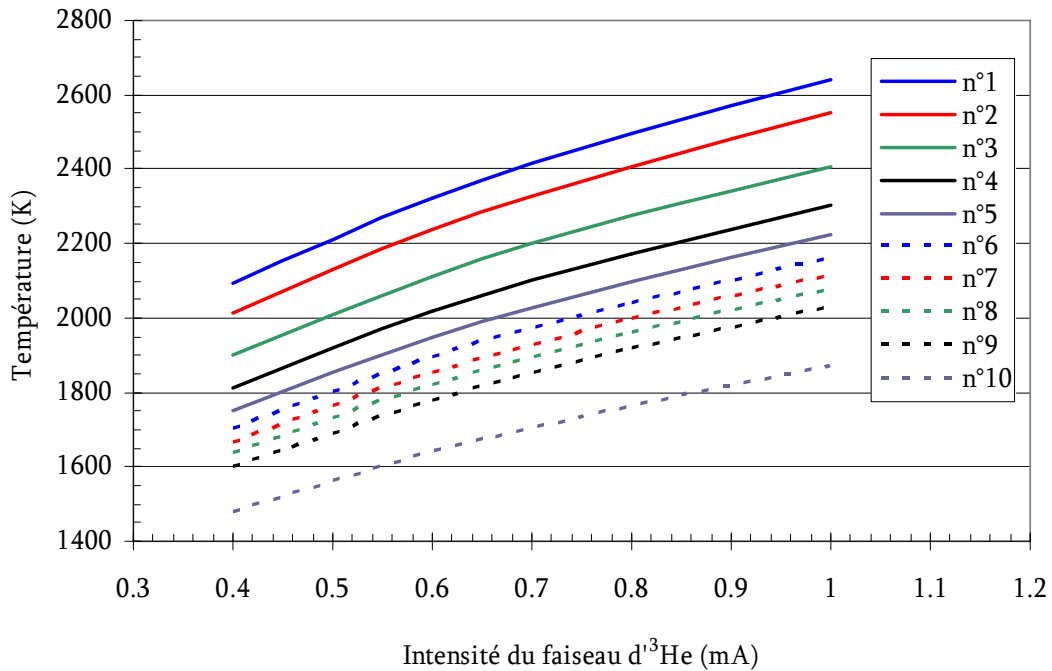
Fig. 40 _ Evolution de la température maximale des disques de l'empilement en fonction de l'intensité du faisceau d 3 He pour le graphite flexible d'épaisseur 125 µm.
