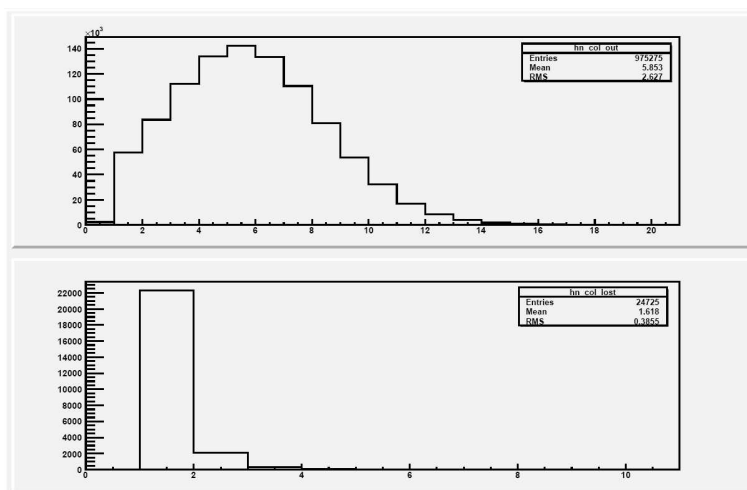
Fig. 128 _ Histogrammes représentant le nombre de collisions effectuées avant que l'alcalin sorte vers la sortie ( hn_col_out ) ou vers l'entrée du tube ( hn_col_lost ).
