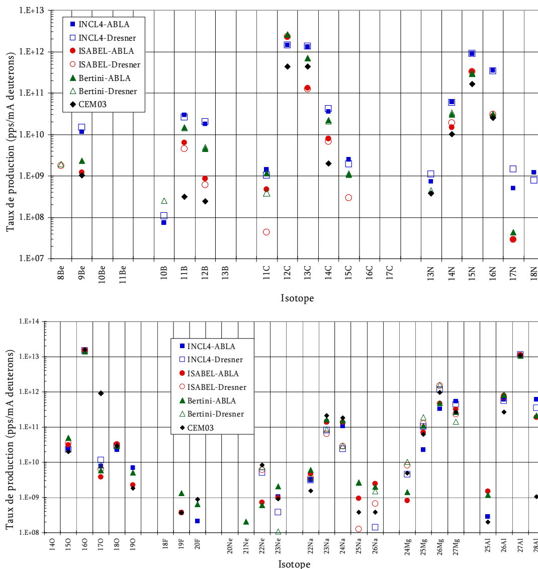
Fig. 9 _ Calcul du taux de production des noyaux résiduels dans la cible d' Al_2O_3 en fonction des modèles.
