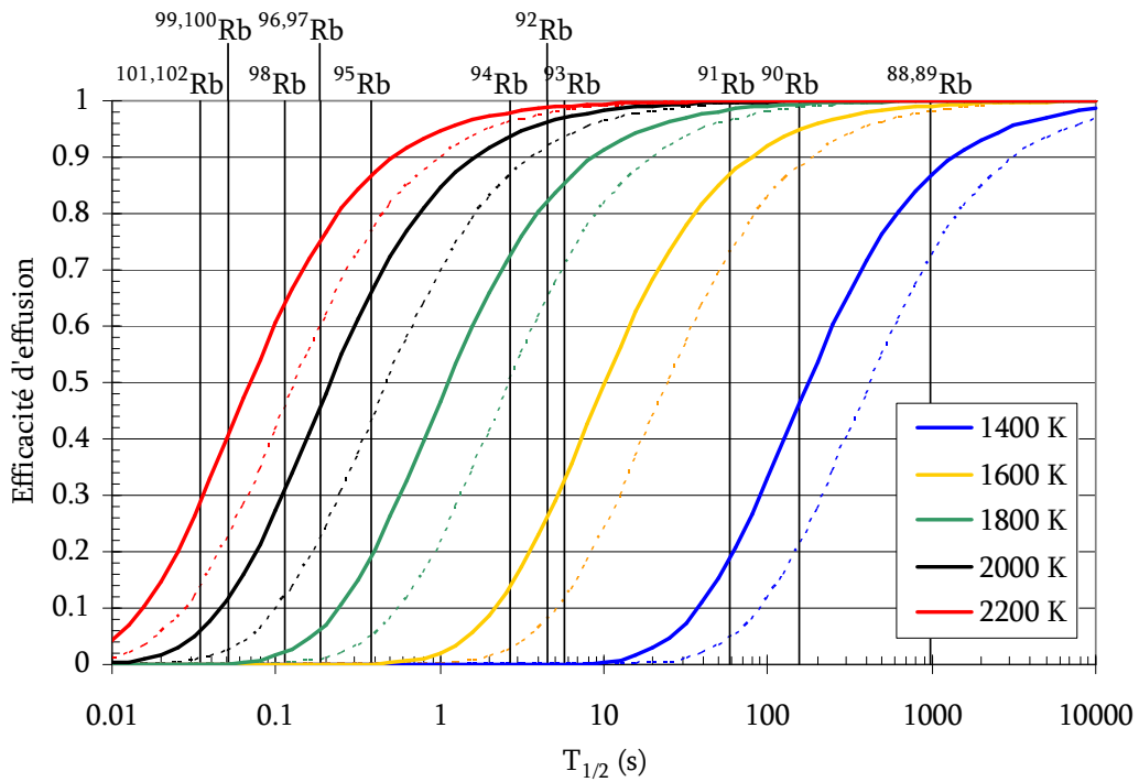
Fig. 109 _ Evolution de l'efficacité d'effusion dans la cible de production pour le rubidium en fonction de la température de la cible et de la durée de vie du noyau.
