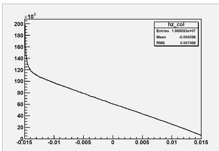
Fig. 120 _ Histogramme représentant le nombre de collisions à la surface du tube en fonction de la position Z selon l'axe du tube (on remarquera que le centre du tube correspond à l'abscisse 0).
