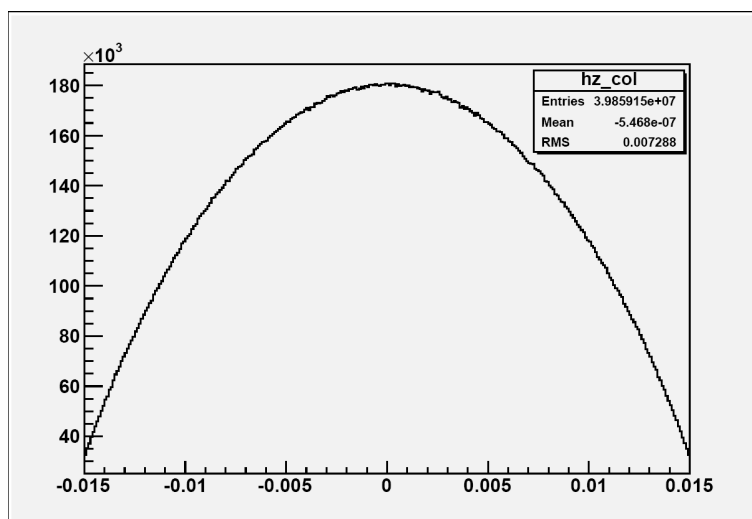
Fig. 123 _ Histogramme représentant le lieu des collisions au cours de la vie de l'alcalin.
