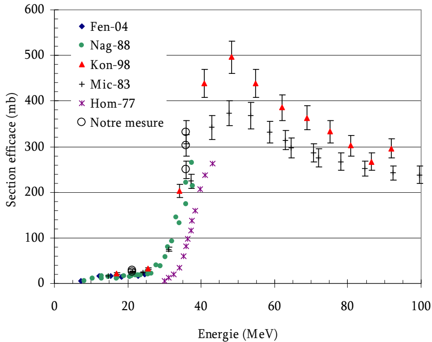
Fig. 32 _ Comparaison de notre mesure de section efficace aux valeurs obtenues dans la littérature pour la réaction ^{59}\text{Co}({}^3\text{He},n){}^{58m+g}\text{Co} . Les barres d'erreurs ne prennent pas en compte les 10% d'incertitude sur l'épaisseur de la feuille de Co.
