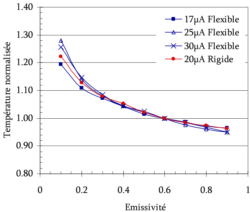
Fig. 115 _ Variation de la température en fonction de l'émissivité du pyromètre 2 (graphique du haut) et du pyromètre 3 (graphique du bas). La température est systématiquement normalisée à la température correspondant à une émissivité de 0,6.
