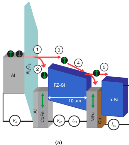
Figure 18 : (a) Le dispositif utilisé pour l'injection et la collection du spin (b) la variation du courant collecté en fonction du champ magnétique appliqué dans le plan
