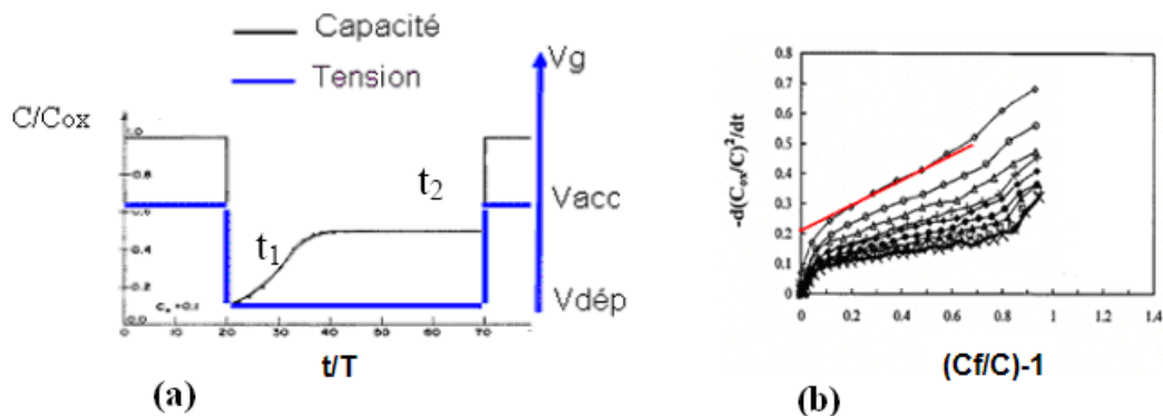
Figure 24 : (a) Principe de la méthode de Zerbst (b) Exemple de tracé de Zerbst pour un ensemble d'échantillons présentant différentes durées de vie [Tan2000]
