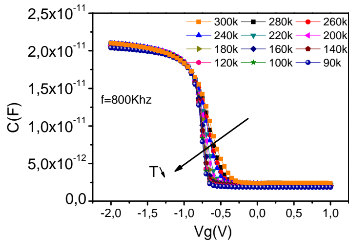
Figure 30: Caractéristiques C(V_g) des structures NiFe/SiO 2 (4 nm)/p-Si avec recuit à la fréquence 800 kHz et à différentes températures
