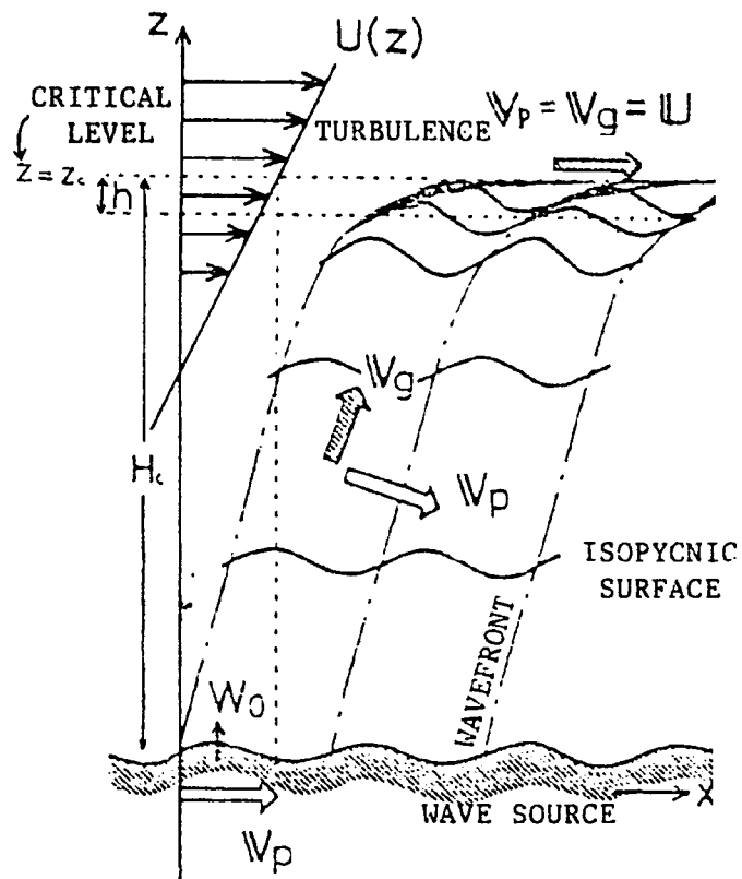
Figure L.6 : Propagation et déferlement au niveau critique z_c des ondes de gravité. V_g et V_p désignent respectivement la vitesse de groupe et la vitesse de phase dont les orientations indiquent une propagation de l'énergie vers le haut [Yamanaka and Tanaka, 1984].
