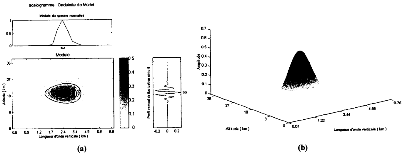
Figure II.11 : Noyau reproduisant de l'ondelette de Morlet au point (a_0, b_0) :
