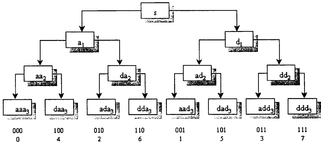
Figure II.27 : Décomposition et reconstruction (progression inverse) en paquets d'ondelettes de codage binaire de Gray (a=0, d=1).
