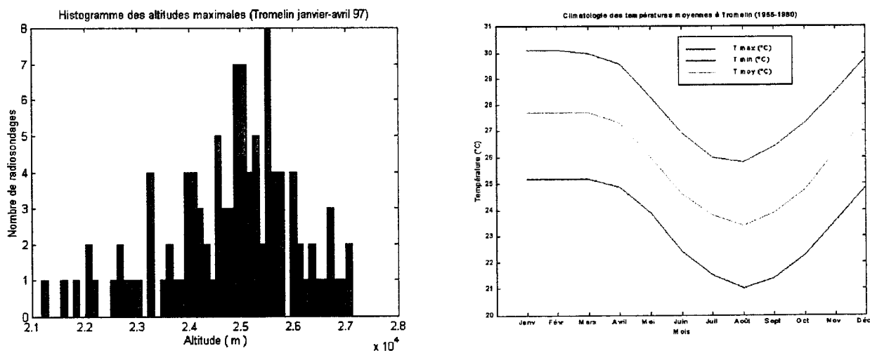
Figure IV.6 : Climatologie des températures moyennes au sol à Tromelin de 1955 à 1980 (données de Météo-France).
