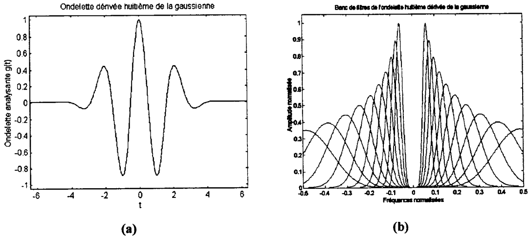
Figure II.7 : a) Ondelette dérivée huitième de la gaussienne, b) Banc de filtres à Q-constant associé.
