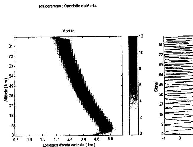
Figure II.21 : Réhaussement d'amplitude du scalogramme du signal de modulation linéaire de longueur d'onde variant entre 2 et 8 km.
