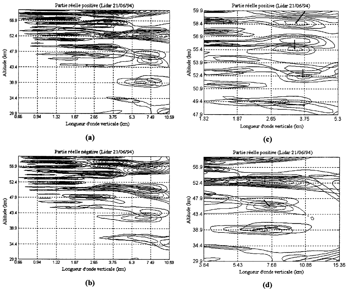
Figure III.35 : Superposition des isocontours de la partie réelle pour la nuit du 21 juin 1994, positive (a) et négative (b) de la transformée en ondelettes par la dérivée huitième de la gaussienne pour deux fichiers successifs n°6 (en noir) et n°9 (en bleu). Zooms sur les modes dominants \lambda_v = 3 km (c) et \lambda_v = 7 km (d). La direction des flèches indique la progression verticale de la phase.
