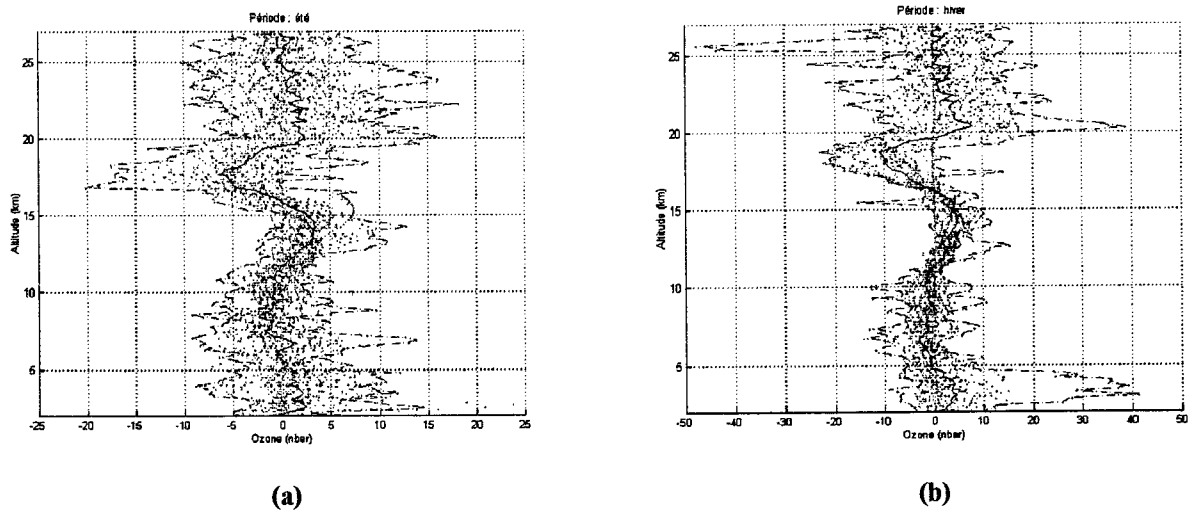
Figure III.15 : Fluctuations de pression partielle d'ozone (en vert), valeurs moyennes et maximales (en rouge et en bleu), extraites des radiosondages de la Réunion : a) été austral b) hiver austral
