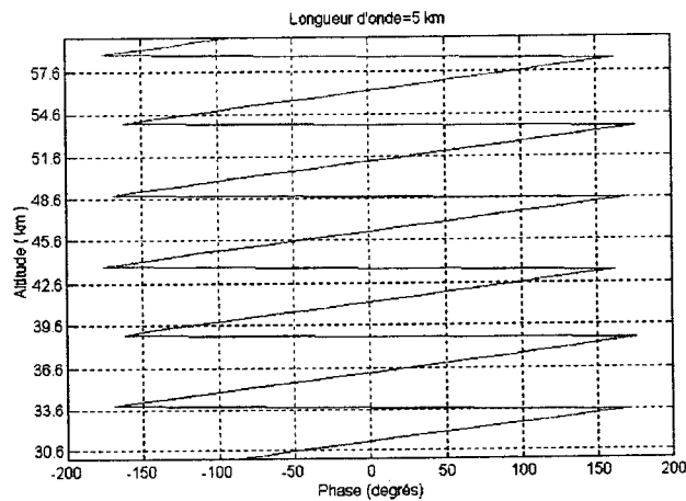
Figure II.13 : Evolution de la phase à la longueur d'onde 5 km.
