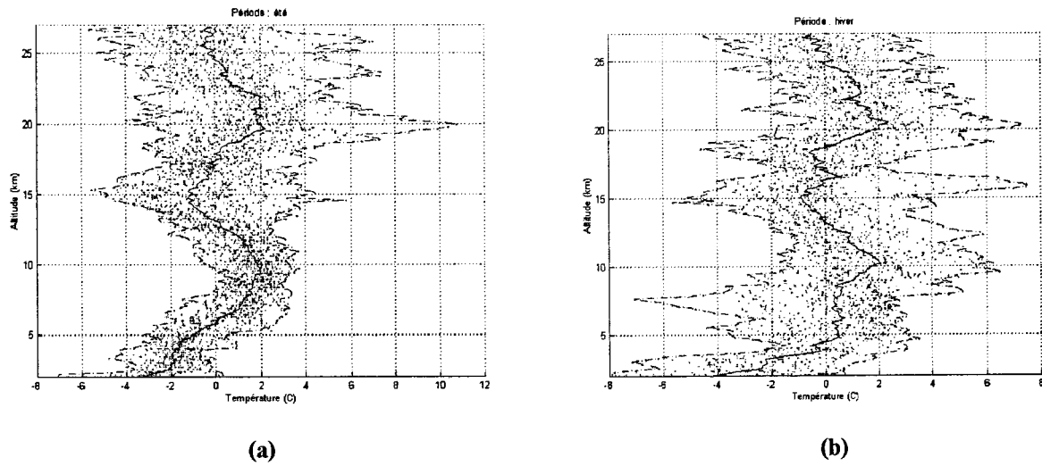
Figure III.14 : Fluctuations de température (en vert), valeurs moyennes et maximales (en rouge et en bleu), extraites des radiosondages de la Réunion : a) été austral b) hiver austral
