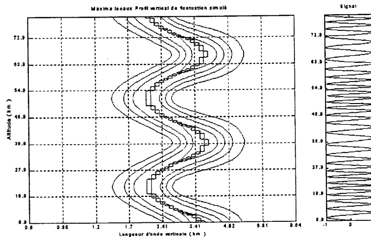
Figure II.14 : Maxima locaux (courbe noire) extraits de la CWT de Morlet d'un signal de modulation sinusoïdale de longueurs d'onde verticales variant entre 2 et 4 km (isocontours bleus).
