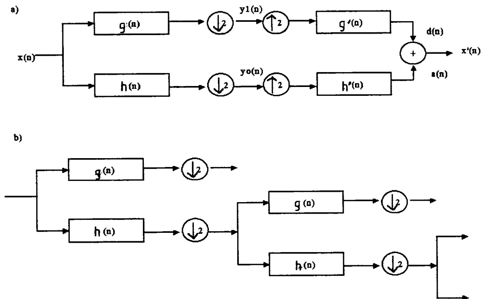
Figure II.22 : Analyse multirésolution et structure pyramidale a) Principe de décomposition et synthèse de l'analyse multirésolution. b) Décomposition pyramidale par la mise en cascade de filtres.
