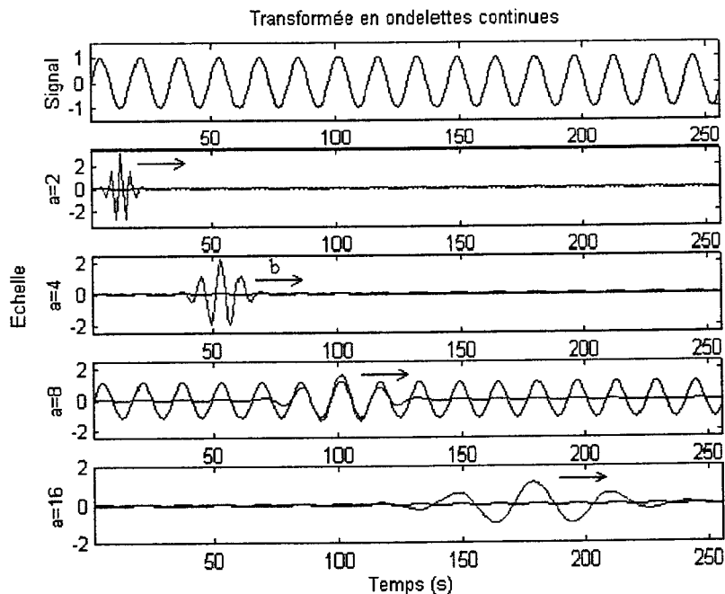
Figure II.1 : Représentation schématique de la transformée en ondelettes continues. Les coefficients en ondelettes (en noir) sont importants à l'échelle a=8 lorsque l'ondelette analysante (en bleu) ressemble aux variations du signal (panneau supérieur).
