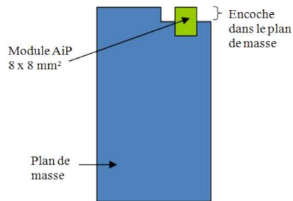
FIG. 4.22 – Module AiP sur PCB de format téléphone portable ( 40 \times 80 \text{ mm}^2 )
