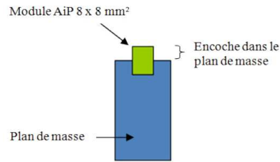
FIG. 4.21 – Module AiP sur PCB de format clé usb standard ( 15 \times 28 \text{ mm}^2 )
