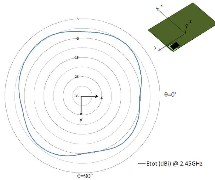
FIG. 5.15 – Gain total (dBi) dans le plan yz mesuré sur le PCB de type téléphone portable
