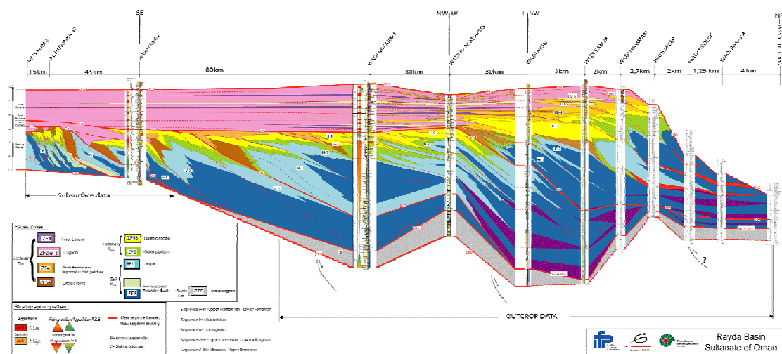
Figure III-9 : Transect régional illustrant le remplissage du bassin de Rayda :les formations Rayda-Salil-Habshhan-Lehswair (Lebec, 2004).
