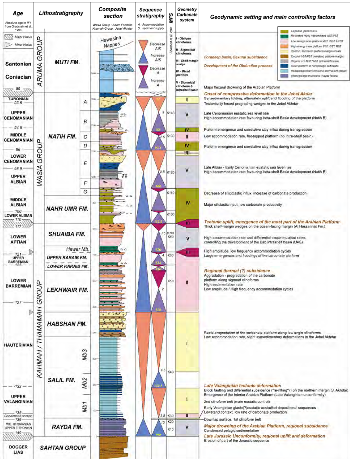
Figure III-6 : Stratigraphie et contexte géodynamique de la plate-forme crétacée en Oman (Razin et al., 2005).
