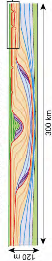
Figure I-3 : Méthodologie générale de l'étude. Une double approche « affleurement-sismique » a été mise en œuvre à deux échelles : régionale et locale.
