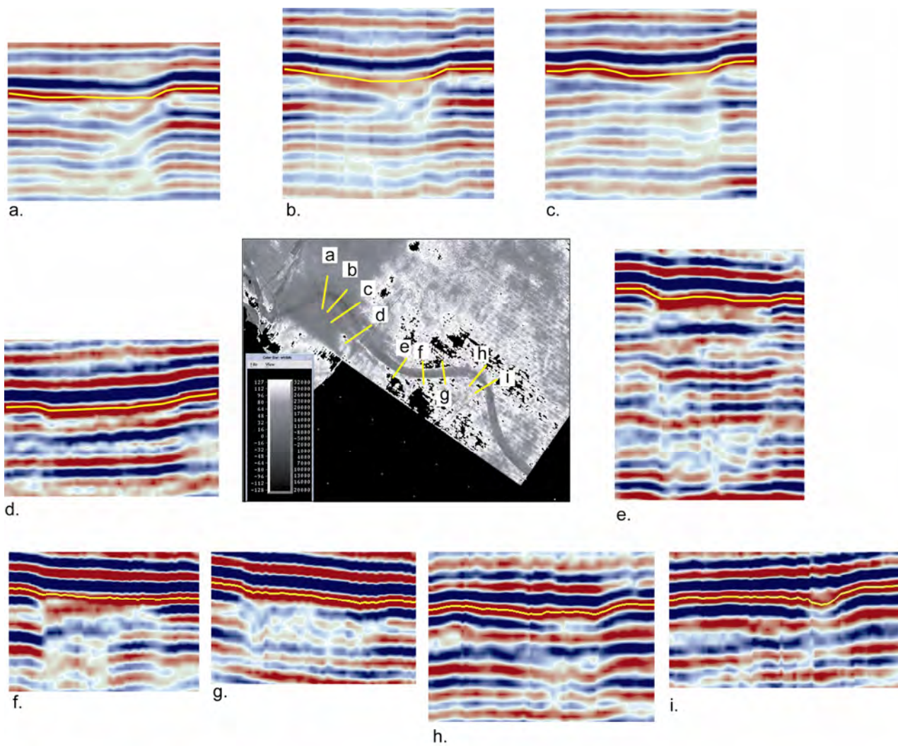
Figure V-16 : Profils sismiques séries au long de l'incision IS2. Ces profils révèlent des hétérogénéités dans le remplissage de cette incision. Le trait jaune souligne la réflexion correspondant au « top Natih E ».
