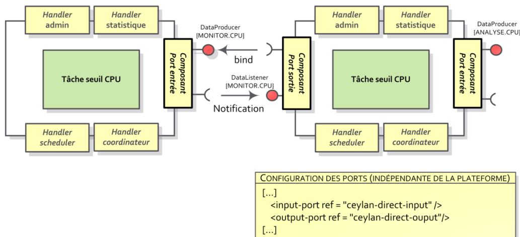
Figure 69 : Implémentation des ports avec communication directe
