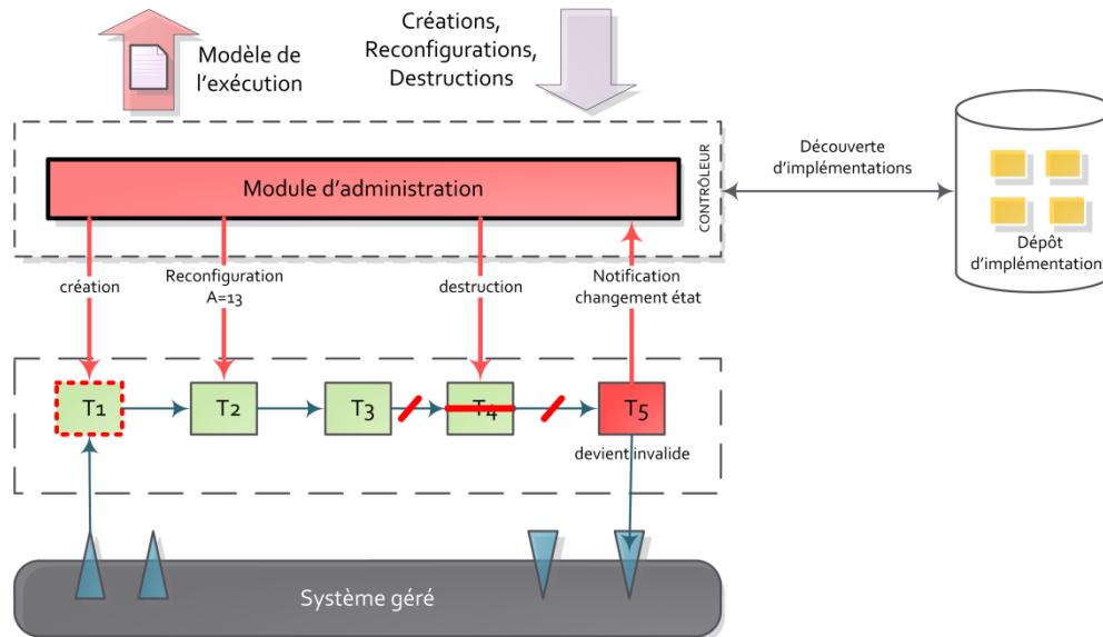
Figure 50 : Module d'administration
