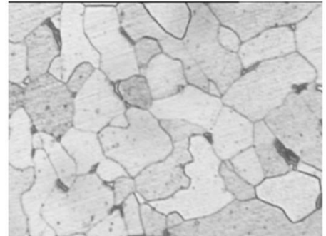
500 μm Fig. 4 Micrographie optique. Structure ferritique
