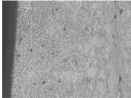
500 μm Fig. 3 Micrographie optique. Structure ferrito-perlitique
