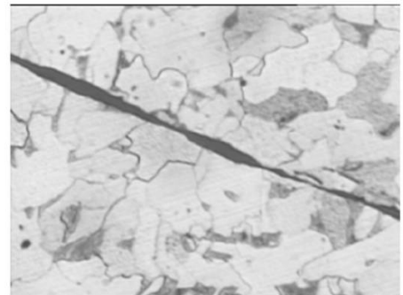
500 μm Fig. 6 Micrographie optique. Structure ferritique, avec scorie monophasée
