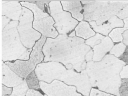
500 μm Fig. 3 Micrographie optique. Structure ferritique
