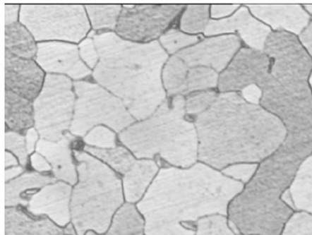
500 μm Fig. 5 Micrographie optique. Structure ferritique
