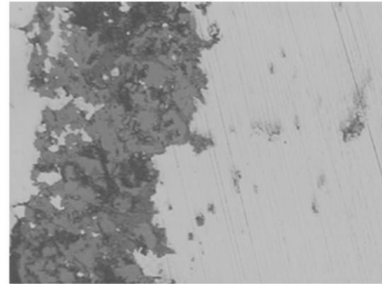
50 μm Fig. 4 Micrographie optique. Scorie avec dendrites de wustite FeO
