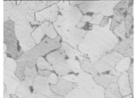
500 μm Fig. 2 Micrographie optique. Structure ferritique avec précipités de cémentite aux joints de grains
