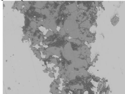
50 μm Fig. 5 Micrographie optique. Scorie avec dendrites de wustite FeO
