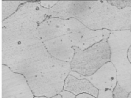
250 μm Fig. 1 Micrographie optique. Structure ferritique
