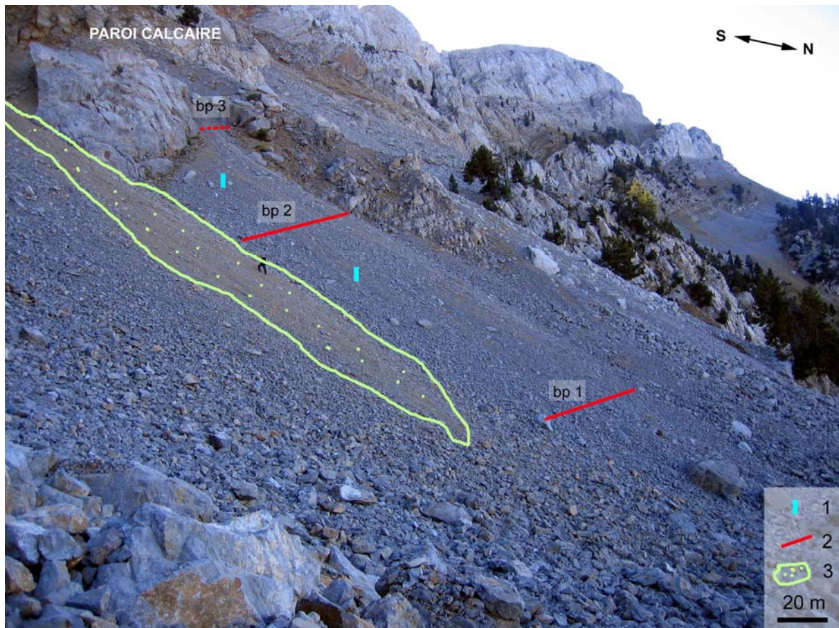
Figure 4.25 – Éboulis instrumenté en Serre de Cadi avec deux bandes peintes (2) continues en zones médiane (bp 2) et distale (bp 1) et cinq cailloux peints alignés en zone proximale (bp 3). Deux colonnes de segments de tubes PVC (1) ont été enfoncées en zone médiane et proximale. Une zone enherbée (3) sépare deux talus d'éboulis.
