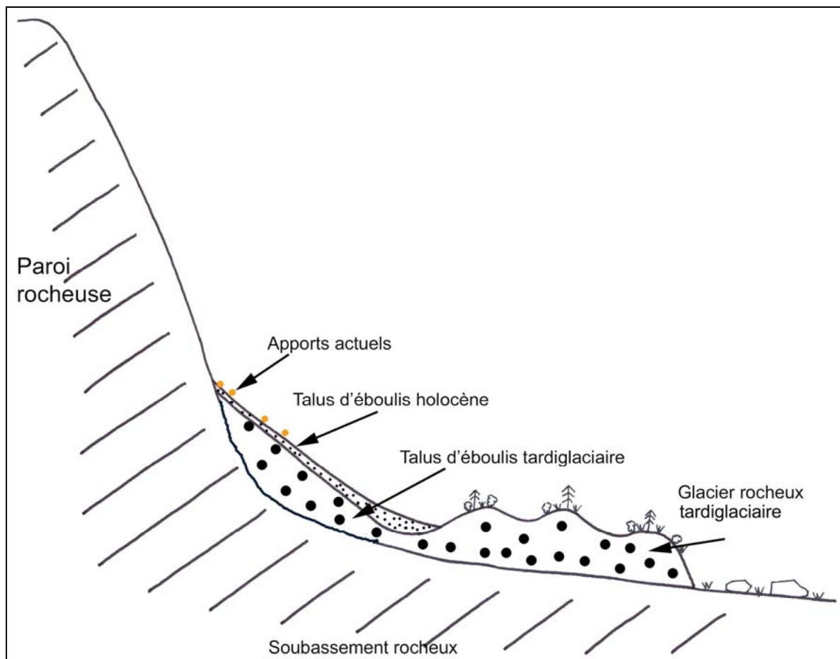
Figure 5.47 – Coupe schématique d'un versant d'ébouilisation avec paroi d'alimentation présentant trois générations de dépôts : un éboulis et un glacier rocheux tardiglaciaire caractérisé par des blocs volumineux, un talus d'éboulis holocène composé de blocs de plus petite taille et les apports actuels, mesurés ponctuellement depuis trois ans et composés de débris dispersés sur la zone proximale de l'éboulis.
