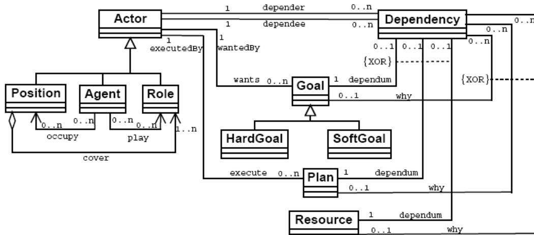
Figure 3-8 : Extrait du méta-modèle d'i* implanté dans Tropos
