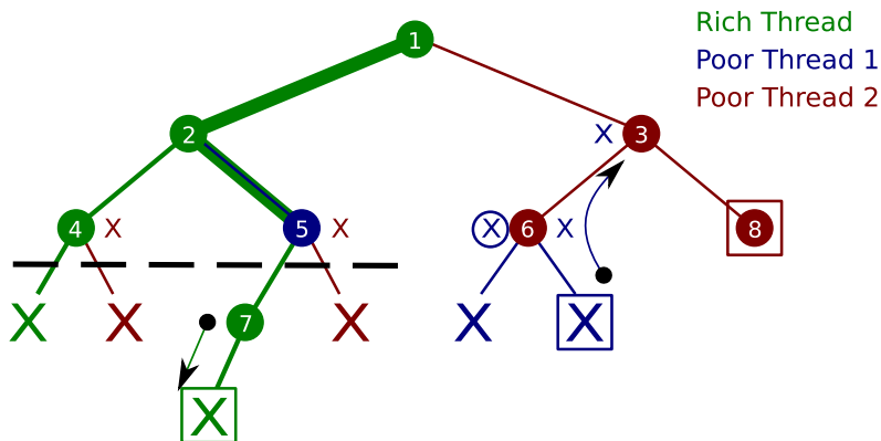
FIG. 5.10 – Exemple MTSS, étape 6
