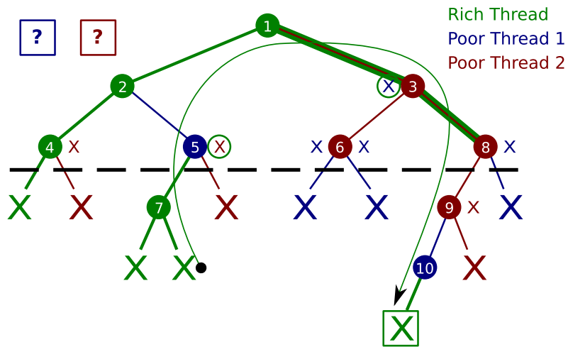
FIG. 5.13 – Exemple MTSS, étape 9
