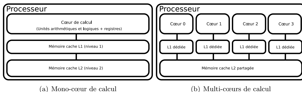
FIG. 2.2 – Schémas de processeurs
