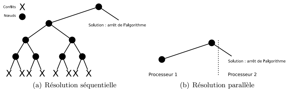
FIG. 3.4 – Accélération super linéaire dans le cas de formules satisfaisables
