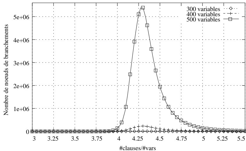
FIG. 1.5 – Pic de difficulté pour le problème 3-SAT
