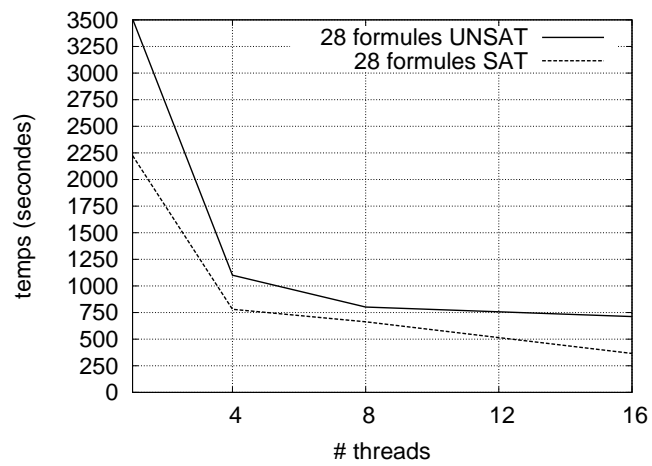
FIG. 6.7 – Performances de MiniSat parallélisé par MTSS
