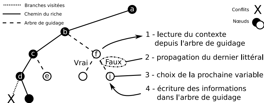
FIG. 5.4 – Étapes du prolongement d'un sous-arbre de guidage
