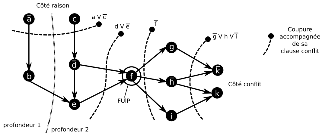
FIG. 1.6 – Graphe d'implication et clauses apprises
