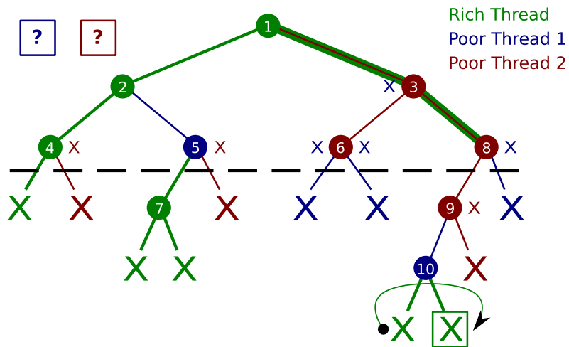
FIG. 5.14 – Exemple MTSS, étape 10
