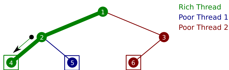
FIG. 5.7 – Exemple MTSS, étape 3
