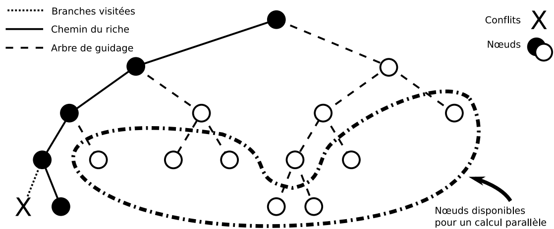
FIG. 4.2 – Exemple d'un arbre de guidage
