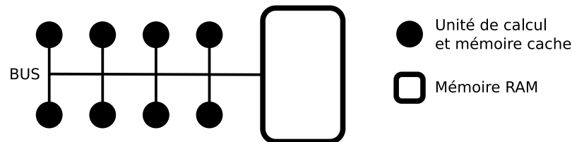
FIG. 2.6 – Schéma d'architecture CC-UMA
