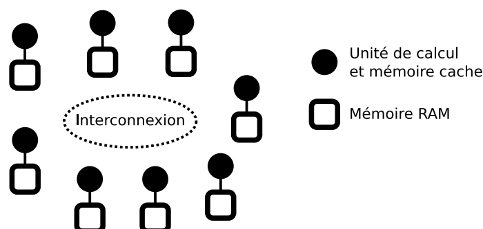
FIG. 2.7 – Schéma d'architecture NUMA
