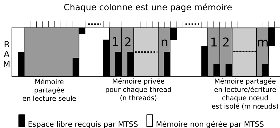
FIG. 5.1 – Cloisonnement des types de mémoire
