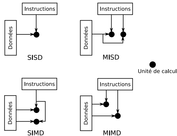
FIG. 2.5 – Taxonomie de la classification de Flynn
