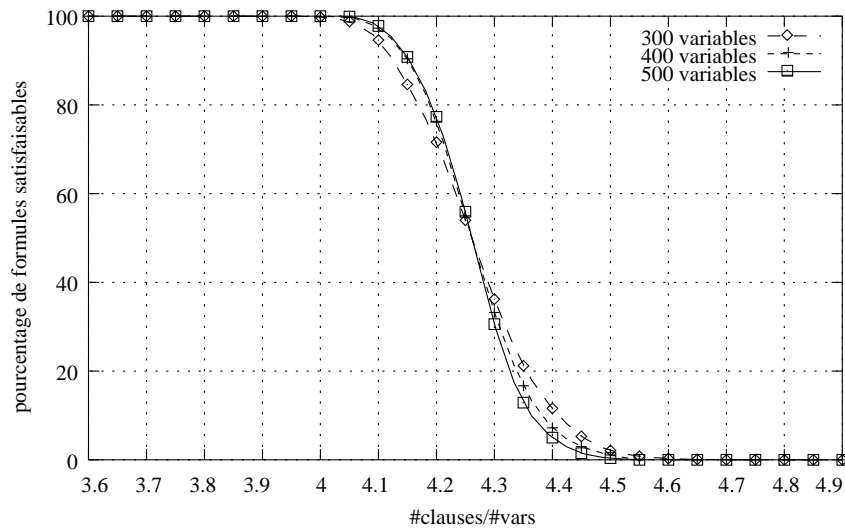
FIG. 1.4 – Transition de phase pour le problème 3-SAT
