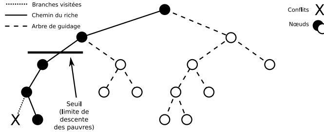
FIG. 5.2 – Principe de seuil
