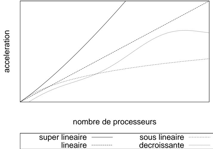
FIG. 2.4 – Exemples d’accélérations possibles, échelle linéaire
