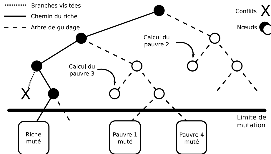
FIG. 5.16 – Parallélisation de solveurs externes
