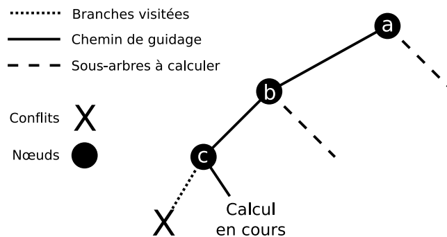
FIG. 3.5 – Chemin de guidage
