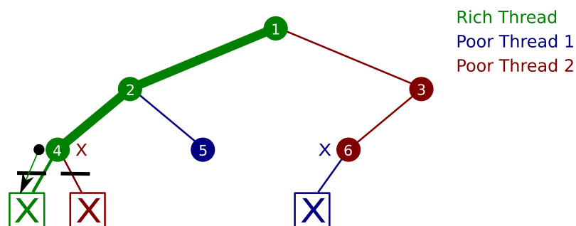
FIG. 5.8 – Exemple MTSS, étape 4
