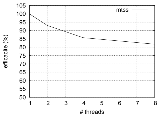
FIG. 6.3 – Efficacité relative de MTSS jusqu'à 8 cœurs
