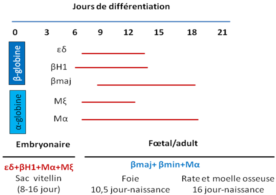
Figure 34 : Expression des gènes de l' α- et de la β-globine au cours de la différenciation des cellules mES.
