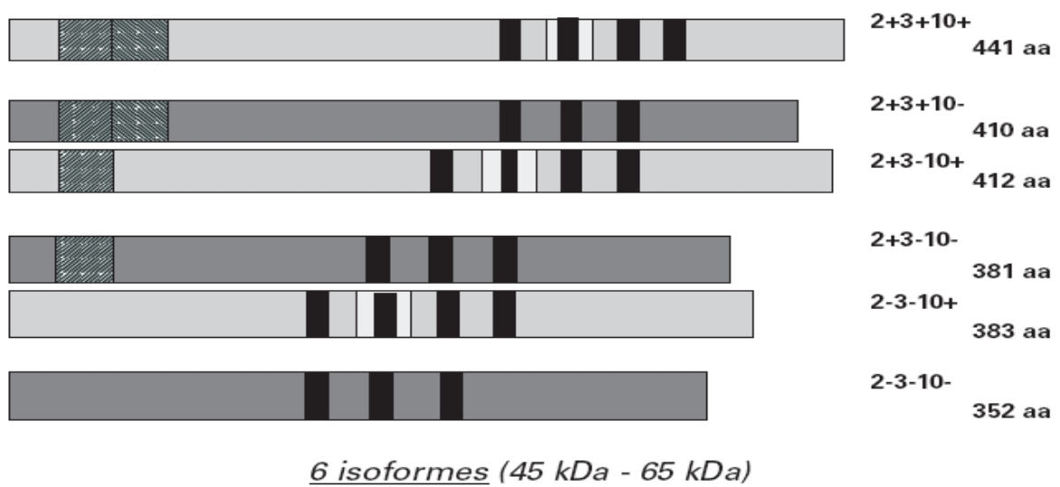
Figure 77 : Les six isoformes de protéines Tau.
