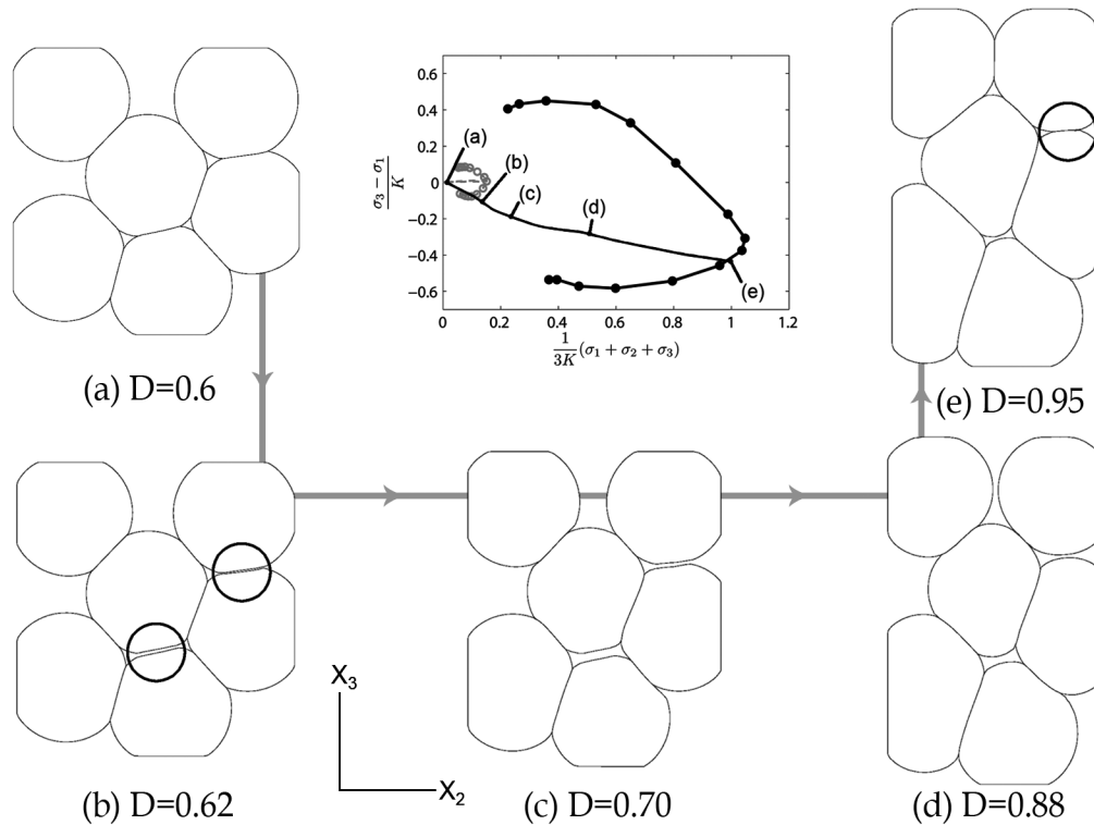
FIGURE 3.23 – La rotation de la surface de charge s’accompagne de la perte de plusieurs contacts dans la structure. Cet exemple correspond au chargement isotrope-déviatoire, avec D_1 = 0,6 . La structure créée par le premier chemin, après décharge à D_1 = 0,6 (a), est modifiée par des pertes de contacts, mises en évidence en (b). La structure évolue ensuite avec le second chemin (c,d), et finalement certains des contacts perdus se reforment (e). Les différents points (a)-(b)-(c)-(d)-(e) sont indiqués dans l’espace des contraintes pour illustrer la position des points de chargement successifs le long du chemin de chargement.
