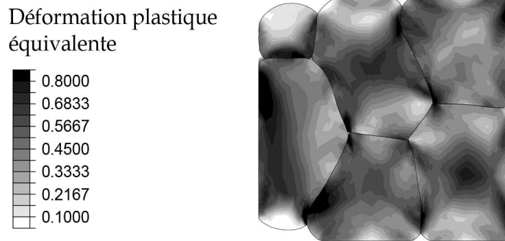
FIGURE 3.21 – Répartition de la déformation plastique équivalente dans une coupe de l'échantillon. Cet exemple correspond au chargement matrice-déviatoire présenté en Figure 3.19, avec une densité relative intermédiaire D_1 = 0,7 et une densité relative finale D_f = 0,95 .
