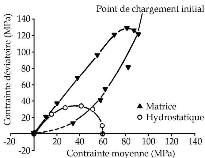
FIGURE 1.6 – Surfaces de charge obtenues par Akisanya et al. (1997) pour une compression hydrostatique et une compression en matrice, avec une poudre de cuivre à grains sphériques. La densité relative correspondant aux deux points de chargement est de 0,8.
