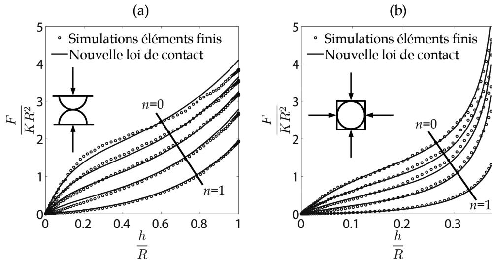
FIGURE 2.11 – Ajustement de la loi de contact définie par l'équation (2.9) pour n = 0, 1; 0,24; 0,5; 1 . (a) Compression simple, (b) Compression isotrope d'une cellule cubique simple.
