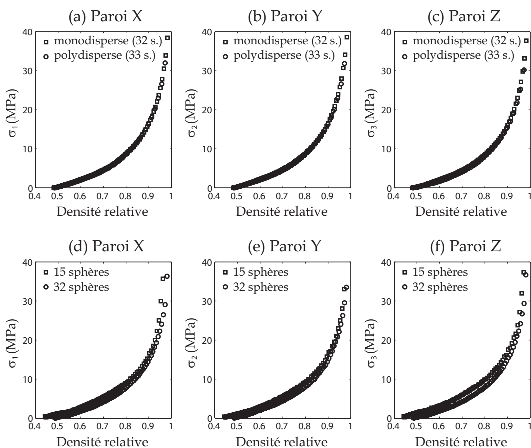
FIGURE 3.3 – Comparaison des échantillons numériques pour la compression isotrope : (a)-(b)-(c) Influence de la polydispersité, (d)-(e)-(f) Comparaison entre les empilement monodisperses de 15 sphères et de 32 sphères.
