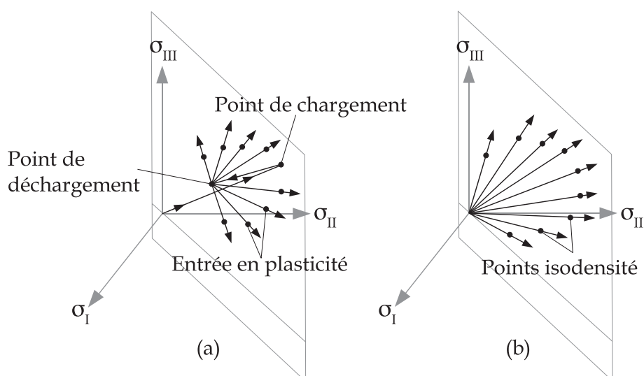
FIGURE 1.5 – Obtention des surfaces de charge. (a) Méthode générale : chargement initial, décharge élastique, recharge dans toutes les directions. (b) Obtention de courbes isodensité.
