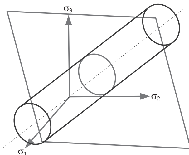
FIGURE 1.1 – Surface de charge de Von Mises.
