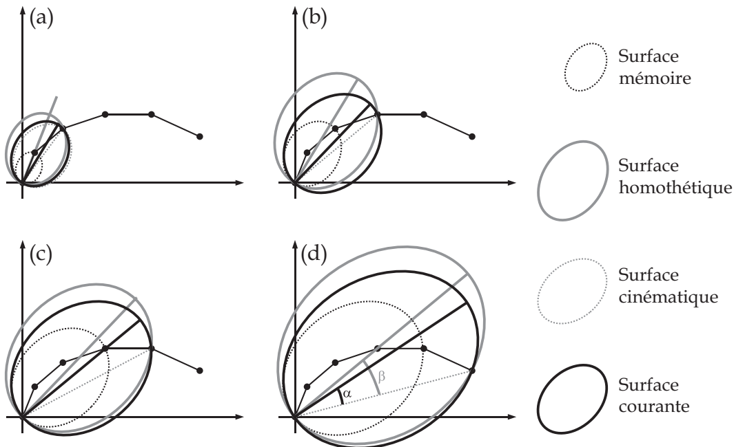
FIGURE 3.27 – Suggestions pour la modélisation de l'évolution des surfaces de charge avec le chemin de chargement.
