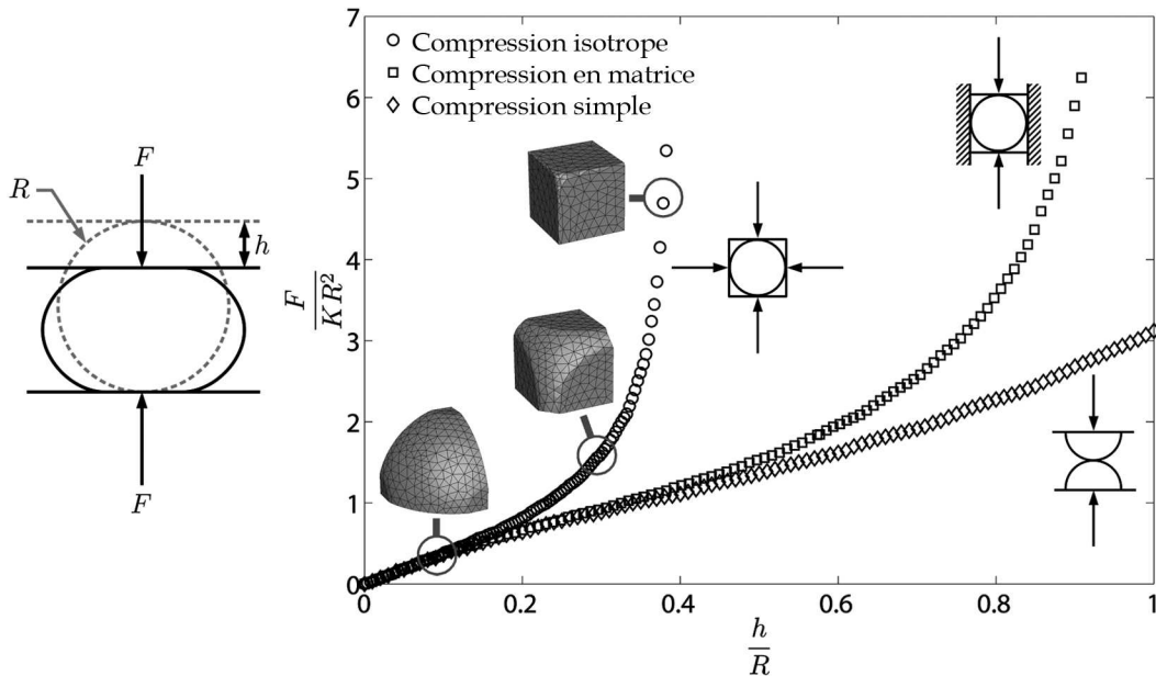
FIGURE 2.6 – Résultats en force-déplacement des simulations par la méthode des éléments finis, pour la compression isotrope et en matrice d'une cellule cubique simple, et la compression simple d'une sphère isolée. Pour la compression isotrope, la géométrie déformée est représentée pour le début de la compression, pour la fin et pour un état intermédiaire. Les paramètres matériau sont donnés par (2.1).
