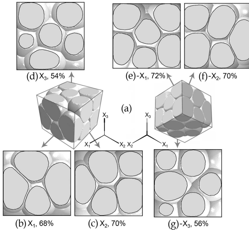
FIGURE 3.20 – Chargement matrice-déviatoire avec la densité relative intermédiaire D_1 = 0,7 et la densité relative finale D_f = 0,95 : proportion de surface en contact avec les parois frontières de l'échantillon. (a) Géométrie déformée 3D de l'échantillon, (b) paroi de normale +X_1 , (c) paroi de normale +X_2 , (d) paroi de normale +X_3 , (e) paroi de normale -X_1 , (f) paroi de normale -X_2 , (g) paroi de normale -X_3 .
