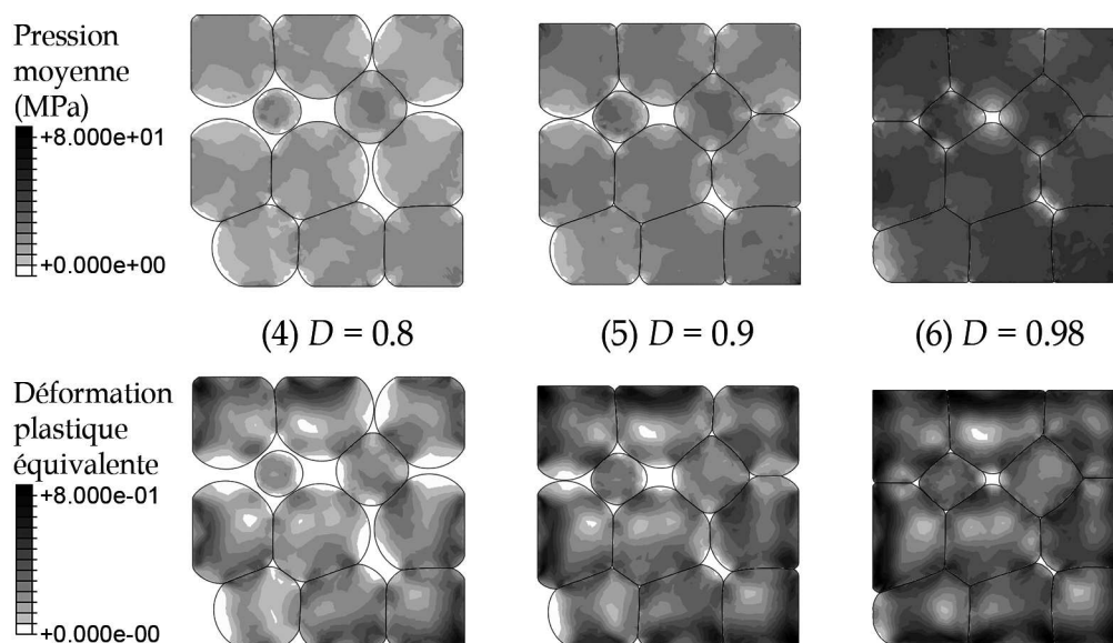
FIGURE 2.30 – Cartes de couleurs représentant l'évolution au cours de la compression, de la pression moyenne et de la déformation plastique équivalente à travers une coupe de l'échantillon. Hautes densités relatives.
