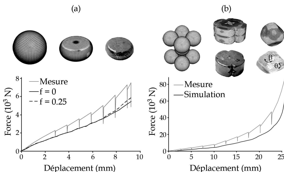
FIGURE 1.17 – Comparaison des résultats des simulations et des données expérimentales de Chen (2008). (a) Compression d’une sphère entre deux plans. Deux simulations sont présentées, avec et sans frottement sphère/plan. (b) Compression de 9 billes dans une matrice cylindrique. Pour la simulation, des coefficients de frottements de 0,25 entre les sphères et la matrice, et 0,1 entre les sphères ont été utilisés. Les angles \beta et \theta qui caractérisent la géométrie de la bille centrale après déformation ont été comparés.
