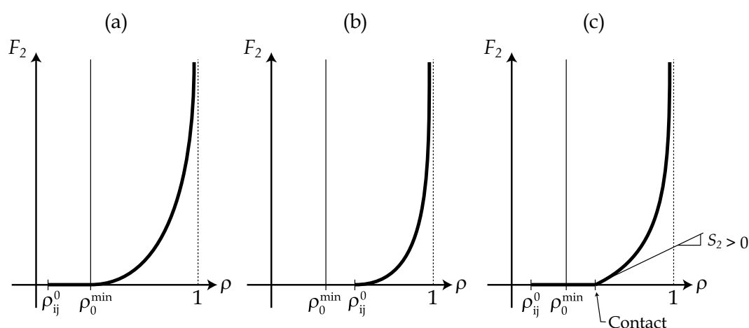
FIGURE 2.10 – Schémas de l'évolution de la force F_2 issue de la raideur S_2 ( F_2 = \int_0^{h/R} S_2 dh/R ) et modélisant la résistance progressive à la compression, en fonction de \rho , pour trois situations : (a) \rho_{ij}^0 < \rho_0^{\min} , (b) \rho_0^{\min} < \rho_{ij}^0 , les sphères sont initialement en contact, (c) \rho_{ij}^0 < \rho_0^{\min} , mais le contact apparaît à une densité relative locale supérieure à \rho_0^{\min} .
