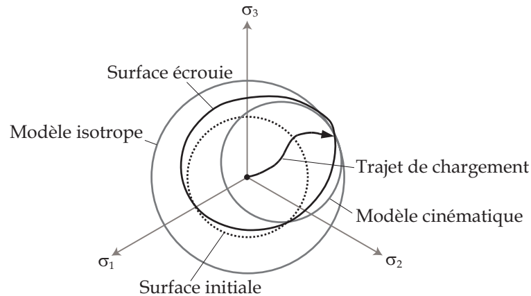
FIGURE 1.2 – Modification par écrouissage de la surface de charge dans le plan déviatoire.
