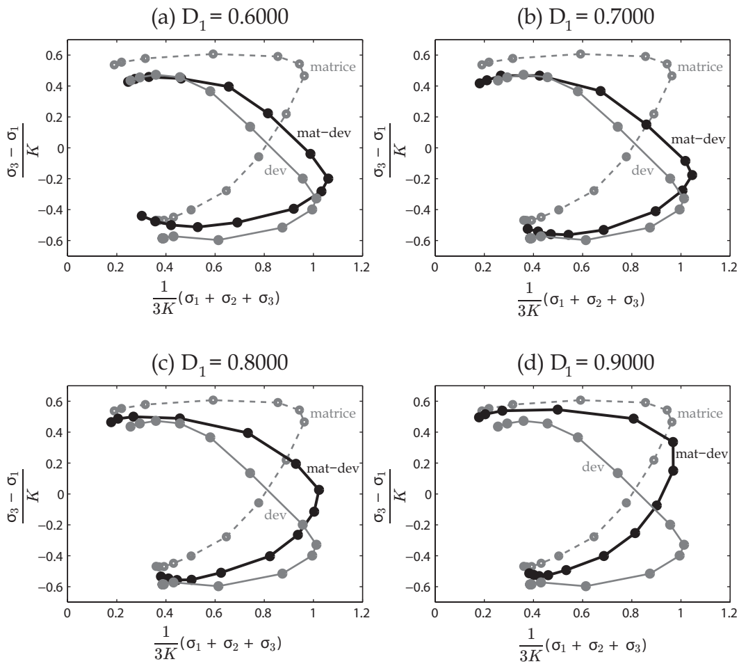
FIGURE 3.16 – Comparaison entre les surfaces de charge correspondant à la densité relative finale D_f = 0,95 , obtenues avec différents chemins de chargement : compression en matrice ('matrice'), chargement matrice-déviatoire ('mat-dev') et monotone déviatoire ('dev'), avec différentes densités relatives intermédiaires D_1 .
