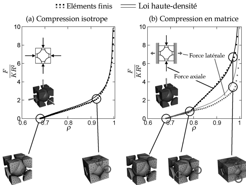
FIGURE 2.17 – Force résultante sur une cellule cubique centrée d'après la simulation par éléments finis et la loi haute-densité. (a) Compression isotrope, (b) Compression en matrice.
