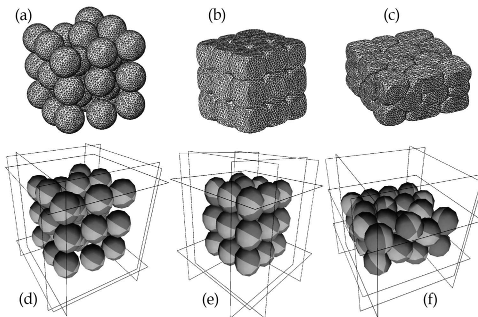
FIGURE 2.20 – Échantillon de 32 sphères monodisperses, modélisé pour la MPFEM (a,b,c) et pour la DEM (d,e,f). (a,d) Échantillon non déformé, (b,e) après compression isotrope, (c,f) après compression en matrice.
