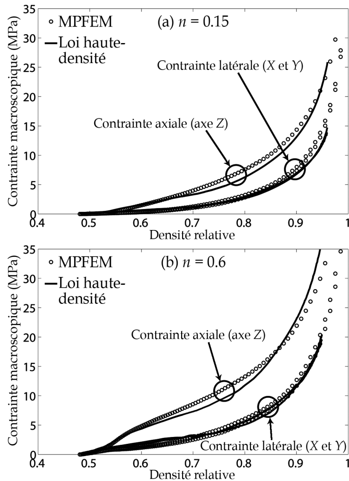
FIGURE 2.26 – Comparaison MPFEM-DEM des contraintes macroscopiques sur l'échantillon de 32 sphères en compression en matrice pour des matériaux différents.
