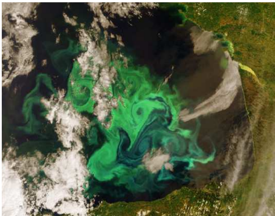
FIG. 3.3 – Dynamique méso et subméso-échelle dans le Golf de Gascogne (06/05/2005) composition en fausse couleur (rgb) à partir des données du capteur MERIS (ENVISAT, ESA), la domaine montrée mesure environ 400km de côté.
