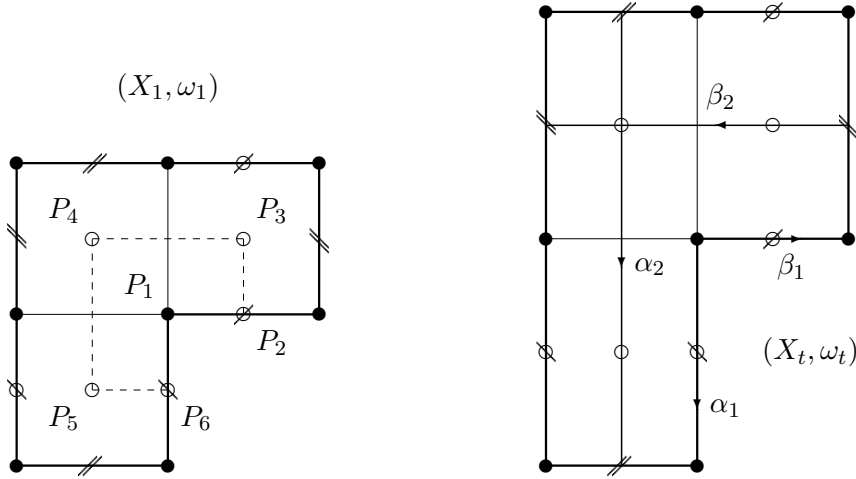
FIGURE 4.3 – La surface à trois carrés : base symplectique et déformation de Teichmüller.
