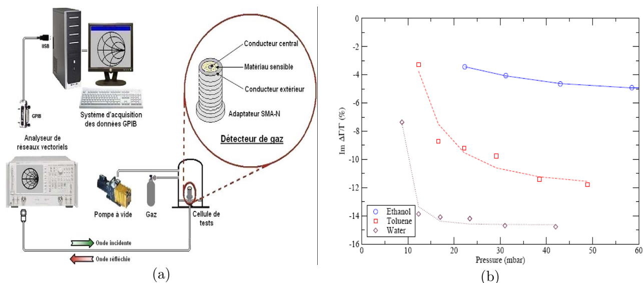
Figure 9. Développement d'un nouveau capteur de gaz basé sur la détection à large bande micro-onde [66], (a) Schéma du montage expérimental utilisé pour tester le capteur de gaz micro-onde ; (b) Evolution de la partie imaginaire de \Delta\Gamma (coefficient de réflexion) en fonction de différentes pressions de vapeur saturante d'éthanol, de toluène et d'eau à 2 GHz ( \text{SrTiO}_3 ) [49].
