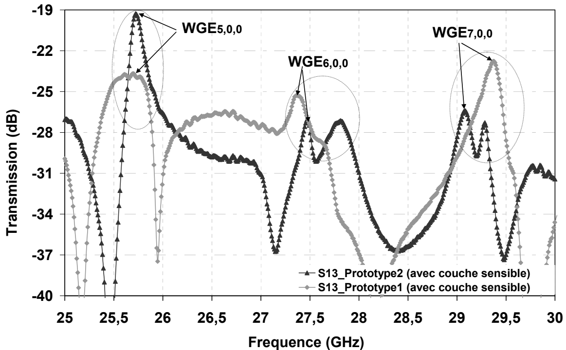
Figure 6. Comparaison du coefficient de transmission de deux prototypes avec couche sensible
