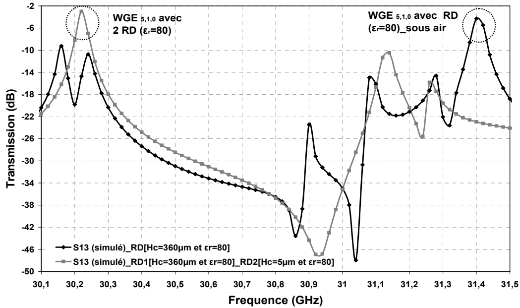
Figure 12. Comparaison du coefficient de transmission entre capteur avec un RD d'épaisseur 360 \mu\text{m} et un capteur avec un RD d'épaisseur 365 \mu\text{m}
