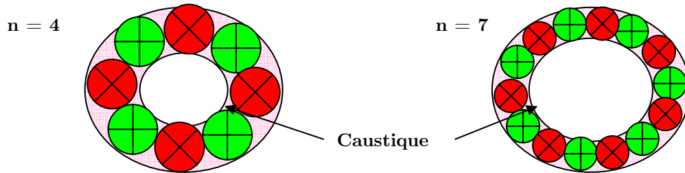
Figure 4. Influence du nombre azimutal sur le rayon de caustique
