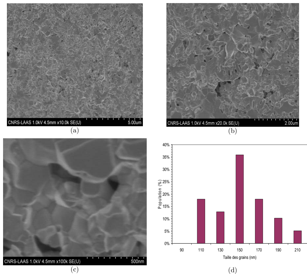
Figure 1. Image MEB de la pastille à 18% de porosité à différentes échelles (a) 5µm, (b) 2µm, (c) 500nm et (d) : distribution en taille des grains de TiO_2
