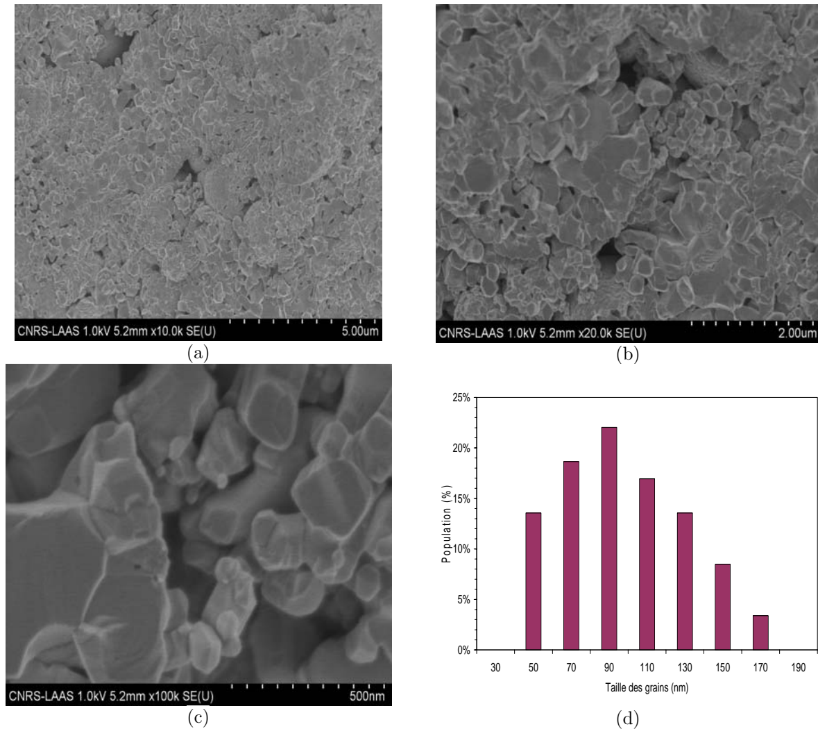
Figure 26. Images MEB de la pastille (échantillon AI127) à 22% de porosité à différentes échelles (a) 5 μm, (b) 2 μm, (c) 500 nm et (d) : distribution en taille des grains de \text{TiO}_2
