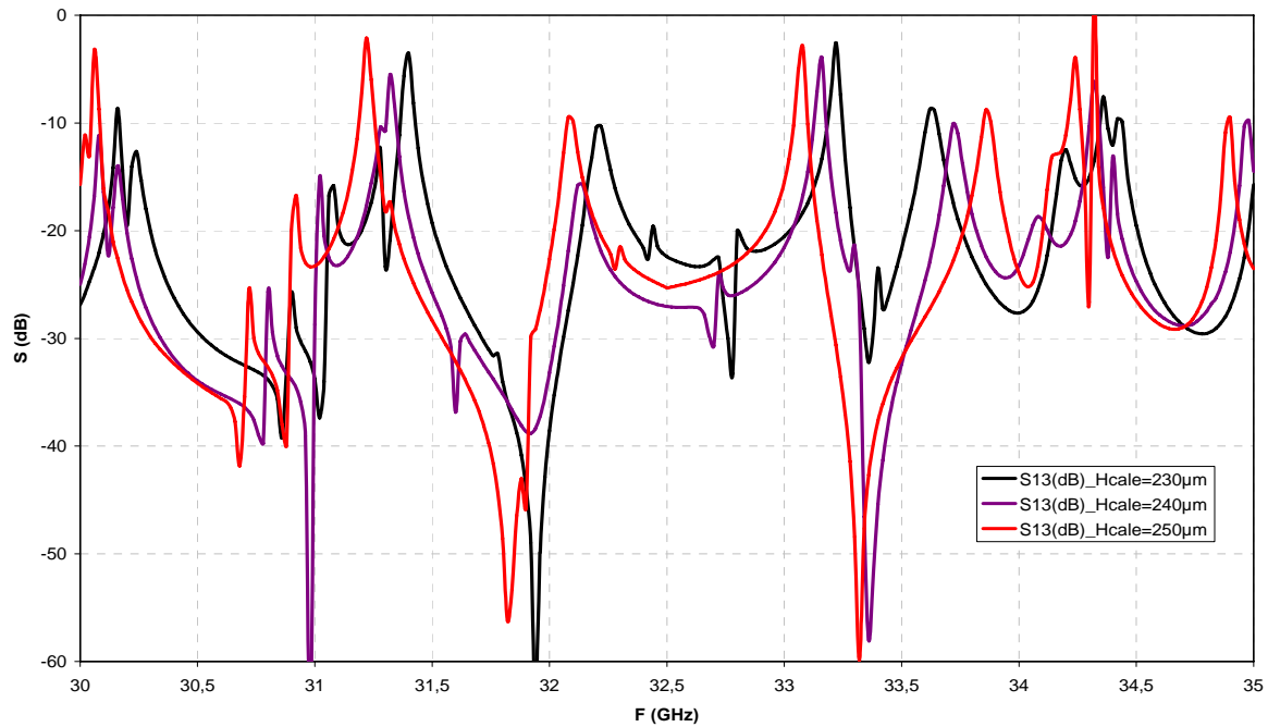
Figure 21. Coefficient de transmission dans la bande de fréquence : [30,35GHz] avec une variation de l'épaisseur de la cale H_{cale,e} entre 230µm à 250µm.
