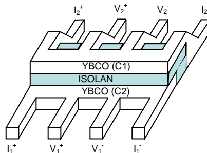
Fig III.89 : Représentation schématique du motif gravé (configuration superposée)
