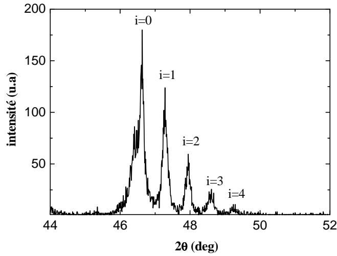
Fig II.37 : Diagramme expérimental de diffraction RX ( \theta - 2\theta ) d'un superréseau [YBCO/LAO] 10 .
