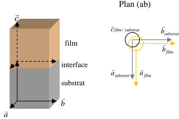
Fig II.3 : Epitaxie directe entre le substrat le film.
