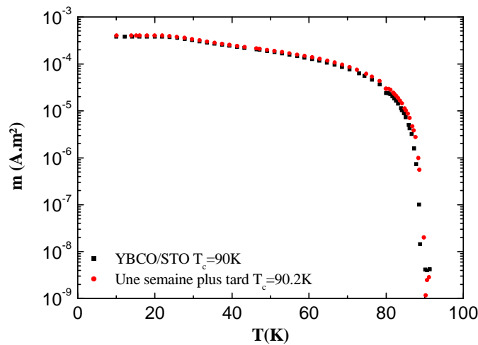
Fig II.61 : Mesure magnétique de deux films fabriqués dans des conditions identiques.
