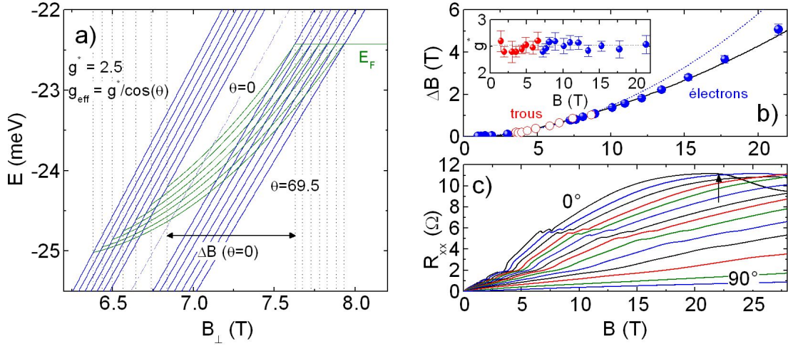
Fig. 4: a) Energie de la bande de Landau N = 1 (voir Fig. 3 b)) en fonction du champ magnétique perpendiculaire au plan, B_{\perp} , et de l'angle \theta . L'angle \theta permet de modifier l'énergie de Zeeman g^* \mu_B B avec g^* = 2.5 . Le mouvement de l'énergie de Fermi a été calculé pour \theta = 0 d'une manière auto-cohérente en supposant que la somme des concentrations des électrons et des trous est constante. Pour \theta > 0 , l'énergie de Fermi a été extrapolée aux champs magnétiques inférieurs. b) Séparation des motifs \Delta B en fonction du champ magnétique. La ligne pointillée est attendu théoriquement si l'énergie de Fermi est une constante. La ligne continue correspond aux calculs montrés en a). Encart : Facteur de Landé pour chaque angle calculé dans le modèle SWM en utilisant les données \Delta B(B) . g^* = 2.5 \pm 0.1 . c) R_{xx} en fonction du champ magnétique pour des angles différents ( T \approx 300 mK). Le champ magnétique auquel l'onde de densité de charge apparaît est repéré par une flèche ( \theta = 0 ).
