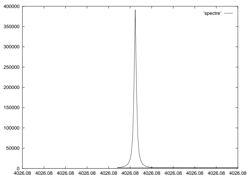
Figure 2.18. Détail d'une raie
