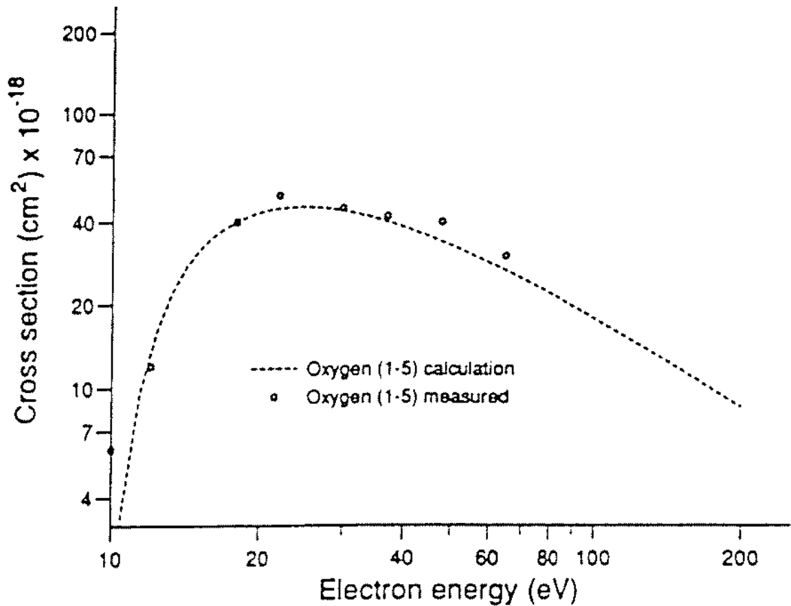
Figure 2.3. Section efficace d'excitation électronique par impact d'électron pour la transition O(2p^4(^3P)) \rightarrow O(3s(^3S)) : travaux de Gallis et al. [16]
