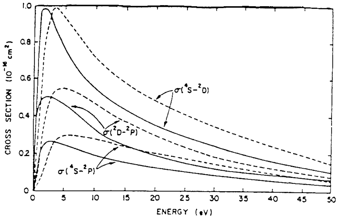
Figure 2.6. Variation de la section efficace inélastique avec l'énergie de l'électron incident pour l'atome d'azote : travaux de Henry et al. [28] (courbe solide) et Smith et al. [27] (courbe en pointillés)
