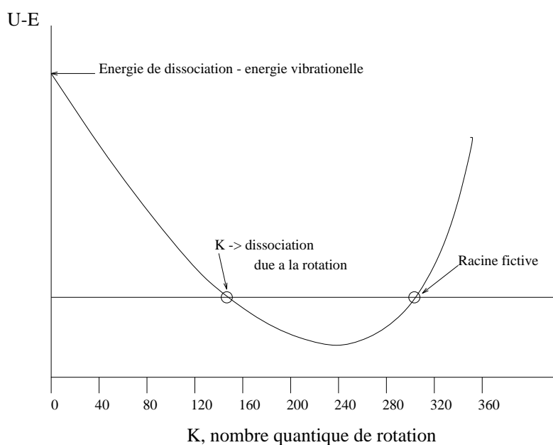
Figure F.2. Détermination de K pour la dissociation
