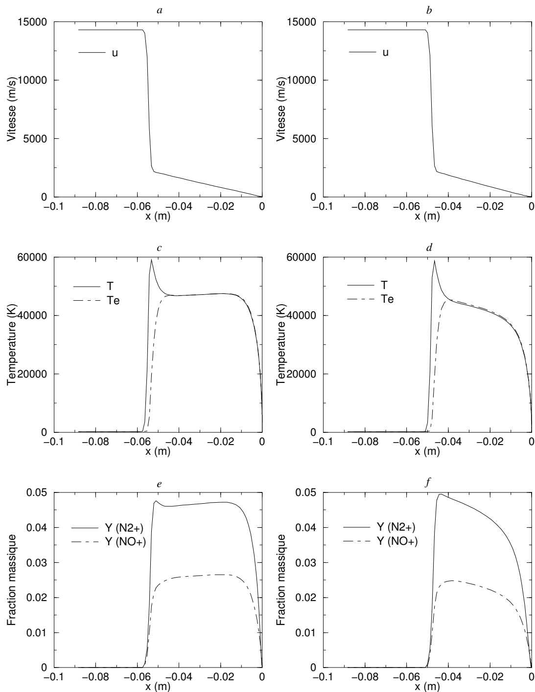
Figure 5.8. Calcul en déséquilibre thermo-chimique sans rayonnement (figures a,c,e ) et avec rayonnement (figures b,d,f ) :
