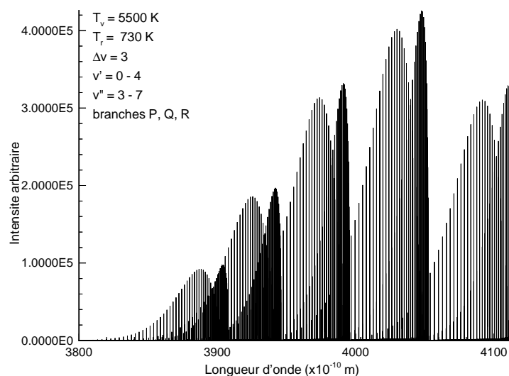
Figure 2.17. Transition radiative N_2(C^3\Pi_u) \longrightarrow N_2(B^3\Pi_g) pour \Delta v = 3 avec T_v = 5500K , et T_r = 730K
