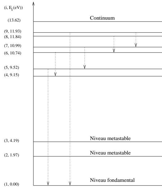
Figure 2.11. Premiers niveaux d'énergie de l'atome d'oxygène
