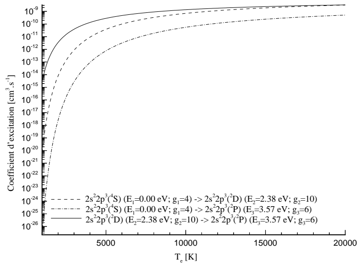
Figure 2.8. Coefficients d'excitation des états métastables par impact électronique en fonction de la température des électrons pour l'atome d'azote
