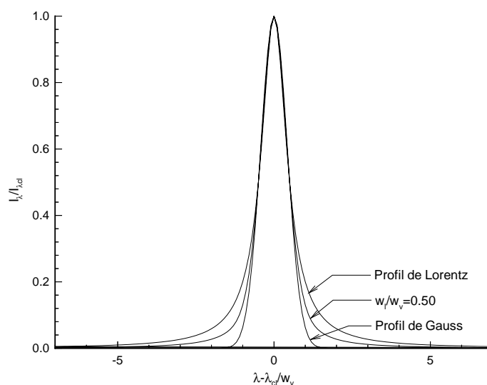
Figure 2.16. Profil de Voigt
