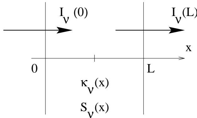
Figure 4.3. Transfert radiatif monodimensionnel pour un milieu non homogène
