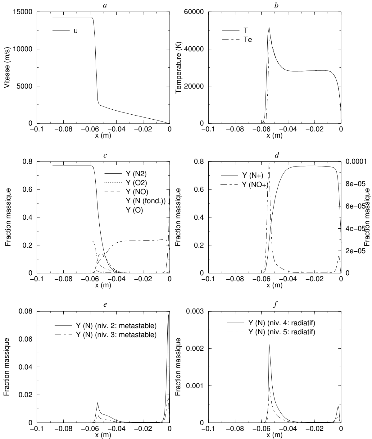
Figure 3.1. Calcul en déséquilibre thermo-chimique sans rayonnement : Profils de vitesse (a), de température (b), de fraction massique (c,d,e,f) le long de la ligne d'arrêt (cas avec N^+ )
