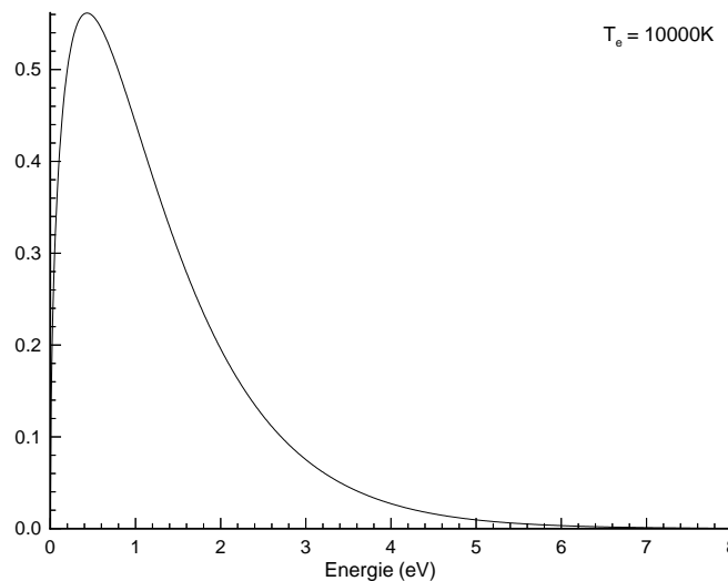
Figure 2.1. Maxwellienne des électrons à la température T_e = 10000K
