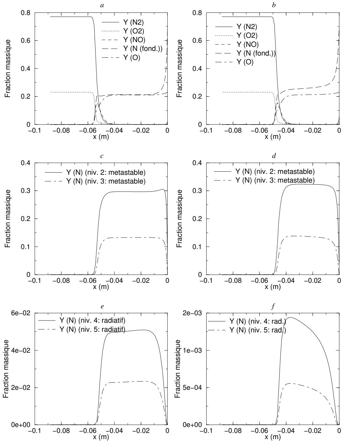
Figure 5.9. Calcul en déséquilibre thermo-chimique sans rayonnement (figures a,c,e) et avec rayonnement (figures b,d,f) : Profils de fraction massique (a,b,c,d,e,f) le long de la ligne d'arrêt (cas avec N_2^+ )
