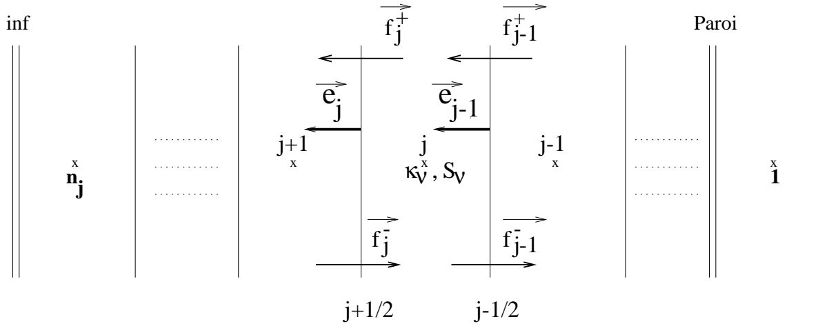
Figure 4.4. Maillage monodimensionnel pour le calcul aérodynamique et du transfert radiatif
