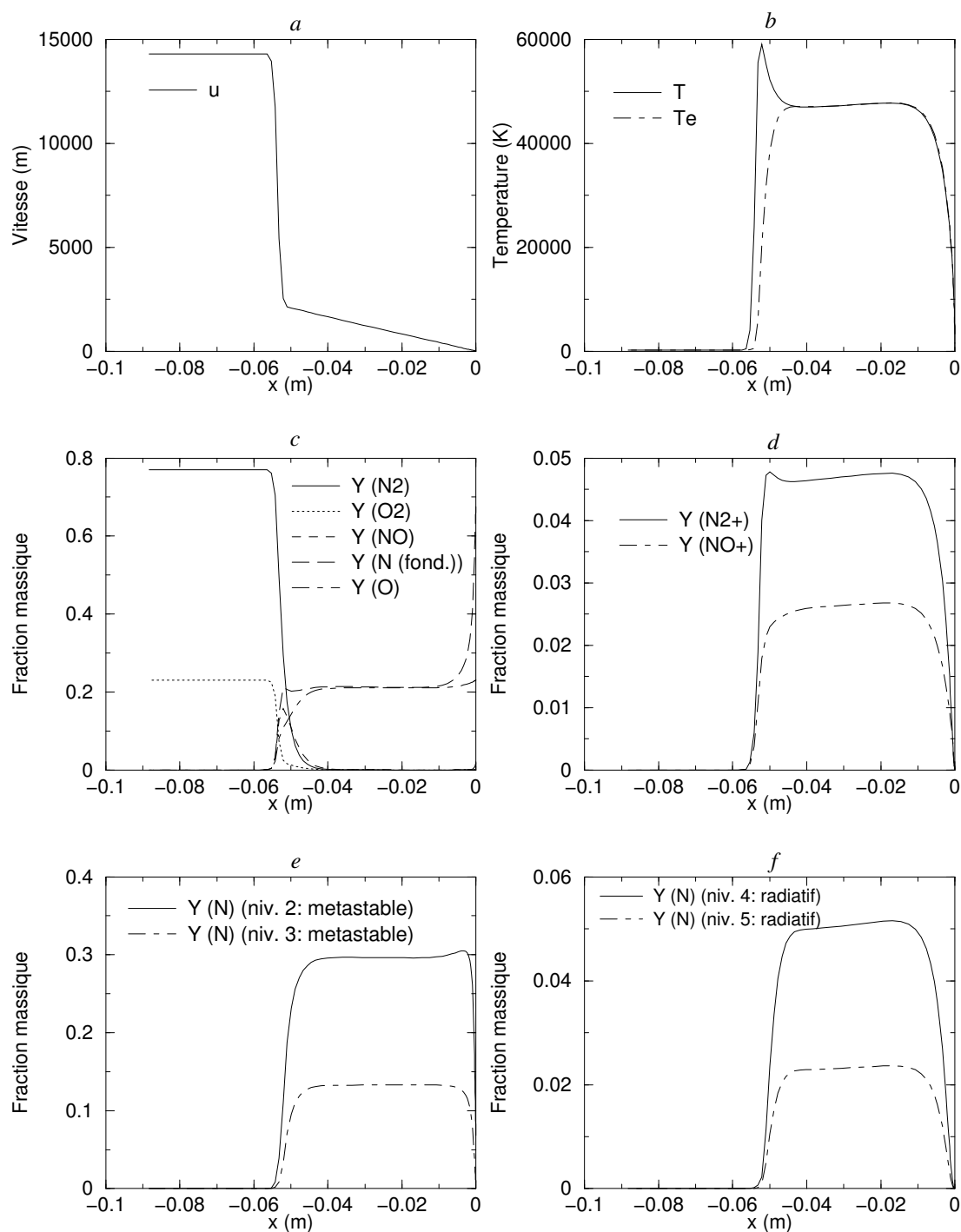
Figure 3.2. Calcul en déséquilibre thermo-chimique sans rayonnement : Profils de vitesse (a), de température (b), de fraction massique (c,d,e,f) le long de la ligne d'arrêt (cas avec N_2^+ )
