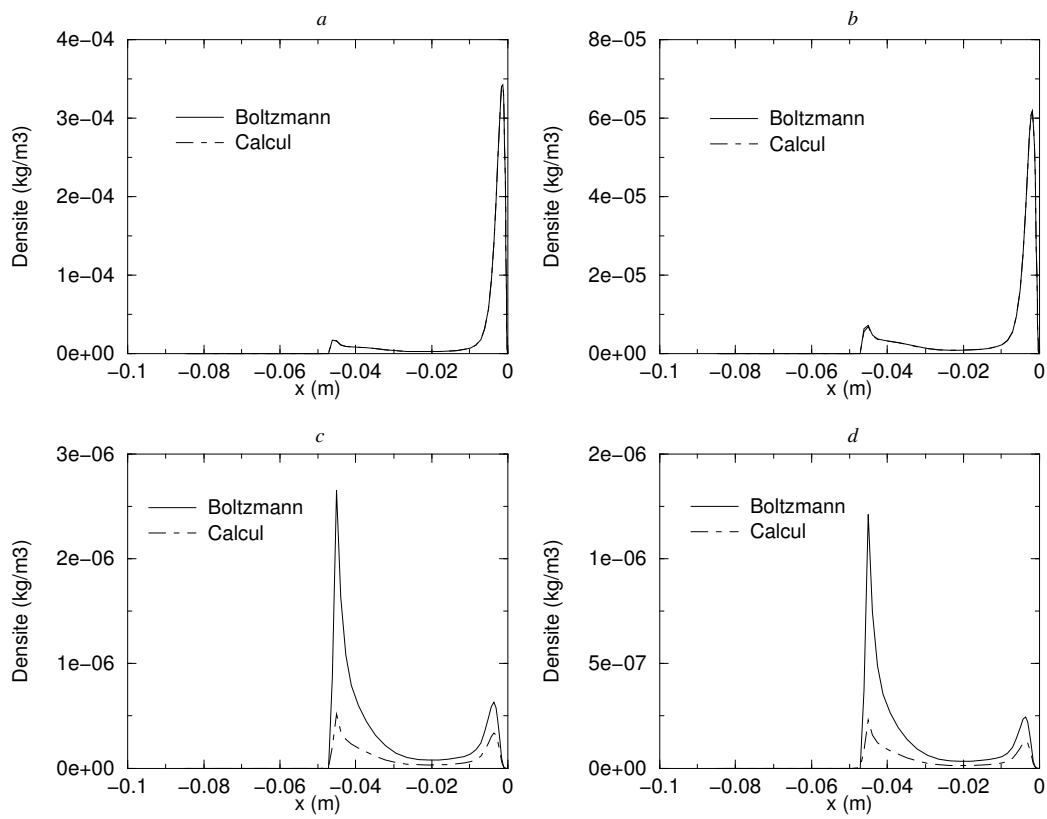
Figure 5.7. Densité des niveaux d'énergie (niveaux métastables en a et b, niveaux radiatifs en c et d) : comparaison entre l'équilibre de Boltzmann et le calcul hors équilibre (cas avec N^+ )
