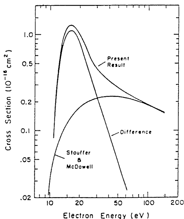
Figure 2.4. Section efficace totale interprétée comme la somme d'une composante représentant les processus d'excitation directe, et une composante représentant les processus d'excitation par cascade : travaux de Stone et al. [17]
