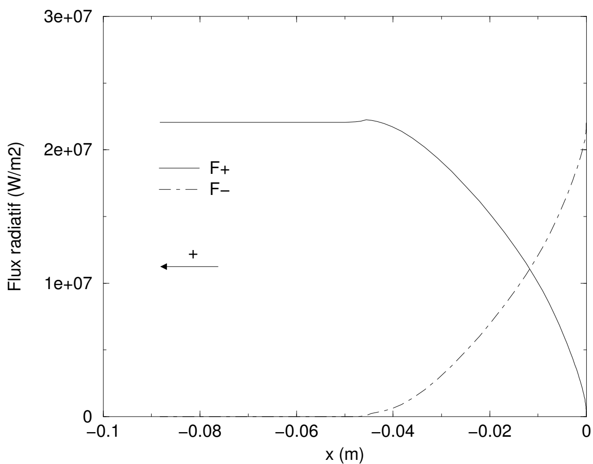
Figure 5.6. Calcul en déséquilibre thermo-chimique avec rayonnement : Flux radiatifs (contribution des raies atomiques et du continuum) le long de la ligne d'arrêt (cas avec N^+ ) avec paroi totalement absorbante
