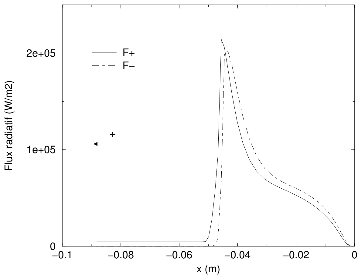
Figure 5.5. Calcul en déséquilibre thermo-chimique avec rayonnement : Flux radiatifs (contribution des raies atomiques) le long de la ligne d'arrêt (cas avec N^+ ) avec paroi totalement réfléchissante
