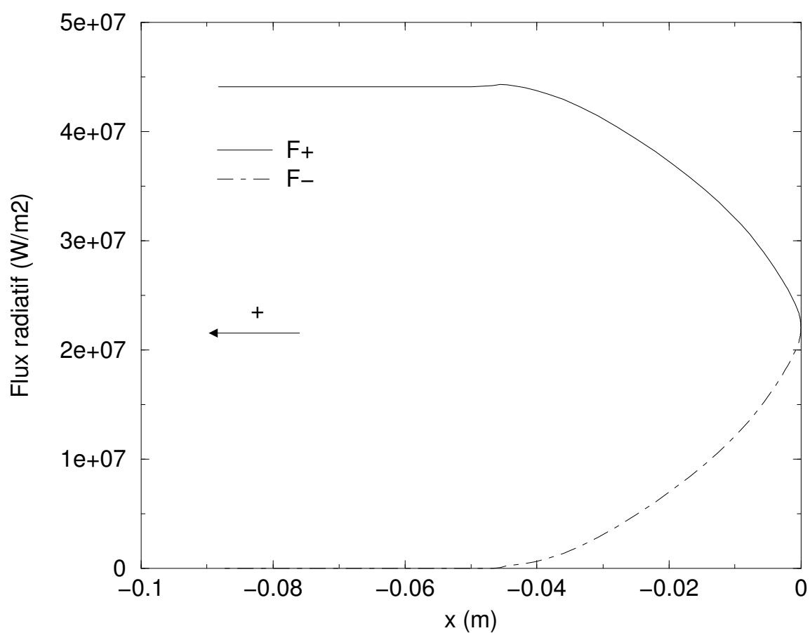
Figure 5.4. Calcul en déséquilibre thermo-chimique avec rayonnement : Flux radiatifs (contribution des raies atomiques et du continuum) le long de la ligne d'arrêt (cas avec N^+ ) avec paroi totalement réfléchissante
