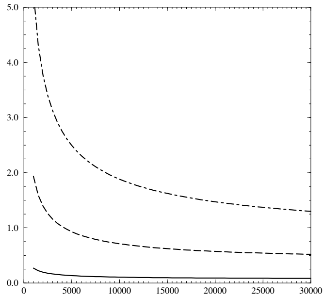
Figure 2.13. Taux de recombinaison radiative pour le carbone ( 10^{-19}m^3s^{-1} ) en fonction de la température électronique (K). Les transitions sont C(3P) - C^+(2P) (ligne continue épaisse), C(1D) - C^+(2P) (tirets longs) et C(1S) - C^+(2P) (tirets-pointillés)
