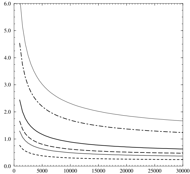
Figure 2.12. Taux de recombinaison radiative pour l'azote ( 10^{-19}m^3s^{-1} ) en fonction de la température électronique ( K ). Les transitions sont N(4S) - N^+(3P) (ligne continue épaisse), N(2D) - N^+(3P) (tirets longs), N(2D) - N^+(1D) (tirets-pointillés), N(2P) - N^+(3P) (tirets), N(2P) - N^+(1D) (pointillés) et N(2P) - N^+(1S) (ligne continue fine)
