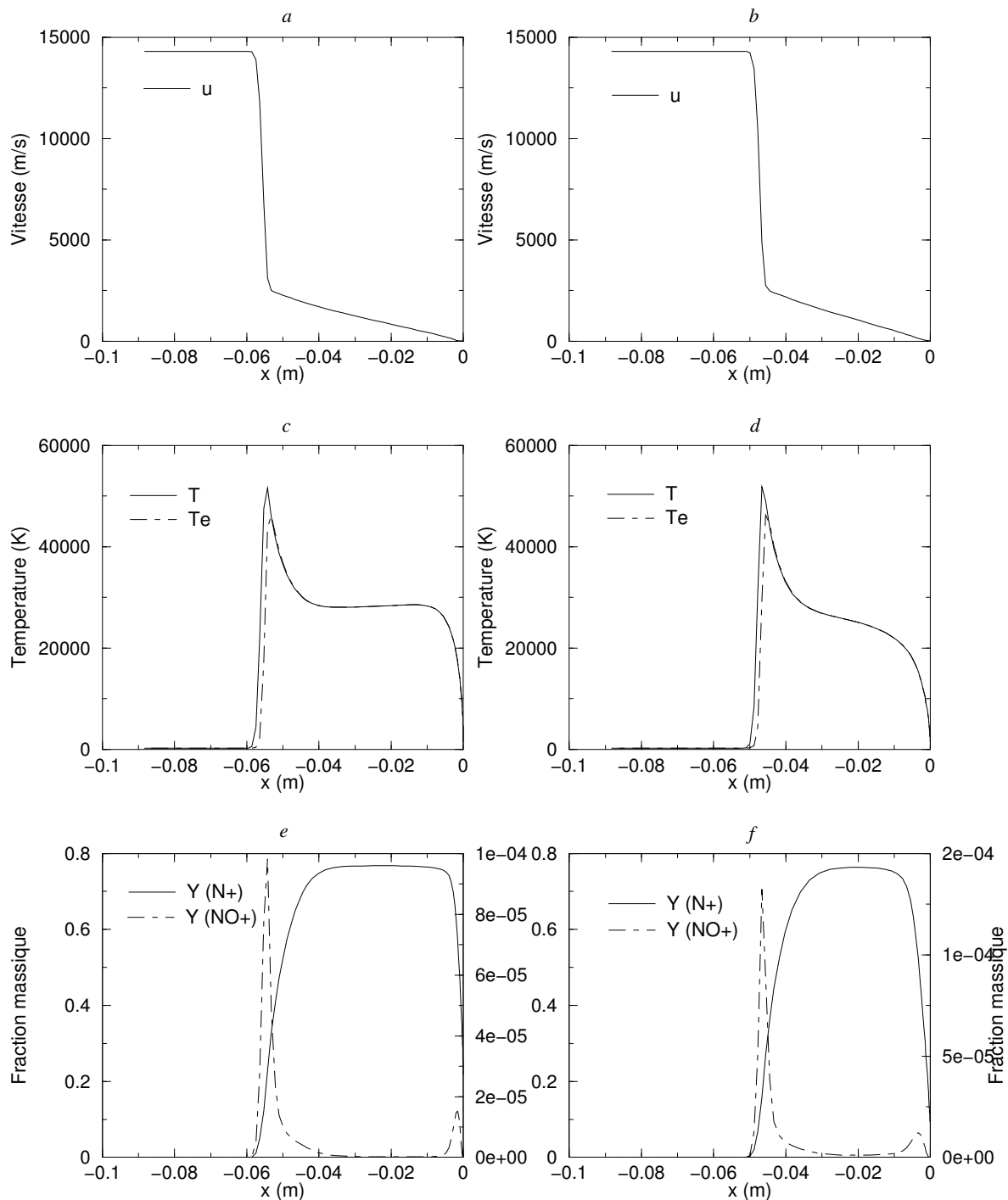
Figure 5.2. Calcul en déséquilibre thermo-chimique sans rayonnement (figures a,c,e ) et avec rayonnement avec paroi totalement réfléchissante (figures b,d,f ) : Profils de vitesse ( a,b ), de température ( c,d ), de fraction massique ( e,f ) le long de la ligne d'arrêt (cas avec N^+ )
