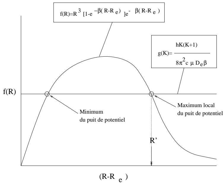
Figure F.1. Représentation des fonctions f(R) et g(K)
