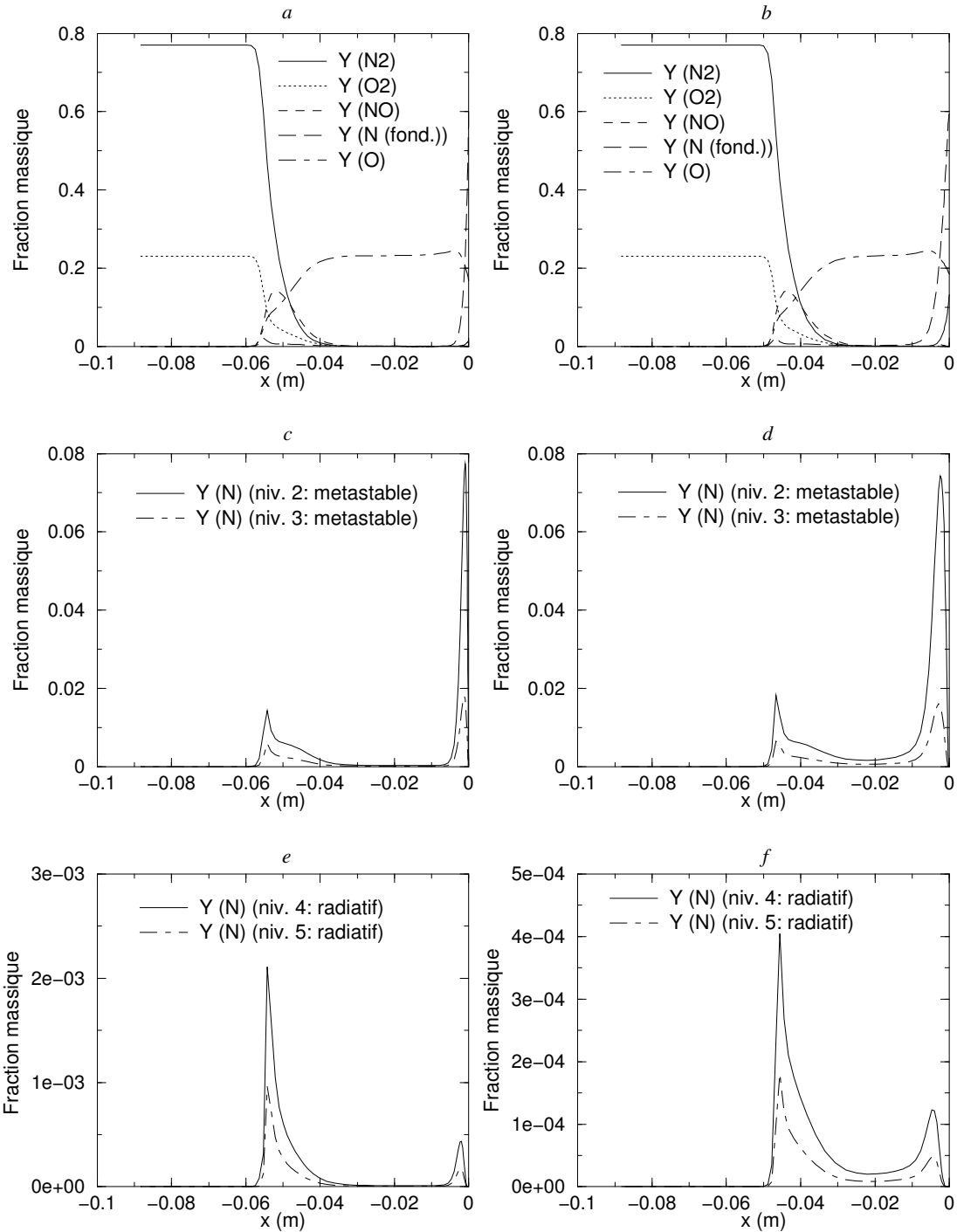
Figure 5.3. Calcul en déséquilibre thermo-chimique sans rayonnement (figures a,c,e ) et avec rayonnement avec paroi totalement réfléchissante (figures b,d,f ) : Profils de fraction massique ( a,b,c,d,e,f ) le long de la ligne d'arrêt (cas avec N^+ )
