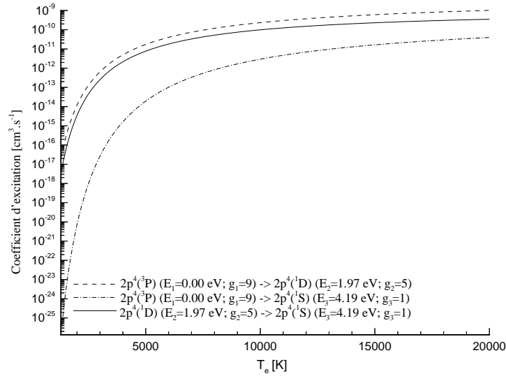
Figure 2.9. Coefficients d'excitation des états métastables par impact électronique en fonction de la température des électrons pour l'atome d'oxygène
