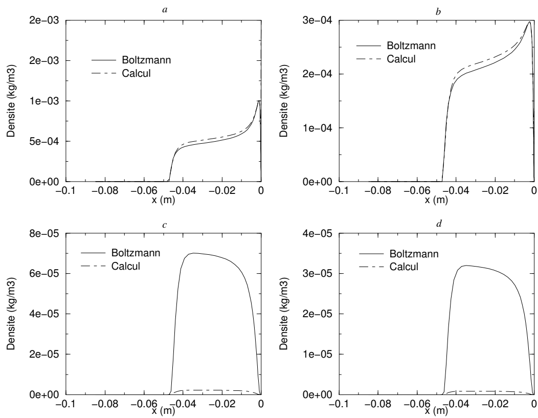
Figure 5.11. Densité des niveaux d'énergie (niveaux métastables en a et b, niveaux radiatifs en c et d) : comparaison entre l'équilibre de Boltzmann et le calcul hors équilibre (cas avec N_2^+ )
