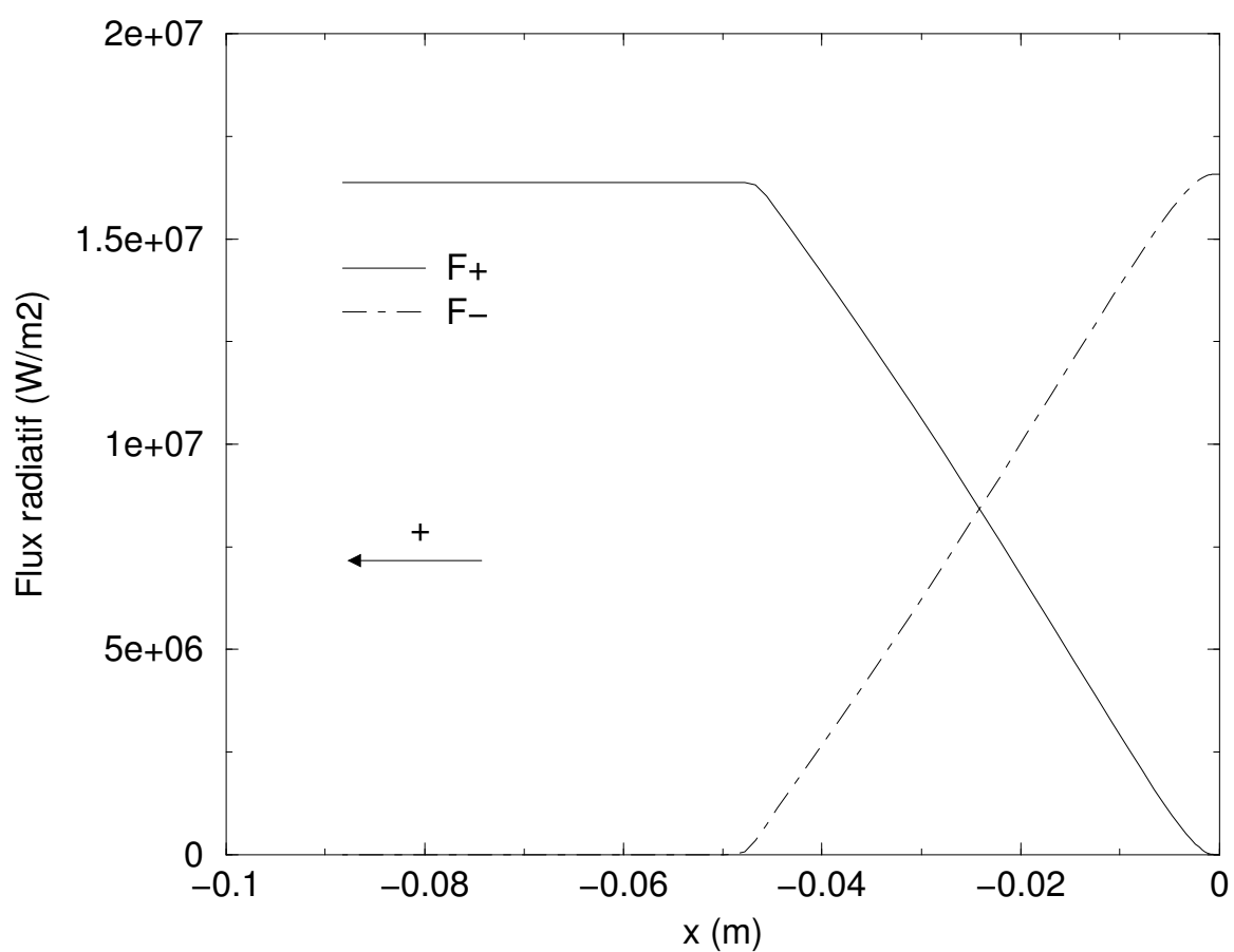
Figure 5.10. Calcul en déséquilibre thermo-chimique avec rayonnement : Flux radiatifs (contribution des raies atomiques et du continuum) le long de la ligne d'arrêt (cas avec N_2^+ )
