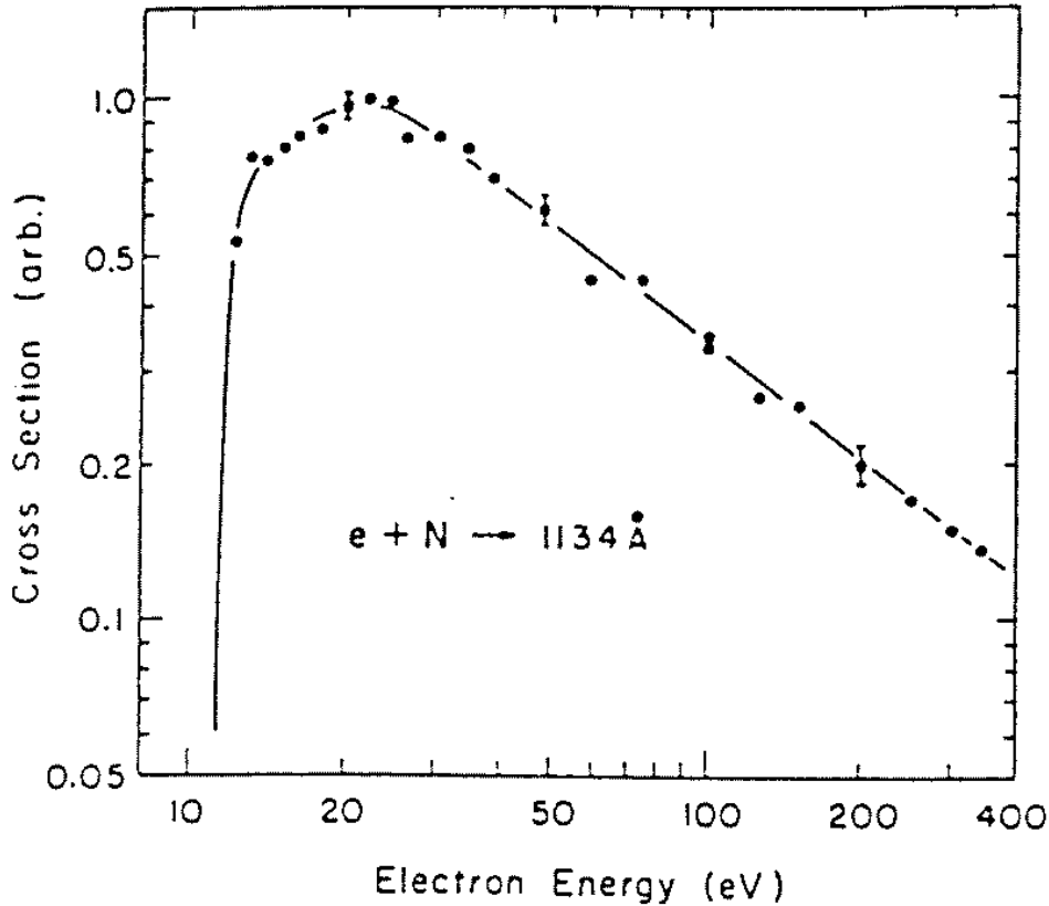
Figure 2.2. Section efficace d'excitation électronique par impact d'électron pour la transition N(2s^2 2p^3 (^4S^0)) \rightarrow N(2s 2p^4 (^4P)) : travaux de Stone et al. [15]
