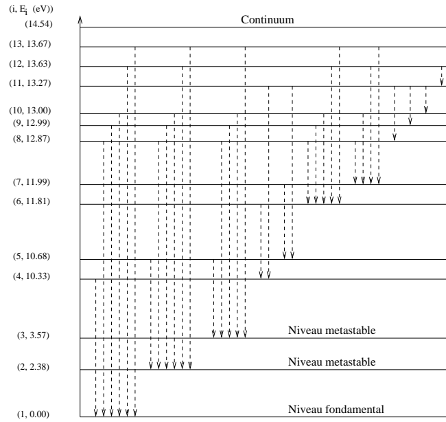
Figure 2.10. Premiers niveaux d'énergie de l'atome d'azote
