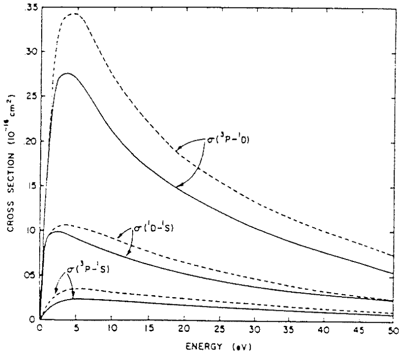
Figure 2.7. Variation de la section efficace inélastique avec l'énergie de l'électron incident pour l'atome d'oxygène : travaux de Henry et al. [28] (courbe solide) et Smith et al. [27] (courbe en pointillés)
