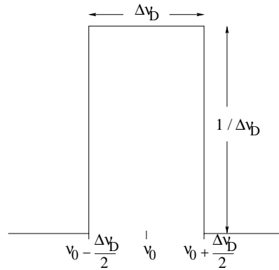
Figure 4.2. Profil de raie Doppler carré normalisé
