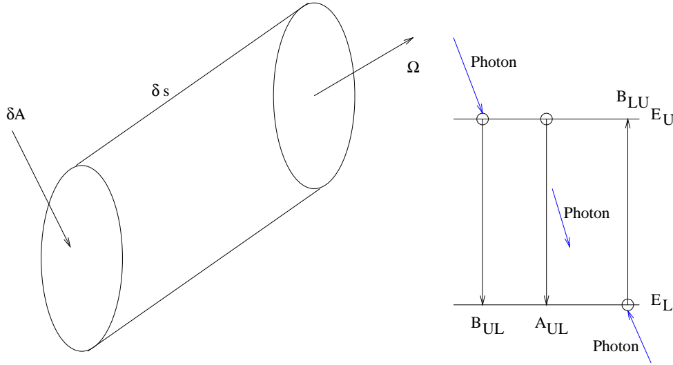
Figure 4.1. Elément de volume de direction \Omega
