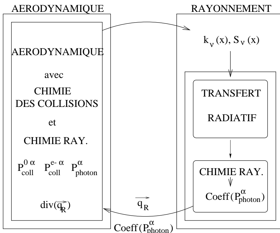
Figure 5.1. Algorithme de couplage
