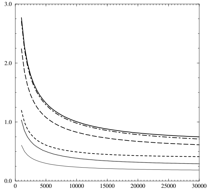
Figure 2.14. Taux de recombinaison radiative pour l'oxygène ( 10^{-19}m^3s^{-1} ) en fonction de la température électronique (K). Les transitions sont O(^3P) - O(^4S) (ligne continue épaisse), O(^3P) - O(^2D) (tirets longs), O(^3P) - O(^2P) (tirets-pointillés), O(^1D) - O(^2D) (tirets), O(^1D) - O(^2P) (pointillés) et O(^1S) - O(^2P) (ligne continue fine)
