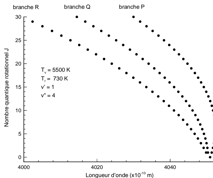
Figure 2.22. Diagramme de Fortrat pour la transition électronique 2^+ ( N_2(C^3\Pi_u) \longrightarrow N_2(B^3\Pi_g) )
