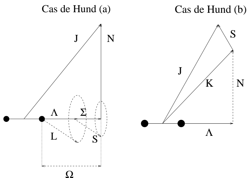
Figure F.3. Diagrammes des vecteurs pour les cas de Hund (a) et (b)
