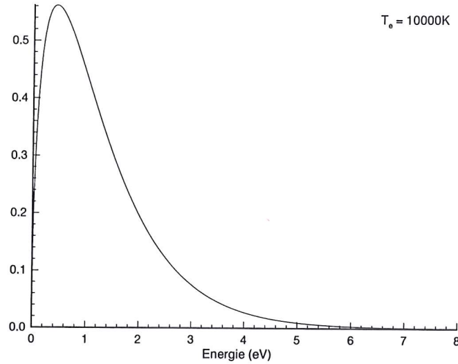
FIG. 2.1 – Maxwellienne des électrons à la température T_e = 10000K
