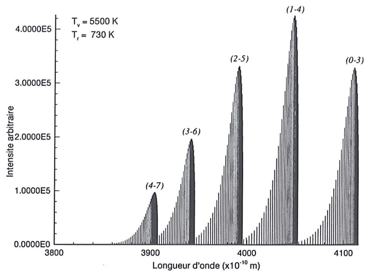
FIG. 2.19 – Transition électronique 2^+ ( N_2(C^3\Pi_u) \rightarrow N_2(B^3\Pi_g) ), branche P ( \Delta J = -1 )
