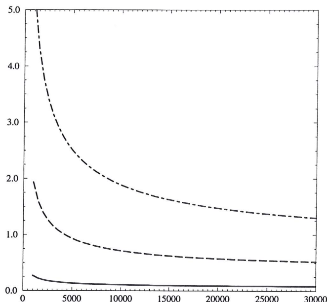
FIG. 2.13 – Taux de recombinaison radiative pour le carbone ( 10^{-19} m^3 s^{-1} ) en fonction de la température électronique ( K ). Les transitions sont C(3P) - C^+(2P) (ligne continue épaisse), C(1D) - C^+(2P) (tirets longs) et C(1S) - C^+(2P) (tirets-pointillés)
