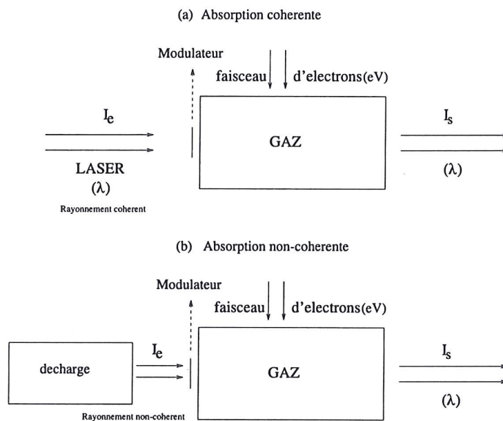
FIG. 2.5 – a) Absorption cohérente; b) Absorption non-cohérente
