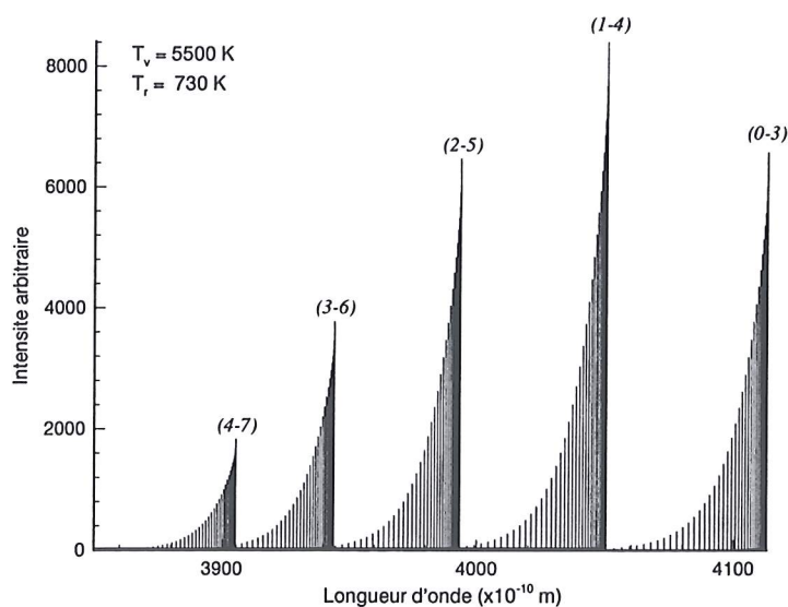
FIG. 2.20 – Transition électronique 2^+ ( N_2(C^3\Pi_u) \rightarrow N_2(B^3\Pi_g) ), branche Q ( \Delta J = 0 )
