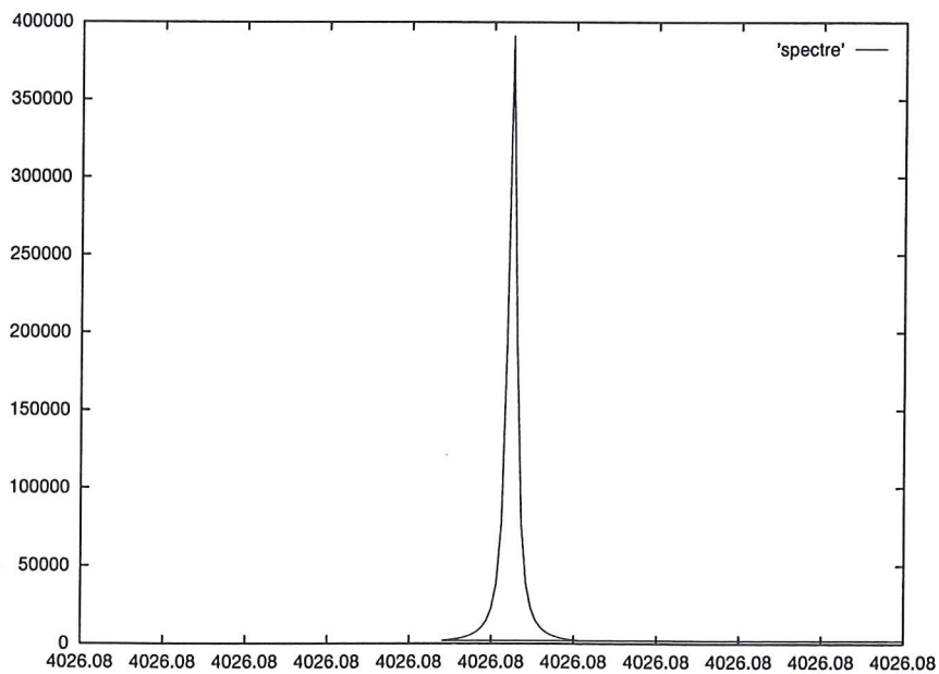
FIG. 2.18 – Détail d'une raie
