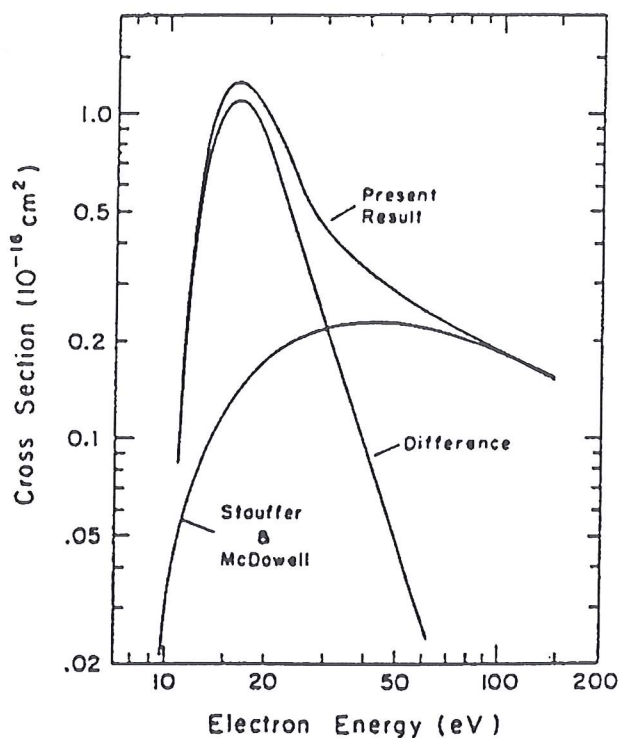
FIG. 2.4 – Section efficace totale interprétée comme la somme d'une composante représentant les processus d'excitation directe, et une composante représentant les processus d'excitation par cascade: travaux de Stone et al. [17]
