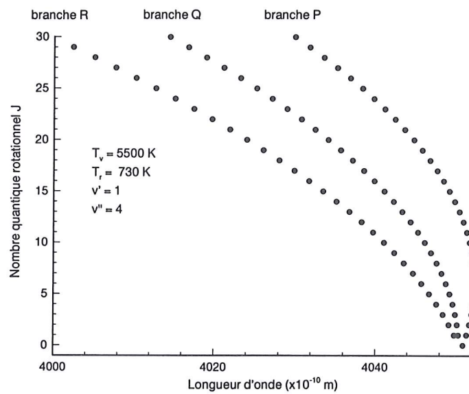
FIG. 2.22 – Diagramme de Fortrat pour la transition électronique 2^+ ( N_2(C^3\Pi_u) \longrightarrow N_2(B^3\Pi_g) )
