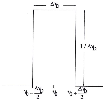
FIG. 4.2 – Profil de raie Doppler carré normalisé
