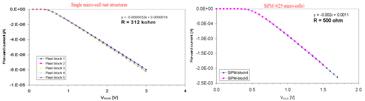
Graphique 4-19 : caractéristiques courant-tension des résistances seules et d'une matrice de photodiodes+résistance (SiPM) dans le sens passant d'ITC-irst (Italie).
