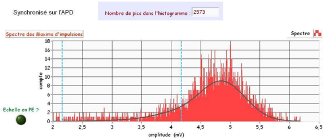
Graphique 4-24 : les variations de l'amplitude de l'impulsion Geiger dans le noir.
