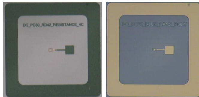
Figure 4-5 : deux photodiodes de 12µm et 30µm de côté, avec et sans résistance.
