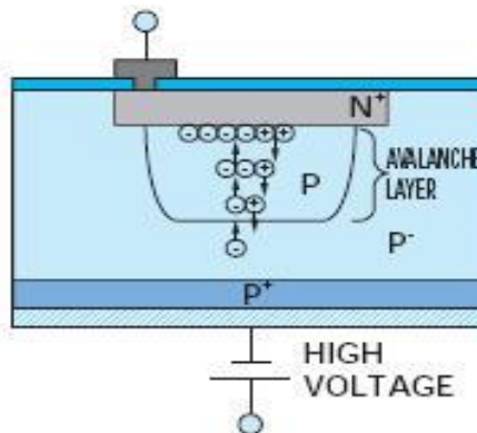
Figure 3-11 : la structure technologique présentée par Hamamatsu.
