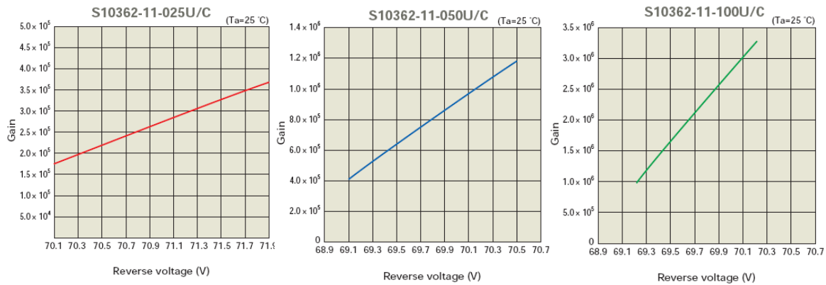
Graphique 4-35 : le gain expérimental des trois SiPM de Hamamatsu en fonction de la tension d'alimentation.
