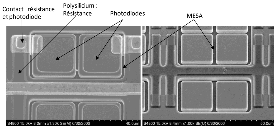
Figure 3-1 : le premier dispositif protégé par MESA.
