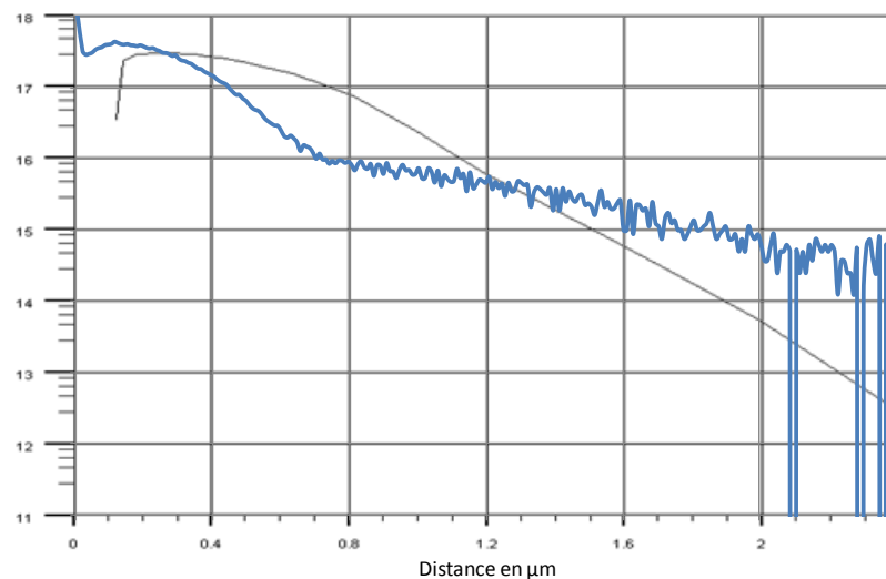
Graphique 3-9 : les deux profils de la zone P, simulé (en noir) et mesuré (en bleu).
