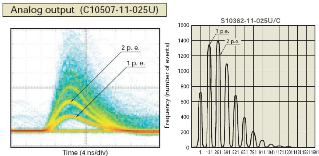
Graphique 4-36 : les courbes dynamiques temporelles en sortie du SiPM (à gauche) et la distribution des impulsions sur une charge de 50 ohms, avec 1 canal = 1mV (à droite) Vpol=71,0V.
