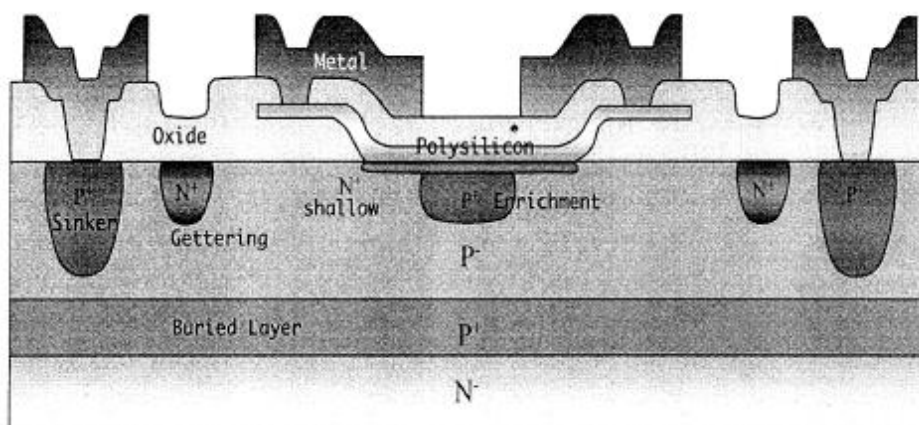
Figure 3-7 : la structure proposée par Sciacca avec une technologie compatible CMOS.
