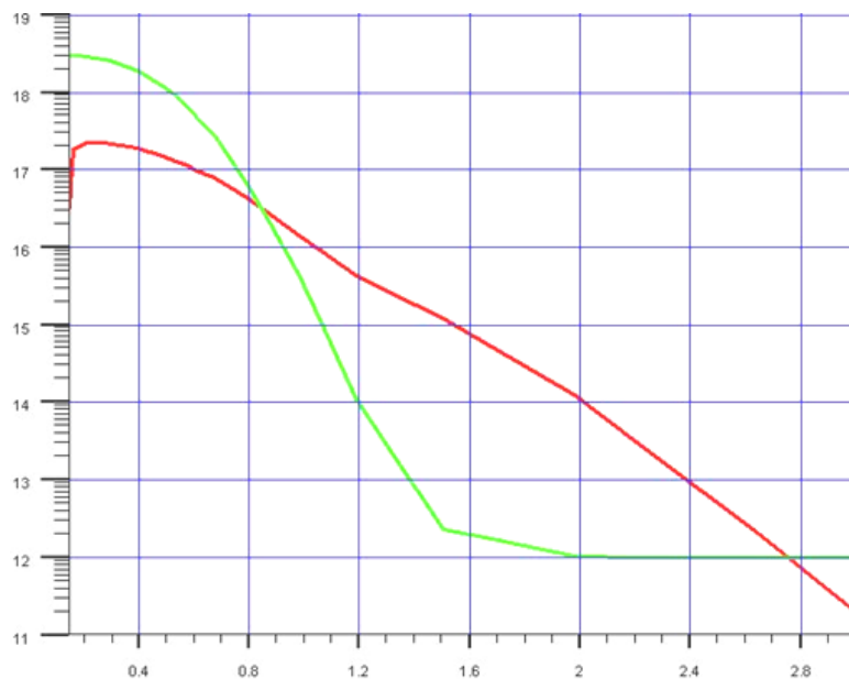
Graphique 3-5 : le profil de dopage de 4 couches constituant la diode à réaliser.
