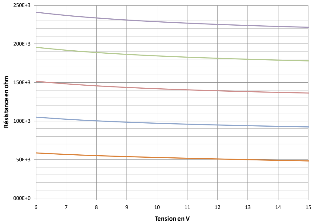
Graphique 4-7 : test des résistances ( \sim 50 kΩ/□) en polysilicium.
