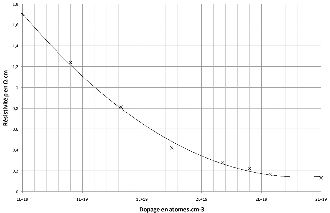
Graphique 4-8 : le modèle de la résistivité en fonction du dopage.
