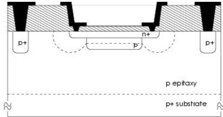
Figure 3-12 : la structure technologique proposée par SensL.
