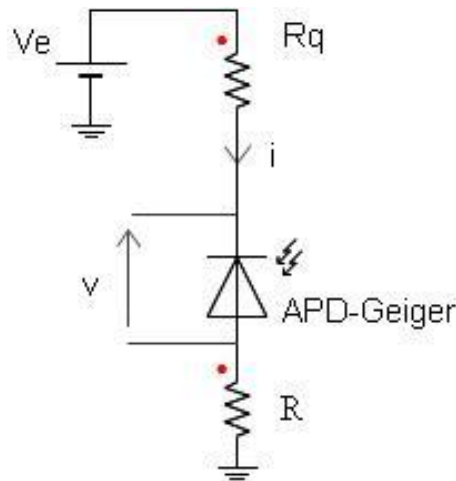
Figure 1-17 : le circuit électronique simple d'une APD-Geiger.
