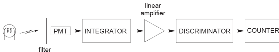
Figure 1-14 : la chaîne de détection et d'acquisition de signal.
